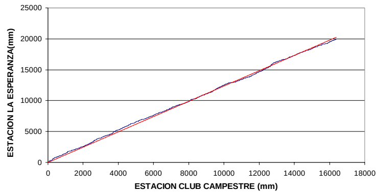
Figura 24. Curva de doble masa Esperanza contra CDMB.
