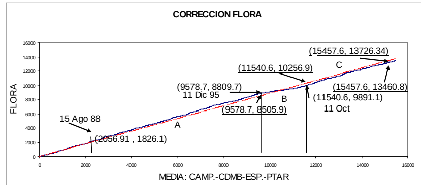
Figura 29. Corrección error sistemático para la estación la Flora.
