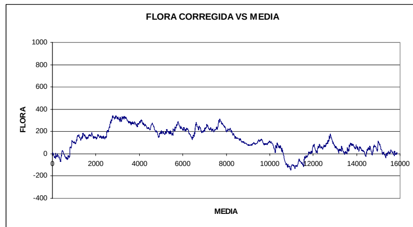
Figura 31. Curva del residuo para la estación La Flora corregida
