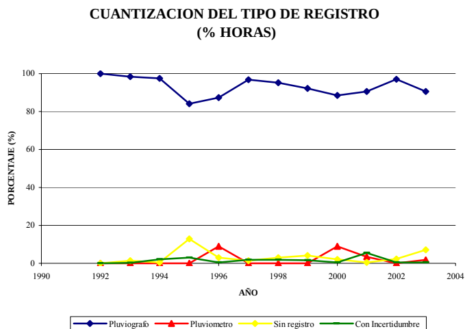
Figura 8. Porcentaje del registro del Pluviografo Ruitoque Alto.
