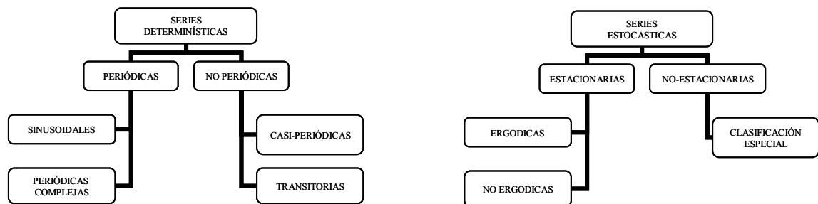
Figura 53. Clasificación de las series de tiempo según Vujica.
