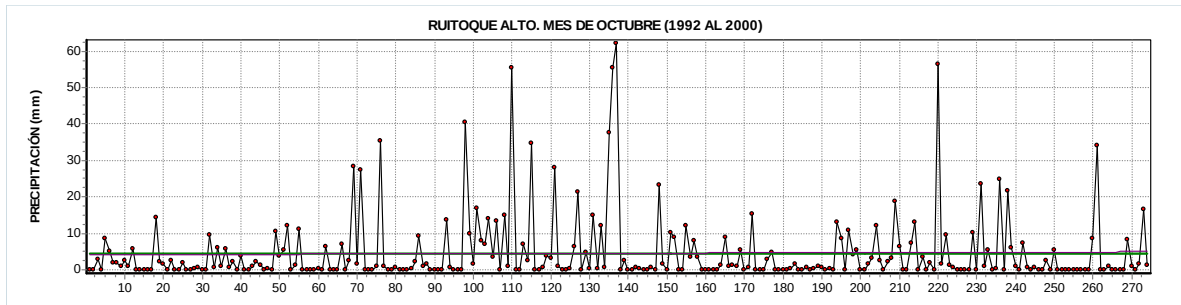
Figura 48. Valores diarios de precipitación para la estación Ruitoque Alto durante los meses de Octubre durante los años 1992 a 2000.
