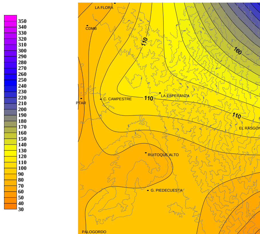
Figura 68. Distribución de la precipitación media en el mes de Junio.
