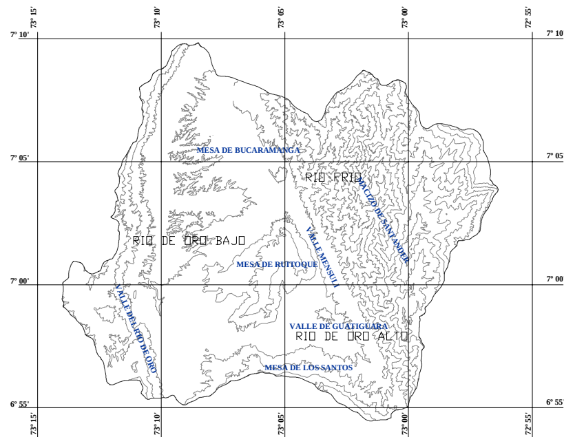
Figura 2. Cuenca del Río de Oro, curvas de nivel cada 50m.
