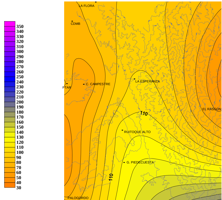
Figura 64. Distribución de la precipitación media del mes de Febrero.
