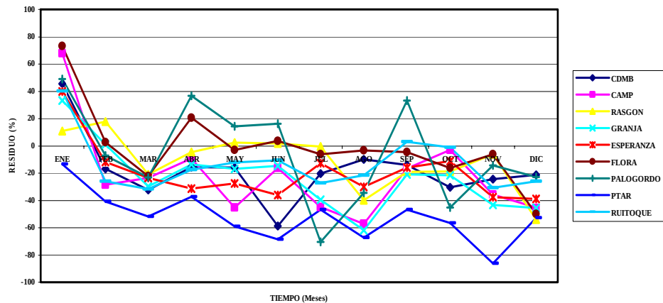
Figura 44. Valores residuales en porcentaje sobre el valor promedio del número de eventos de precipitación mensual del periodo de estudio para el año 1997.
