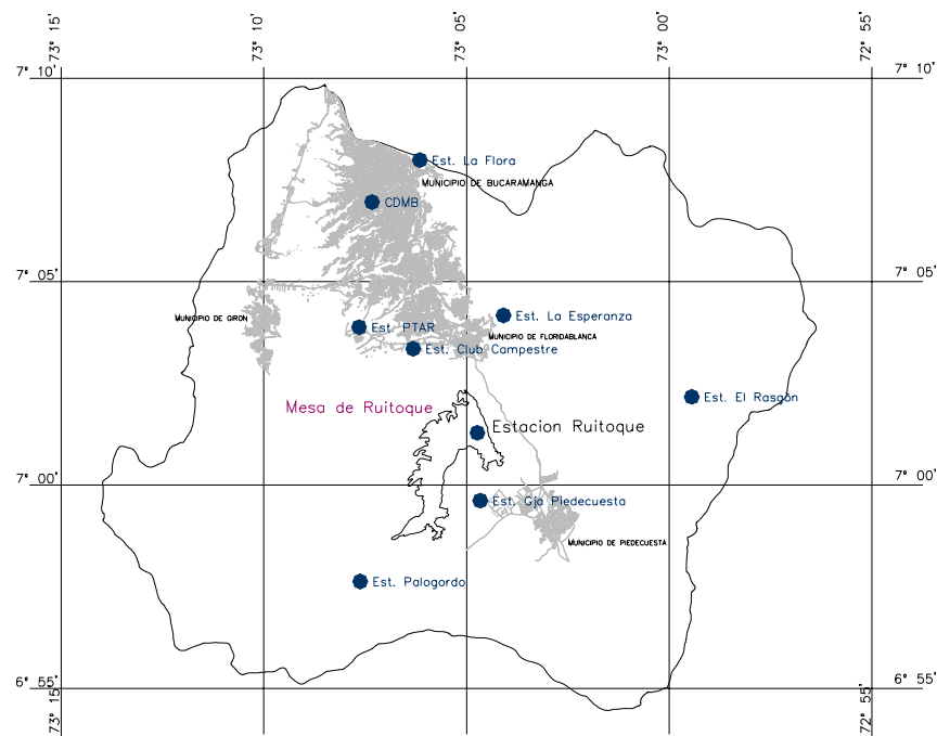
Figura 4. Inventario de estaciones de la CDMB y el IDEAM en la Cuenca del Río de Oro.
