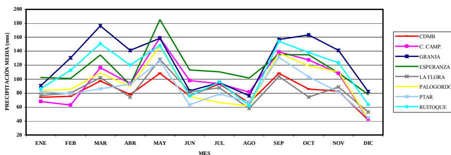
Figura 32. Valores mensuales multianuales promedio de precipitación para el periodo Julio de 1992 a Diciembre de 2000.
