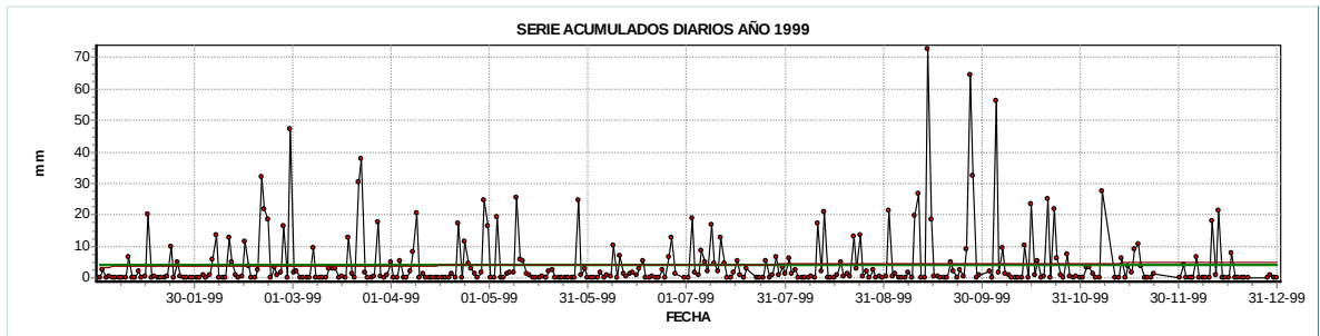
Figura 16. Serie de precipitación diaria para el año 1999.
