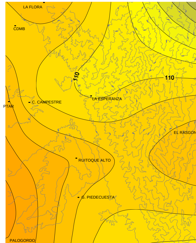
Figura 69. Distribución de la precipitación media en el mes de Julio.
