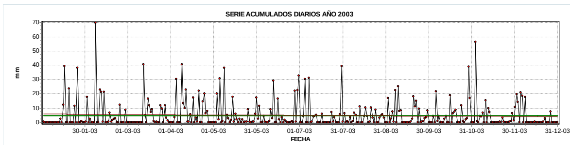
Figura 20. Serie de precipitación diaria para el año 2003.
