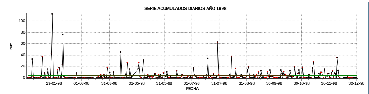
Figura 15. Serie de precipitación diaria para el año 1998.
