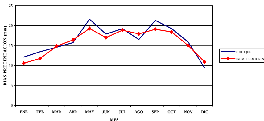
Figura 40. Número de eventos mensuales promedio de precipitación para el periodo Jul. de 1992 a Dic. de 2000 en la estación Ruitoque Alto.
