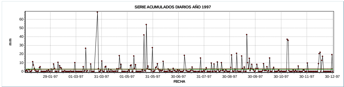
Figura 14. Serie de precipitación diaria para el año 1997.
