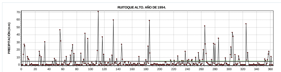
Figura 47. Valores diarios de precipitación para la estación Ruitoque Alto durante el año de 1994.
