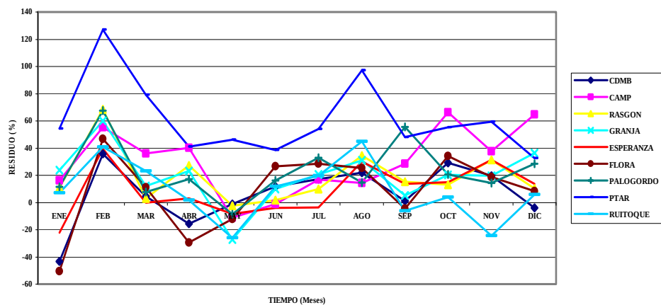
Figura 45. Valores residuales en porcentaje sobre el valor promedio del número de eventos de precipitación mensual del periodo de estudio para el año 1999.
