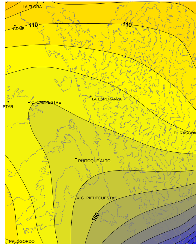
Figura 71. Distribución de la precipitación media en el mes d Septiembre.
