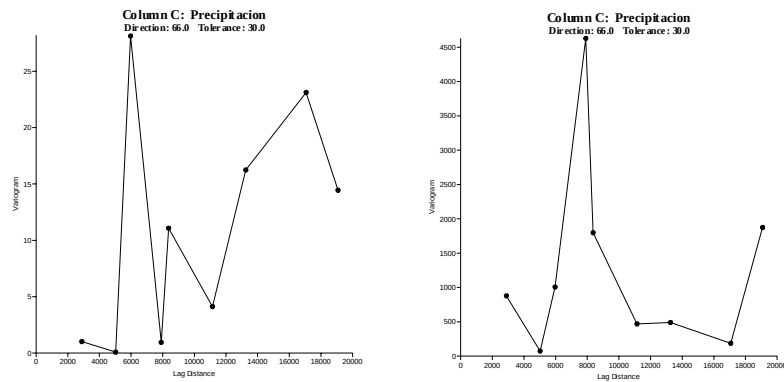
Figura 57. Ejemplo de iteración sobre los variogramas correspondientes a los días 21 de Julio de 1992 y 23 de Marzo de 2000.
