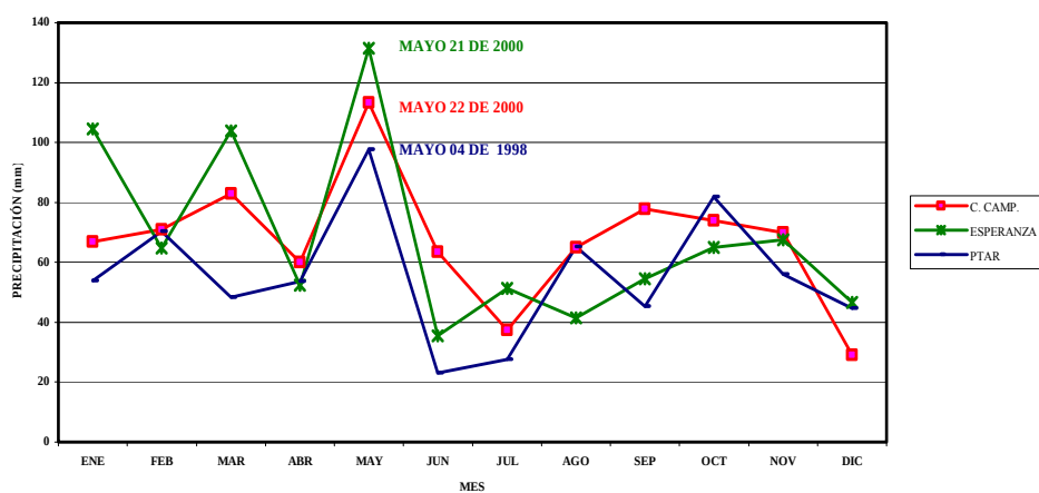
Figura 36. Ocurrencia del máximo evento histórico de precipitación para las estaciones Club Campestre, La Esperanza y PTAR, durante el periodo Jul. de 1992 a Dic. de 2000.
