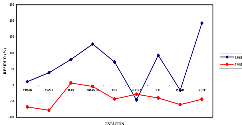
Figura 46. Valores residuales en porcentaje del total de precipitación durante los meses de Enero de 1998 y 1999.
