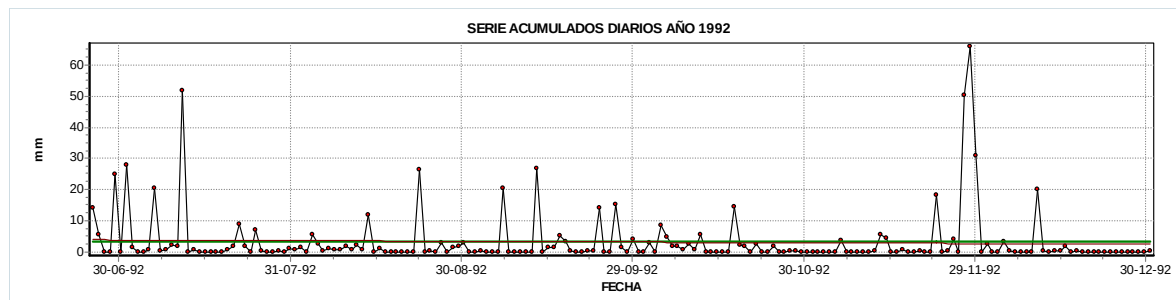
Figura 9. Serie de precipitación diaria para el año 1992.
