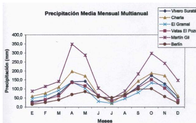
Figura 33. Precipitación media mensual multianual de la Cuenca superior del Río Lebrija.
