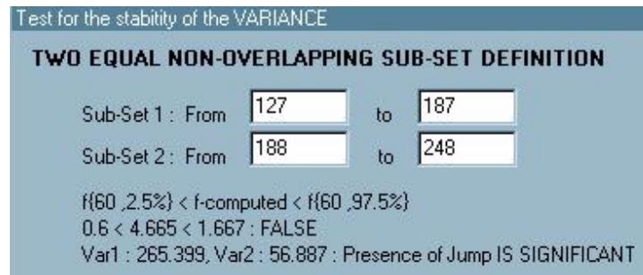
Figura 52. Resultado del programa SPELL-STAT para la prueba de estabilidad de varianza sobre la serie de los Eneros en la estación Ruitoque Alto.
