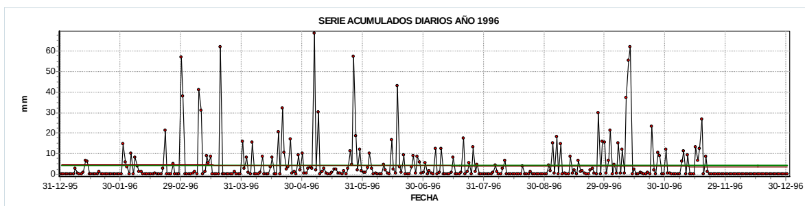
Figura 13. Serie de precipitación diaria para el año 1996.
