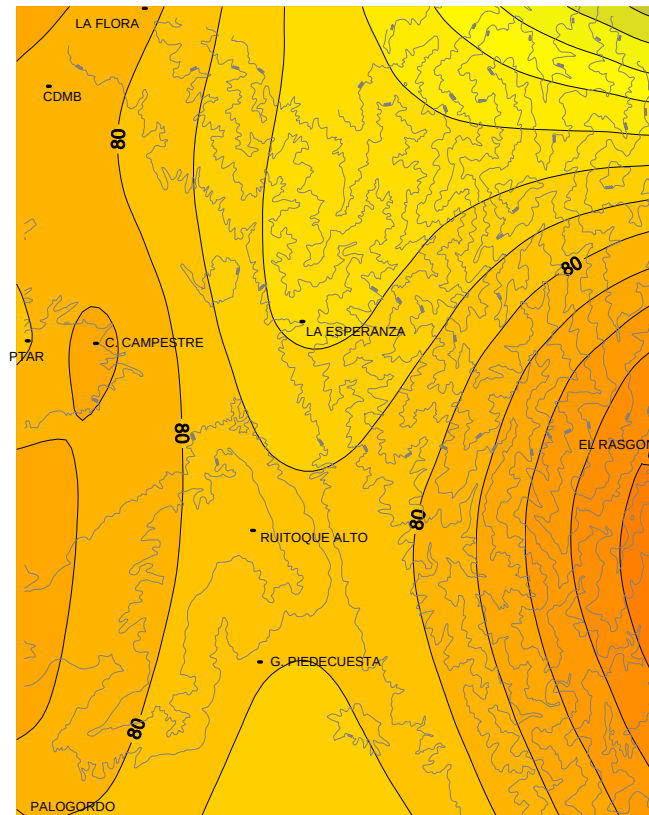
Figura 63. Distribución de la precipitación media del mes de Enero.
