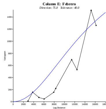
Figura 60. Modelamiento del variograma experimental correspondiente a los valores promedio mensuales para el mes de Febrero a partir del modelo cuadrático racional.
