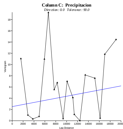
Figura 58. Variogramas experimental y modelado para el 21 de julio de 1992.
