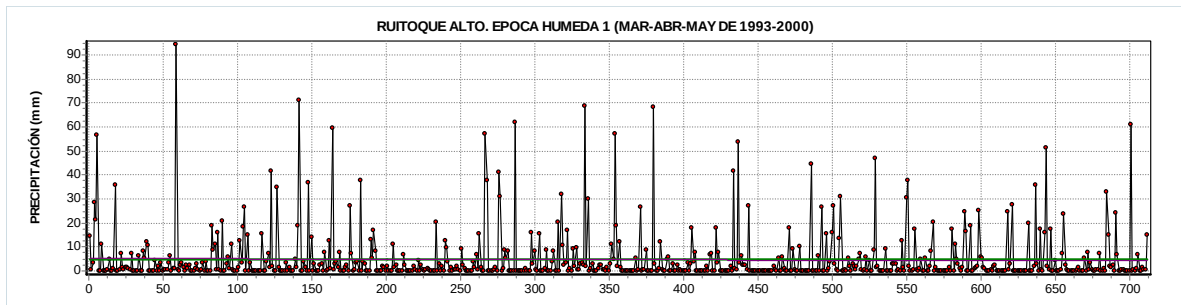
Figura 49. Valores diarios de precipitación para la estación Ruitoque Alto para la primera época húmeda del ciclo anual de los años 1993 al 2000.
