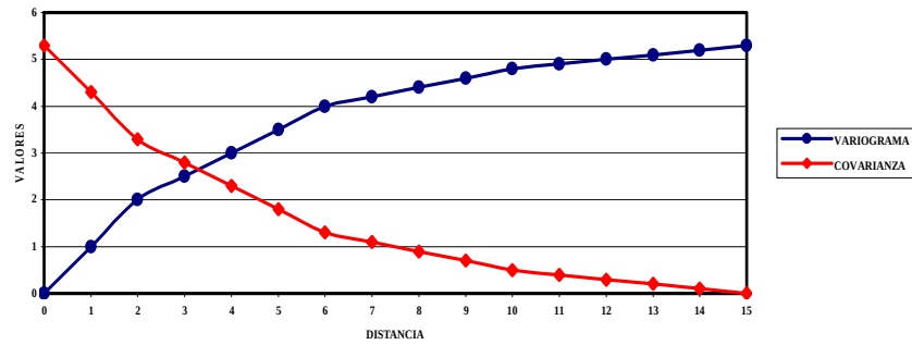
Figura 54. Relación entre el comportamiento del variograma y el comportamiento de la función de covarianza.
