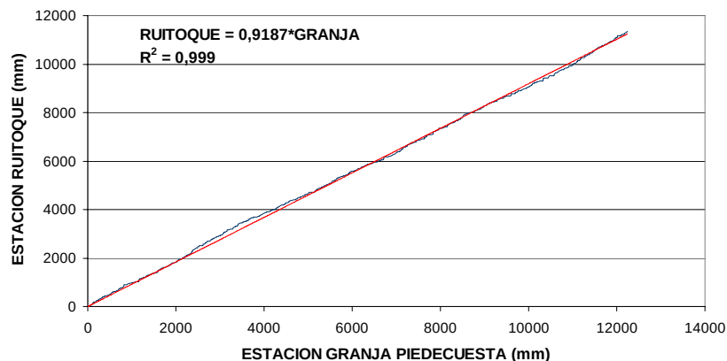
Figura 27. Curva de doble masa Granja Piedecuesta contra Ruitoque Alto.
