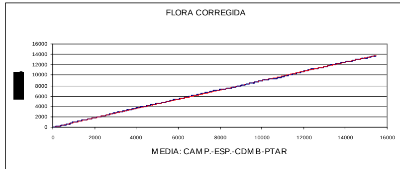
Figura 30. Curva de doble masa para la estación La Flora corregida.
