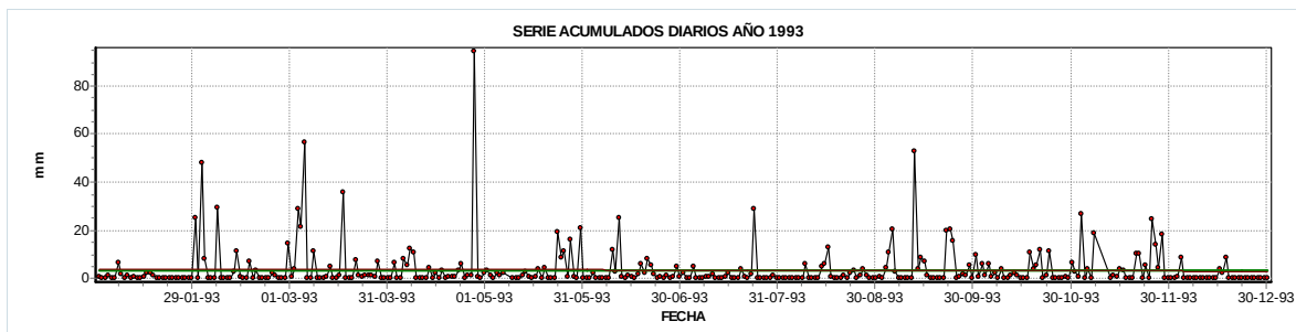
Figura 10. Serie de precipitación diaria para el año 1993.
