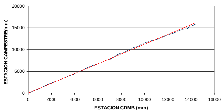
Figura 25. Curva de doble masa Campestre contra CDMB.
