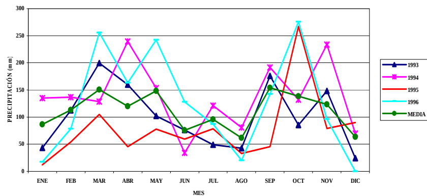
Figura 42. Variación de las series anuales de precipitación total mensual para la estación Ruitoque Alto, durante los años 1993 a 1996.
