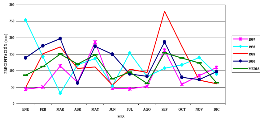
Figura 43. Variación de las series anuales de precipitación total mensual para la estación Ruitoque Alto, durante los años 1997 a 2000.
