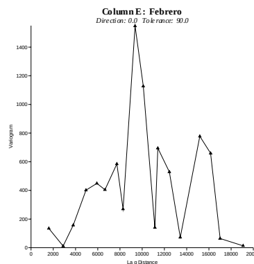
Figura 59. Variograma experimental para la serie de valores promedio mensuales del mes de Febrero.
