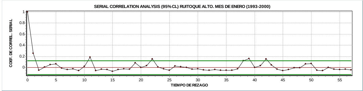
Figura 51. Correlograma de la serie de precipitación durante los meses de Enero de 1993 al 2000 para la estación Ruitoque Alto.
