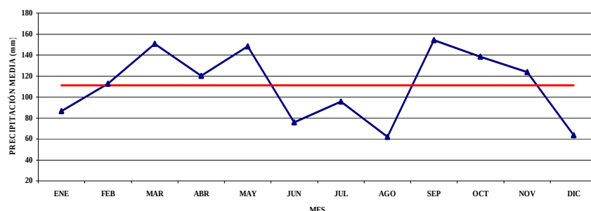
Figura 39. Valores mensuales multianuales promedio de precipitación para la estación Ruitoque Alto durante el periodo, Julio de 1992 a Diciembre de 2000.
