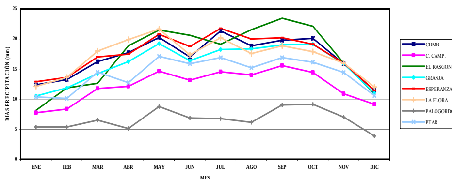
Figura 35. Número de eventos mensuales promedio para el periodo Jul. de 1992 a Dic. de 2000.
