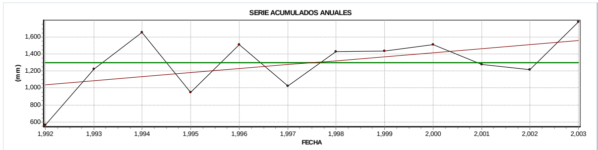
Figura 22. Serie de acumulados anuales para el periodo de 1992 al 2003.
