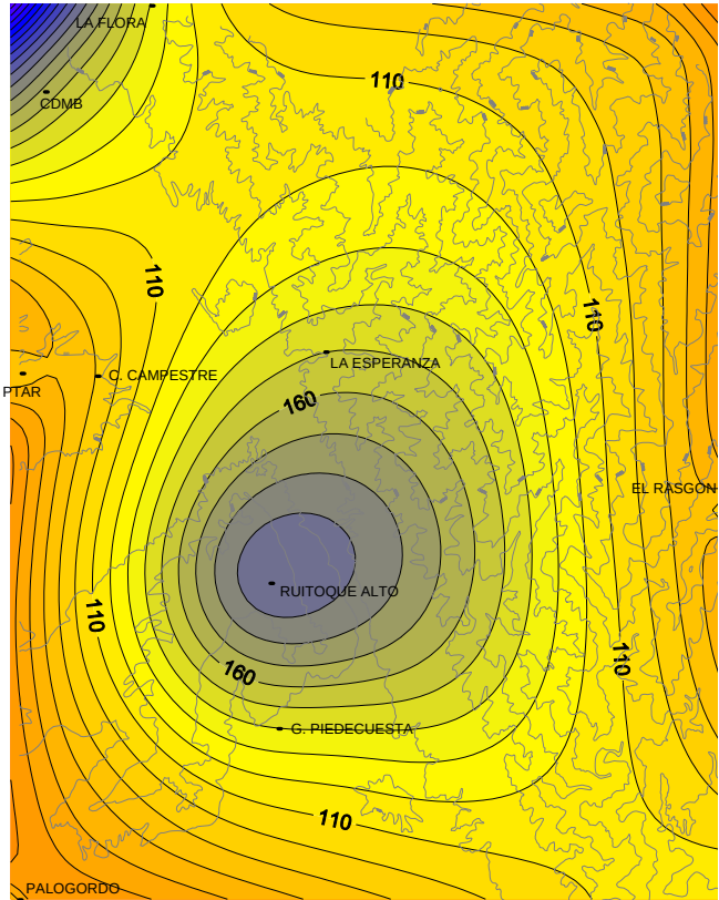
Figura 65. Distribución de la precipitación media en el mes de Marzo.
