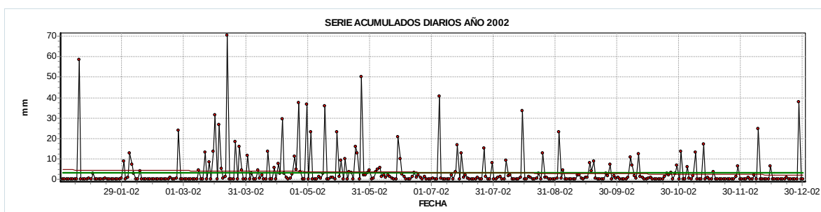
Figura 19. Serie de precipitación diaria para el año 2002.
