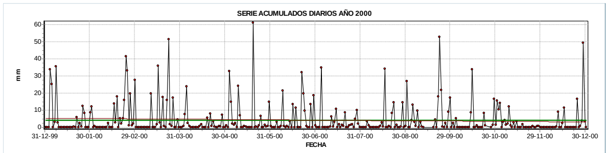
Figura 17. Serie de precipitación diaria para el año 2000.
