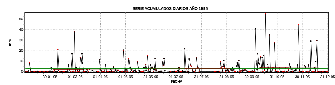
Figura 12. Serie de precipitación diaria para el año 1995.
