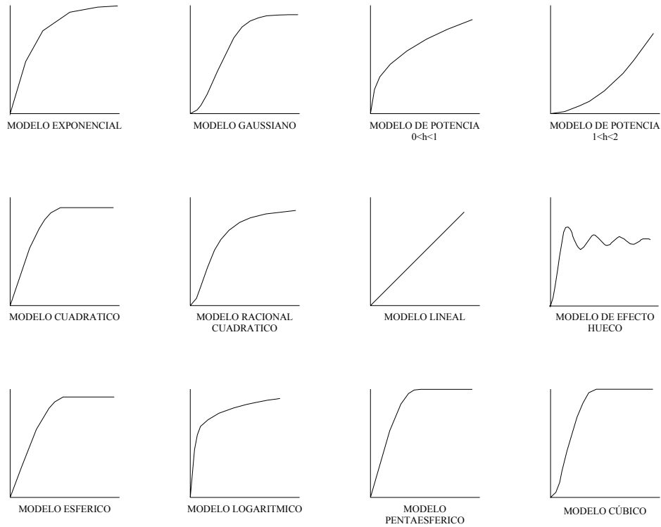
Figura 56. Modelos teóricos típicos de variograma.
