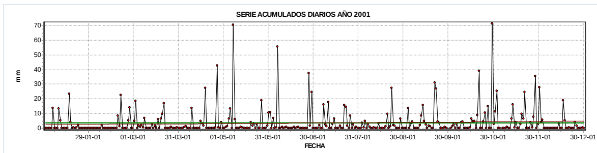
Figura 18. Serie de precipitación diaria para el año 2001.
