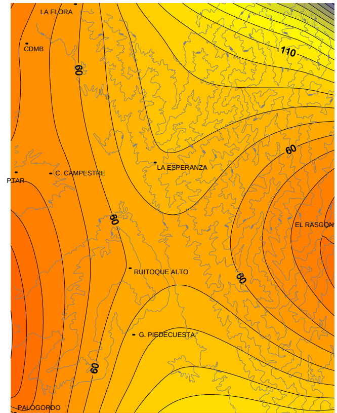
Figura 74. Distribución de la precipitación media en el mes de Diciembre.
