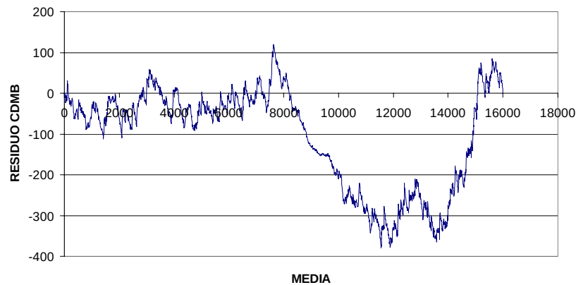
Figura 26. Curva de residuos acumulados para CDMB contra la media acumulada.
