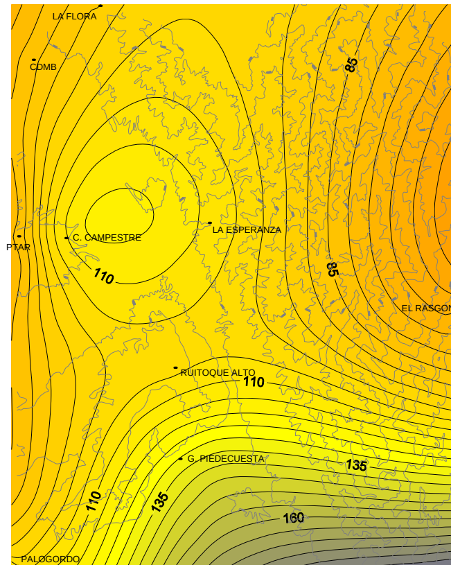
Figura 73. Distribución de la precipitación media en el mes de Noviembre.
