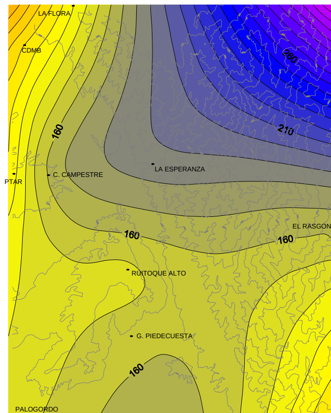
Figura 67. Distribución de la precipitación media en el mes de Mayo.
