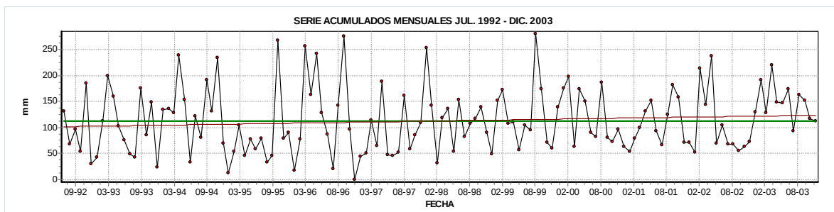
Figura 21. Serie de acumulados mensuales para el periodo Julio de 1992 a Diciembre de 2003.
