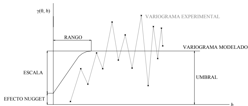
Figura 55. Parámetros que componen el variograma.
