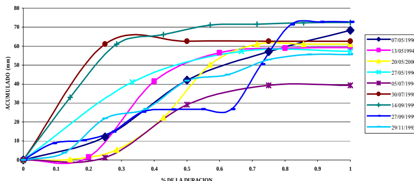
Figura 62. Curvas de porcentaje-masa para eventos inferiores a 80 mm en la estación Ruitoque Alto.
