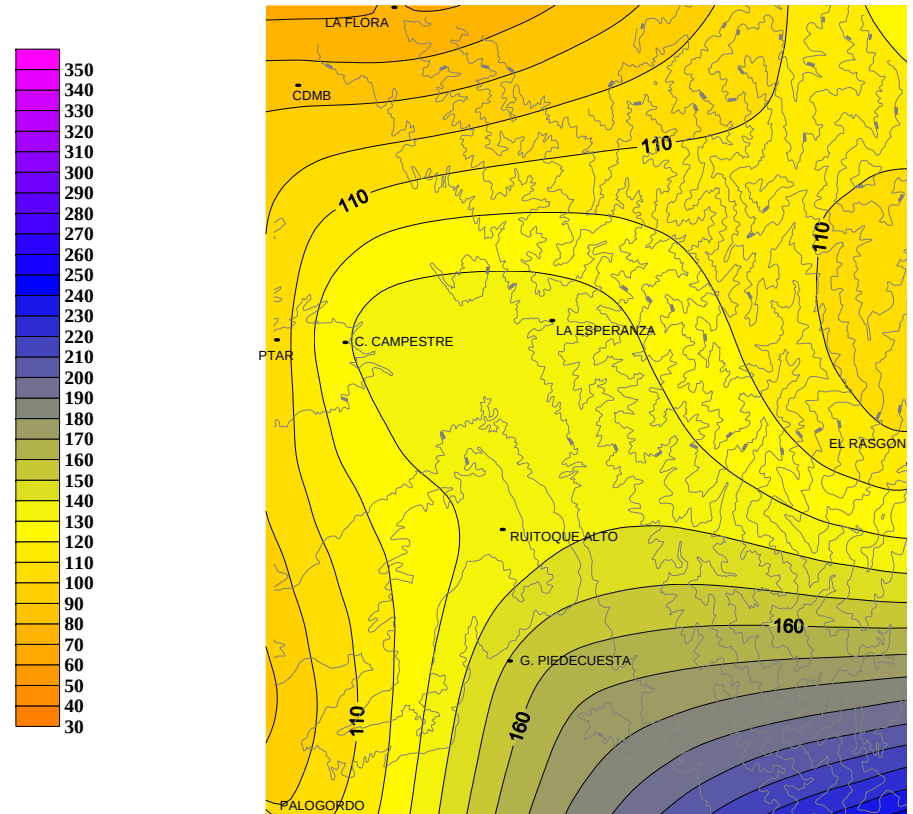
Figura 72. Distribución de la precipitación media en el mes de Octubre.
