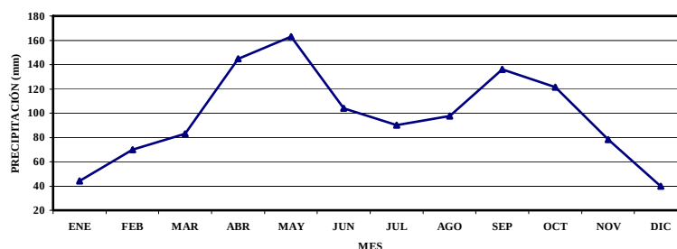
Figura 34. Valores mensuales multianuales promedio de precipitación para la estación El Rasgón durante el periodo, Julio de 1992 a Diciembre de 2000.
