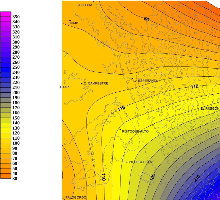
Figura 66. Distribución de la precipitación media en el mes de Abril.
