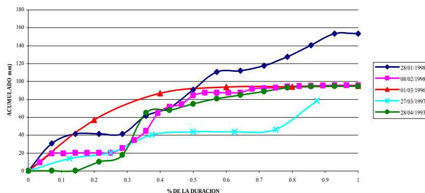
Figura 61. Curvas de porcentaje-masa para eventos superiores a 80 mm en la estación Ruitoque Alto.
