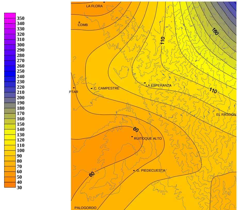
Figura 70. Distribución de la precipitación media en el mes de Agosto.
