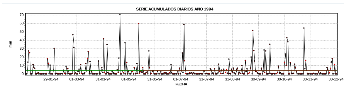
Figura 11. Serie de precipitación diaria para el año 1994.
