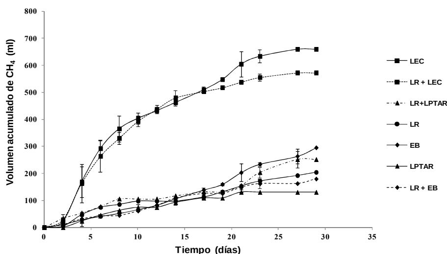
Figura 1.5 Volumen de metano acumulado (condiciones estándar de presión y temperatura) a partir del acetato usando los diferentes inóculos (pH: 7.0, T: 39±2 °C)
