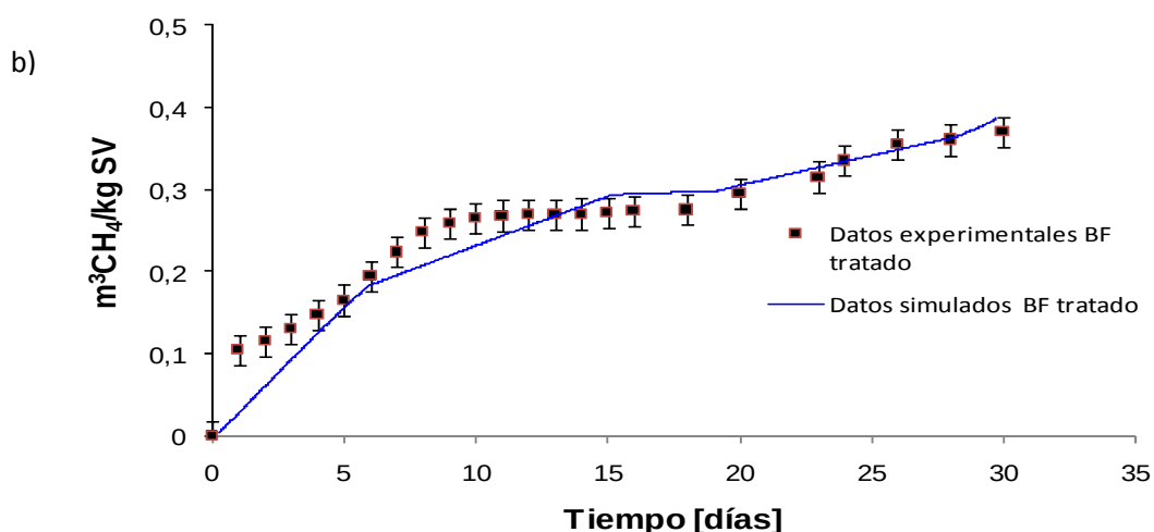
Figura 5.3 Perfiles de biodegradabilidad del bagazo de fique. a) PBM a partir de bagazo de fique en estado natural; b) PBM a partir de bagazo de fique tratado hidrotérmicamente.
