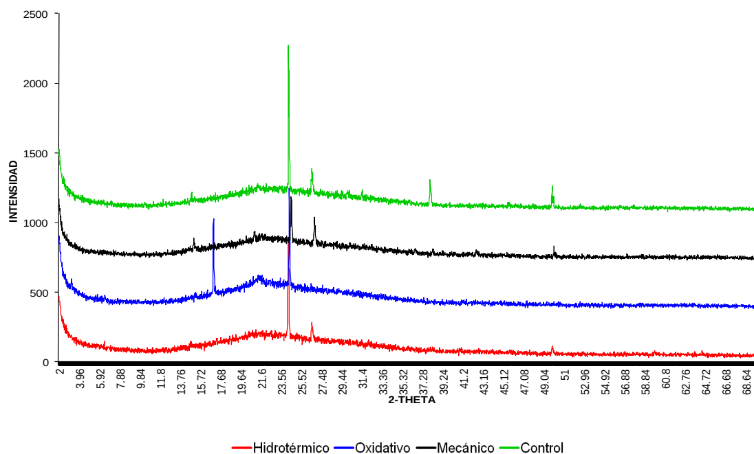
Figura 3.4 Difractograma rayos X del BF tratado y sin tratar
