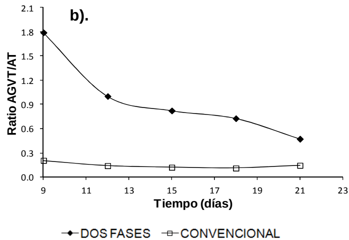
Figura 2.14 Evaluación de la estabilidad de los reactores fase B y convencional: a) pH ; b) Ratio AGV/AT
