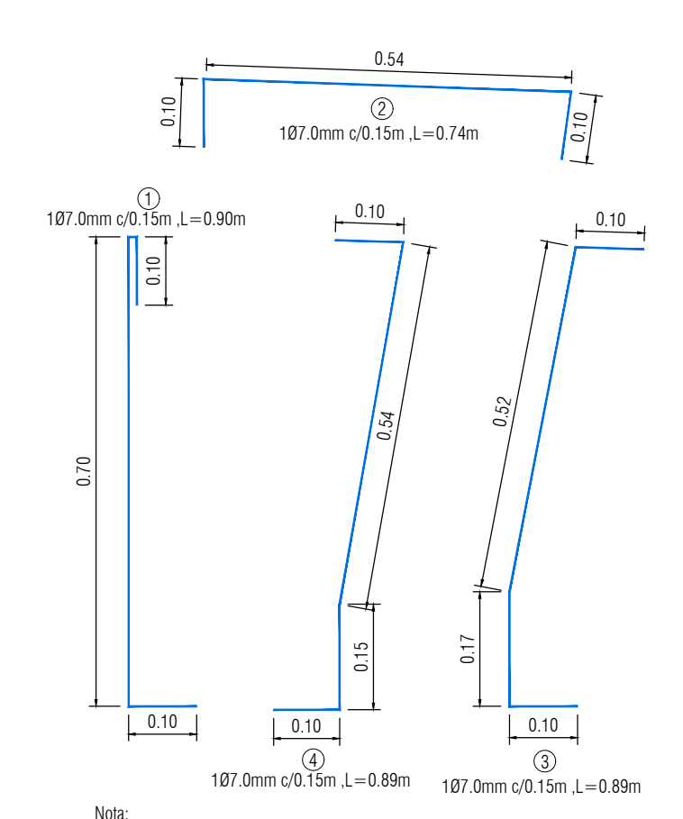
FIGURADO DE REFUERZO ESCALA 1:10
