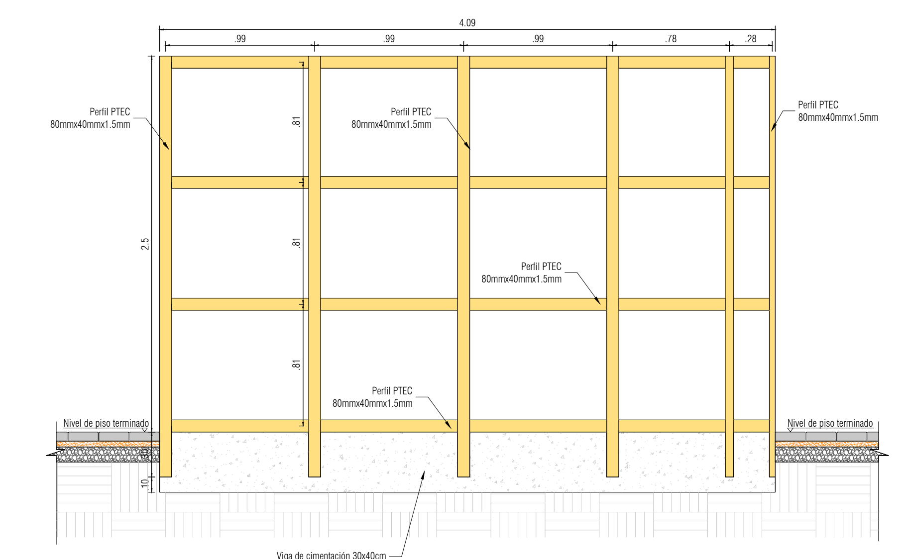
ESTRUCTURA PARA AULA EXTERIOR CORTE A-A ESCALA 1:25
