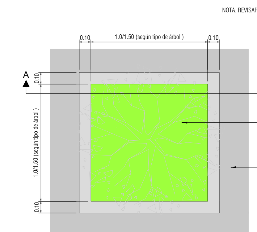
PLANTA ESCALA 1:20
