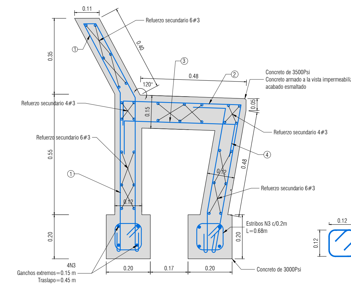
CORTE DE DETALLE DE BANCA CON ESPALDAR ESCALA 1:10
