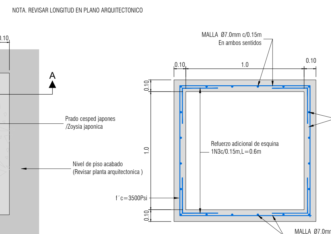
PLANTA ESCALA 1:20
