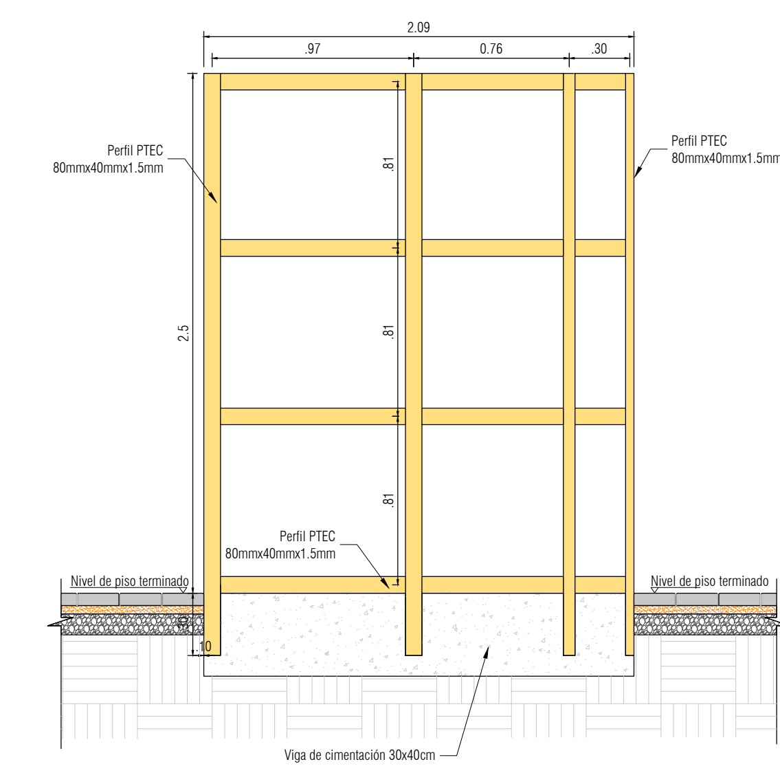
ESTRUCTURA PARA AULA EXTERIOR CORTE B-B ESCALA 1:25
