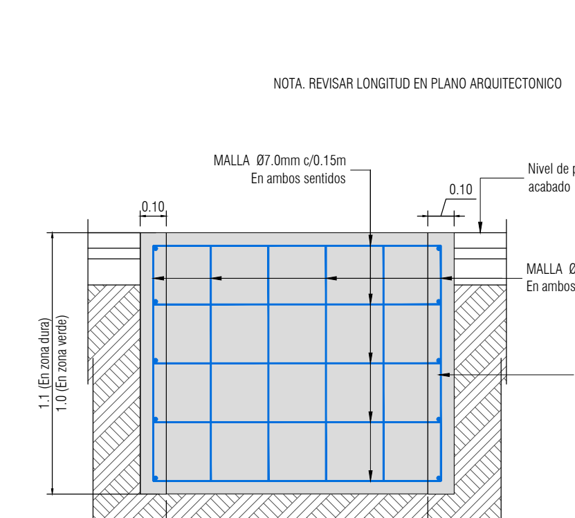
CORTE A-A CONTENEDOR DE RAÍCES CUADRADO-CIRCULAR ESCALA 1:20
