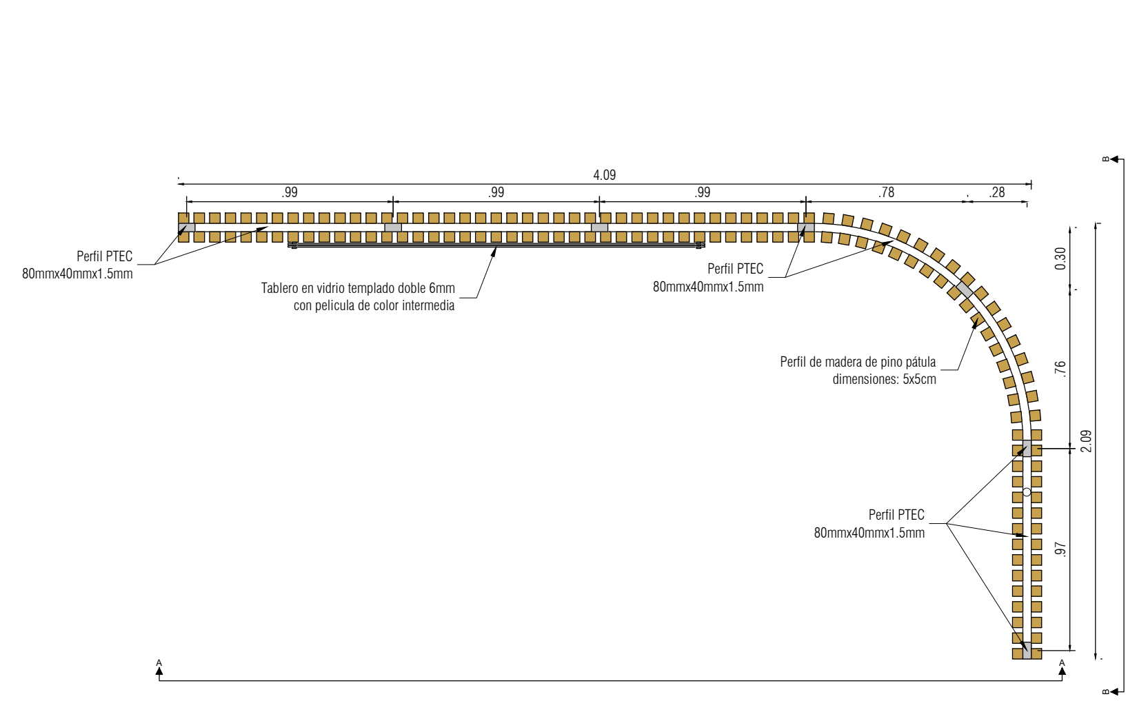
ESTRUCTURA PARA AULA EXTERIOR PLANTA ESCALA 1:25
