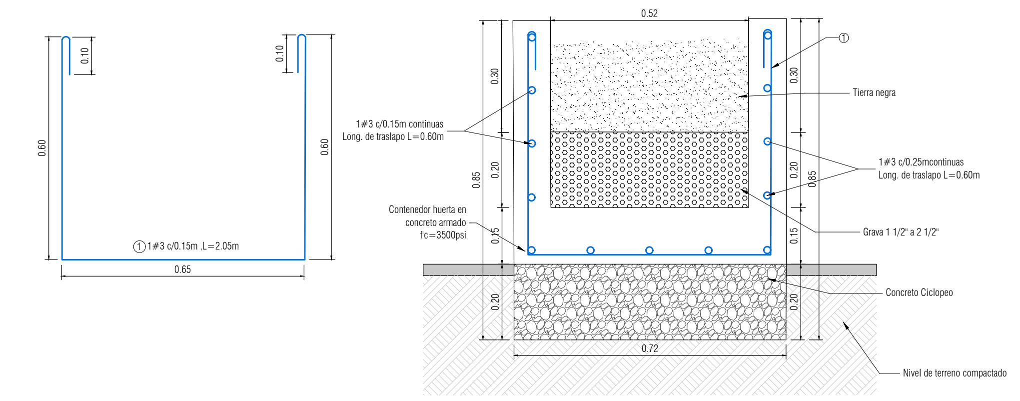
CONTENEDOR HUERTA DIMENSIONES Y REFUERZO ESCALA 1:10
