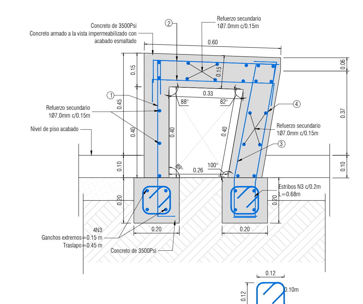
DETALLE DE BANCA CORRIDA SIN ESPALDAR DIMENSIONES Y REFUERZO ESCALA 1:10
