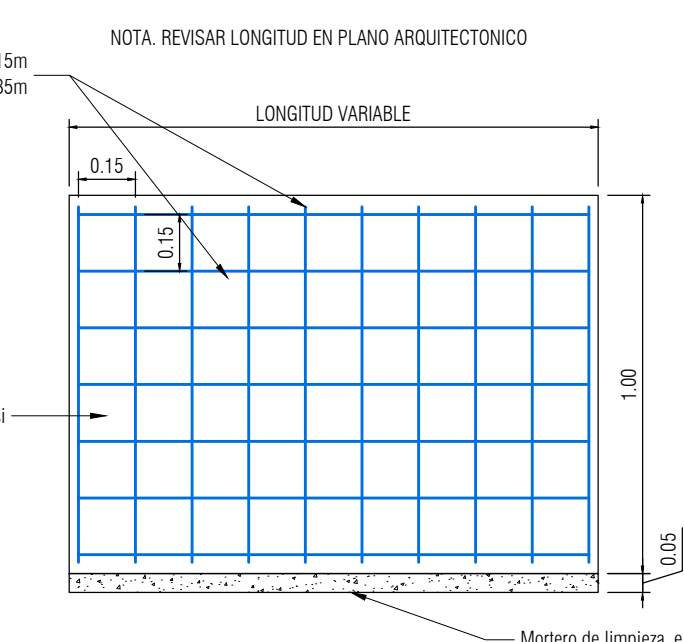
ALZADO TRANSVERSAL CONTENEDOR DE RAÍCES LONGITUDINAL VISTA EN CORTE ESCALA 1:20
