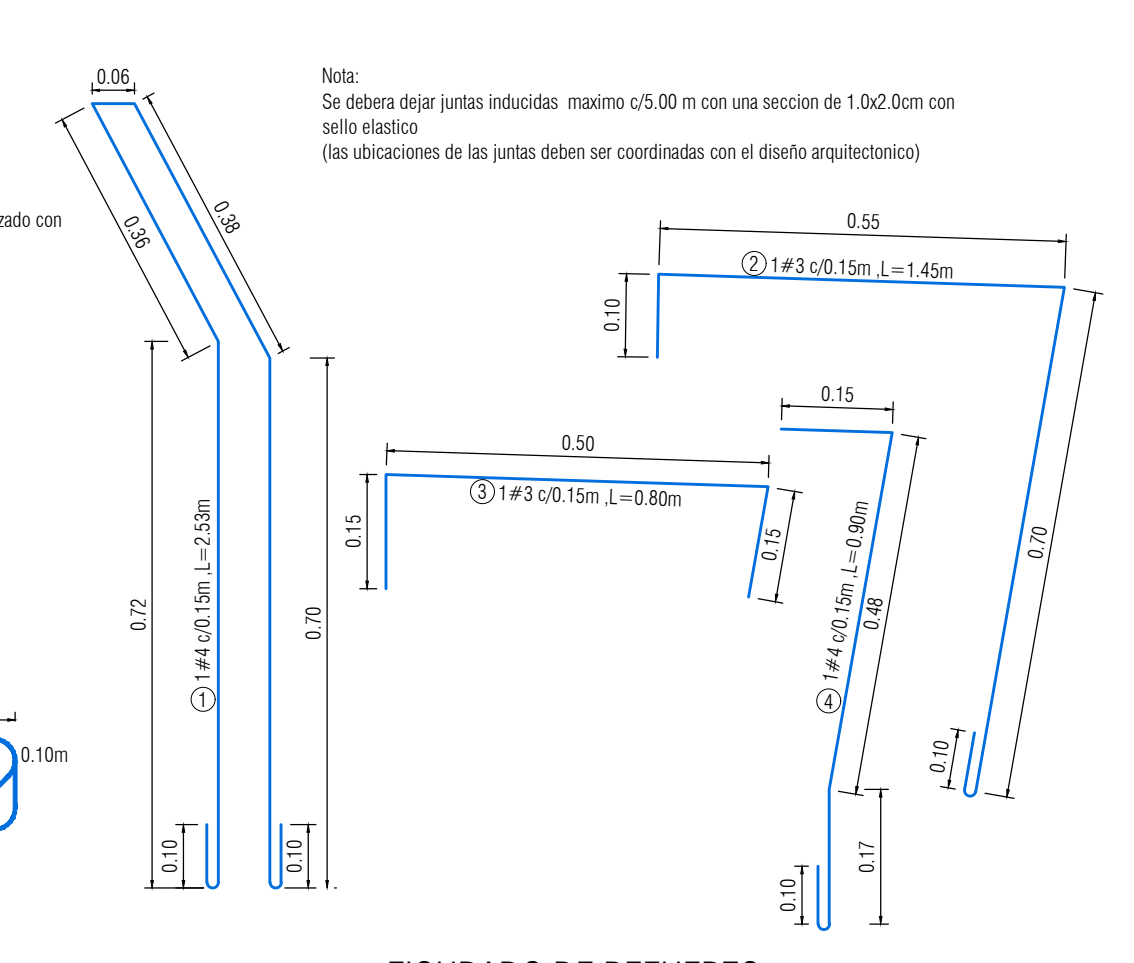
FIGURADO DE REFUERZO ESCALA 1:10
