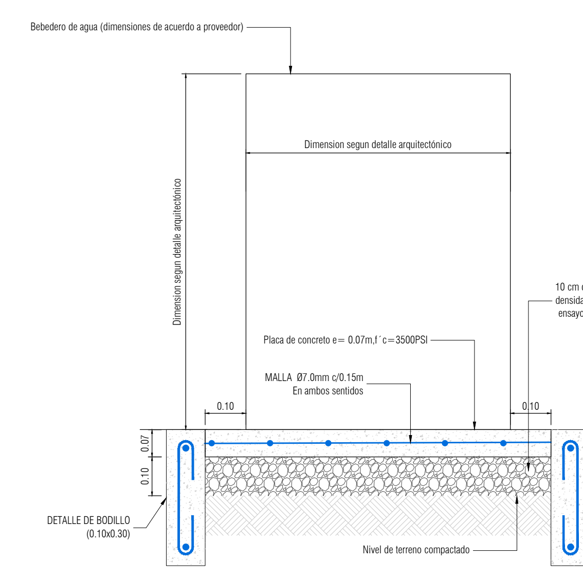
DETALLE ALZADO BEBEDERO DE AGUA DIMENSIONES Y REFUERZO ESCALA 1:10
