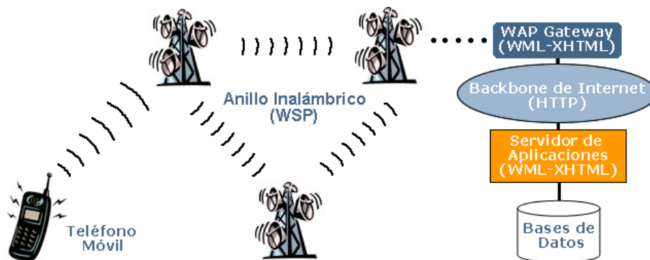
Figura 11. Arquitectura Cliente-Servidor de la Tecnología WAP
