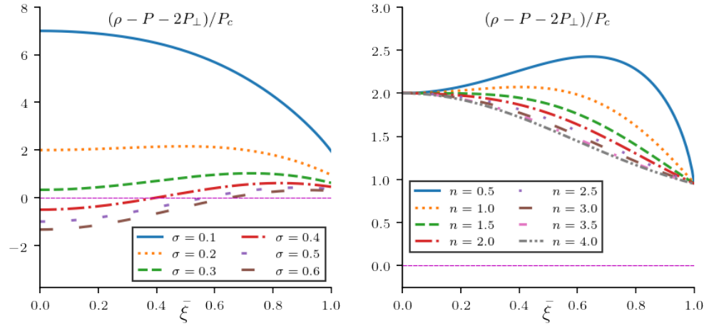
Figura 5.4: Condición de energía sobre la traza para modelos Lane-Emden maestra.
