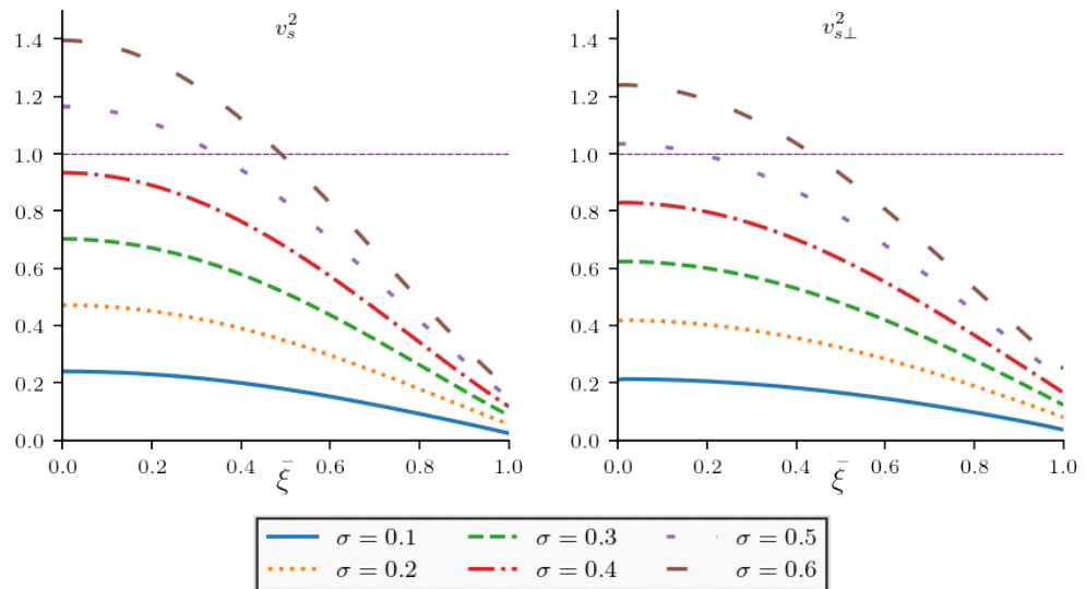
Figura 5.5: Velocidades del sonido, radial y tangencial, al cuadrado para modelos Lane-Emden maestra.
