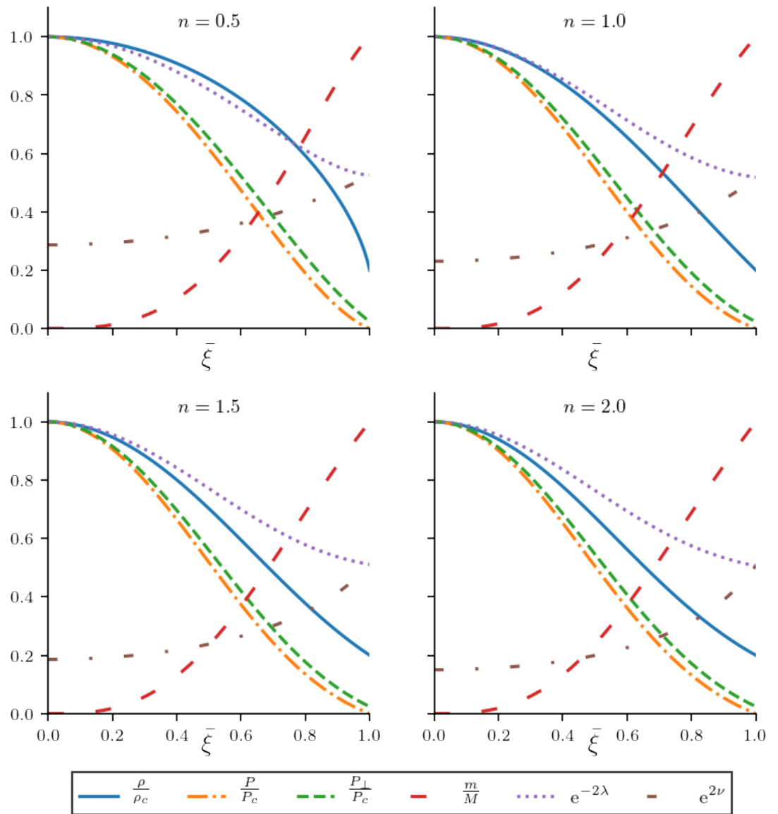
Figura 4.1: Variables físicas adimensionales y funciones métricas para modelos Lane-Emden maestra.
