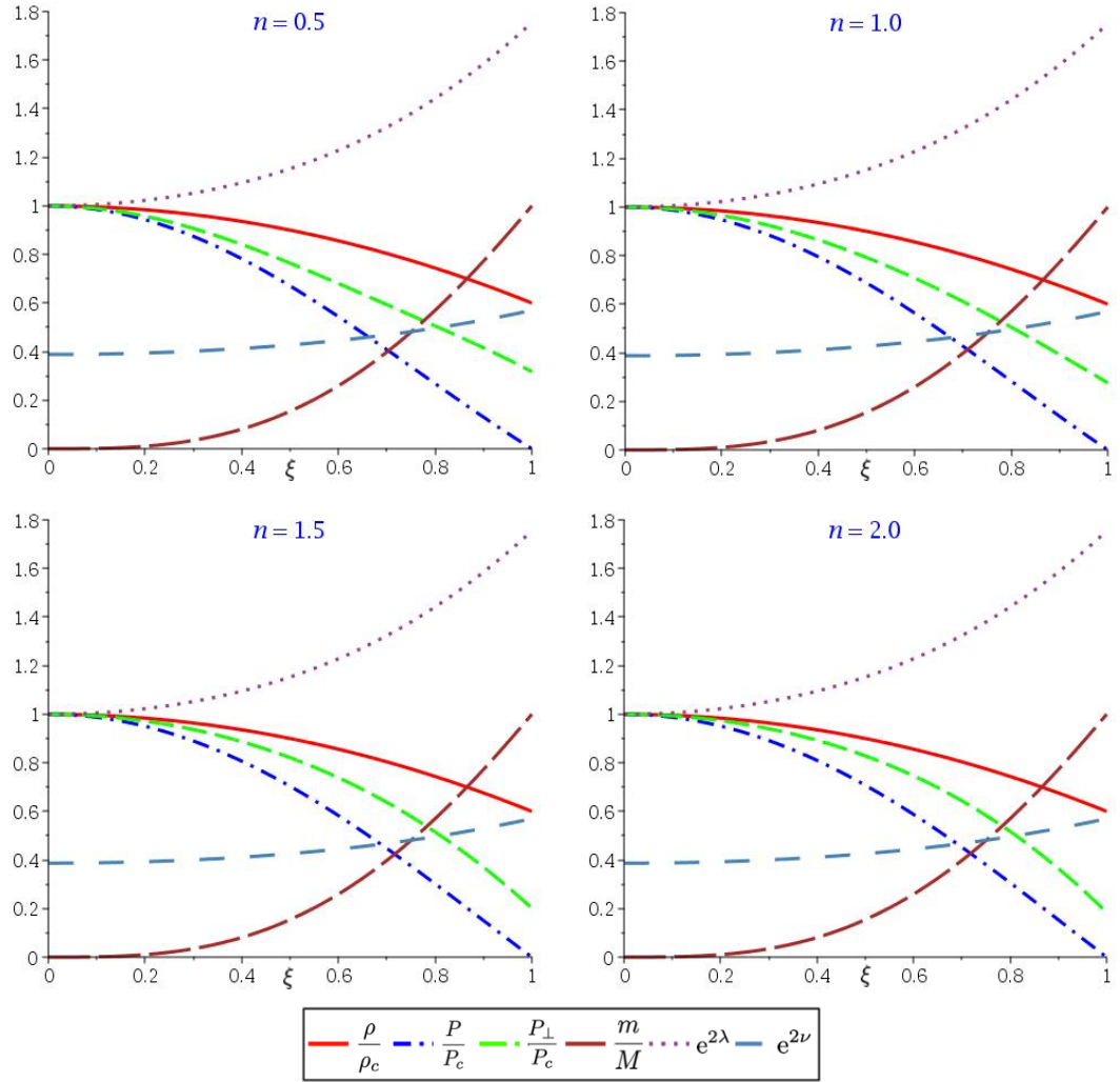
Figura 4.2: Variables físicas adimensionales y funciones métricas para modelos EoS-1.
