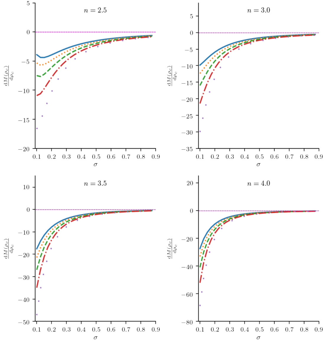
Figura H.2: dM(\rho_c)/d\rho_c en función de \sigma para la ecuación de Lane-Emden Lane-Emden maestra (b).
