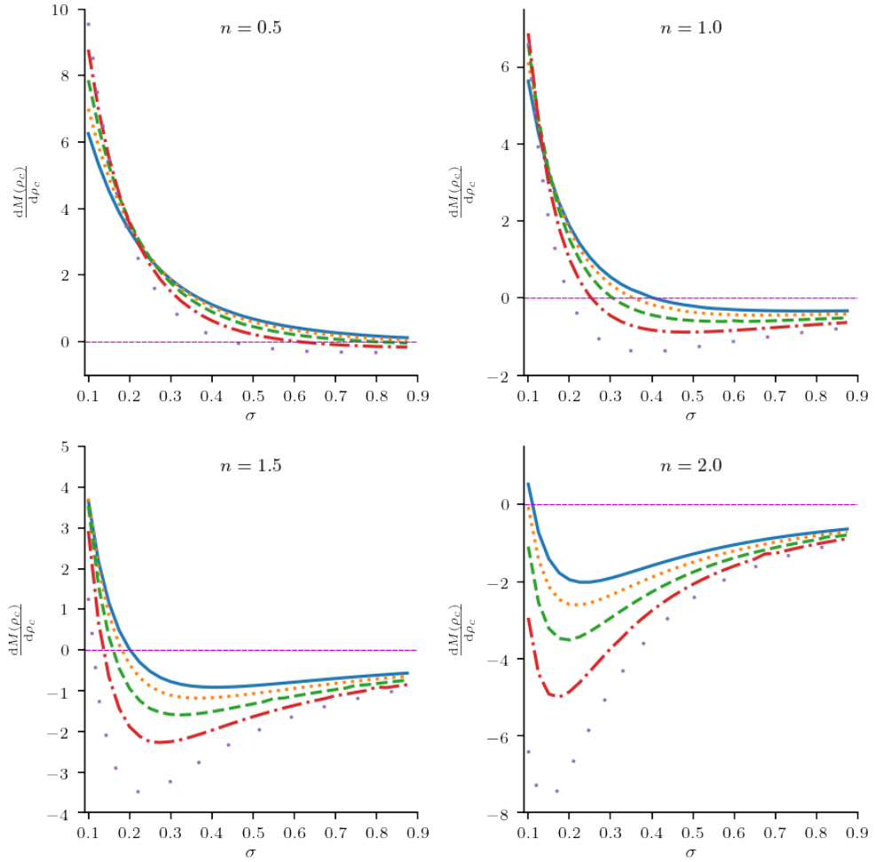
Figura H.1: dM(\rho_c)/d\rho_c en función de \sigma para la ecuación de Lane-Emden maestra (a).
