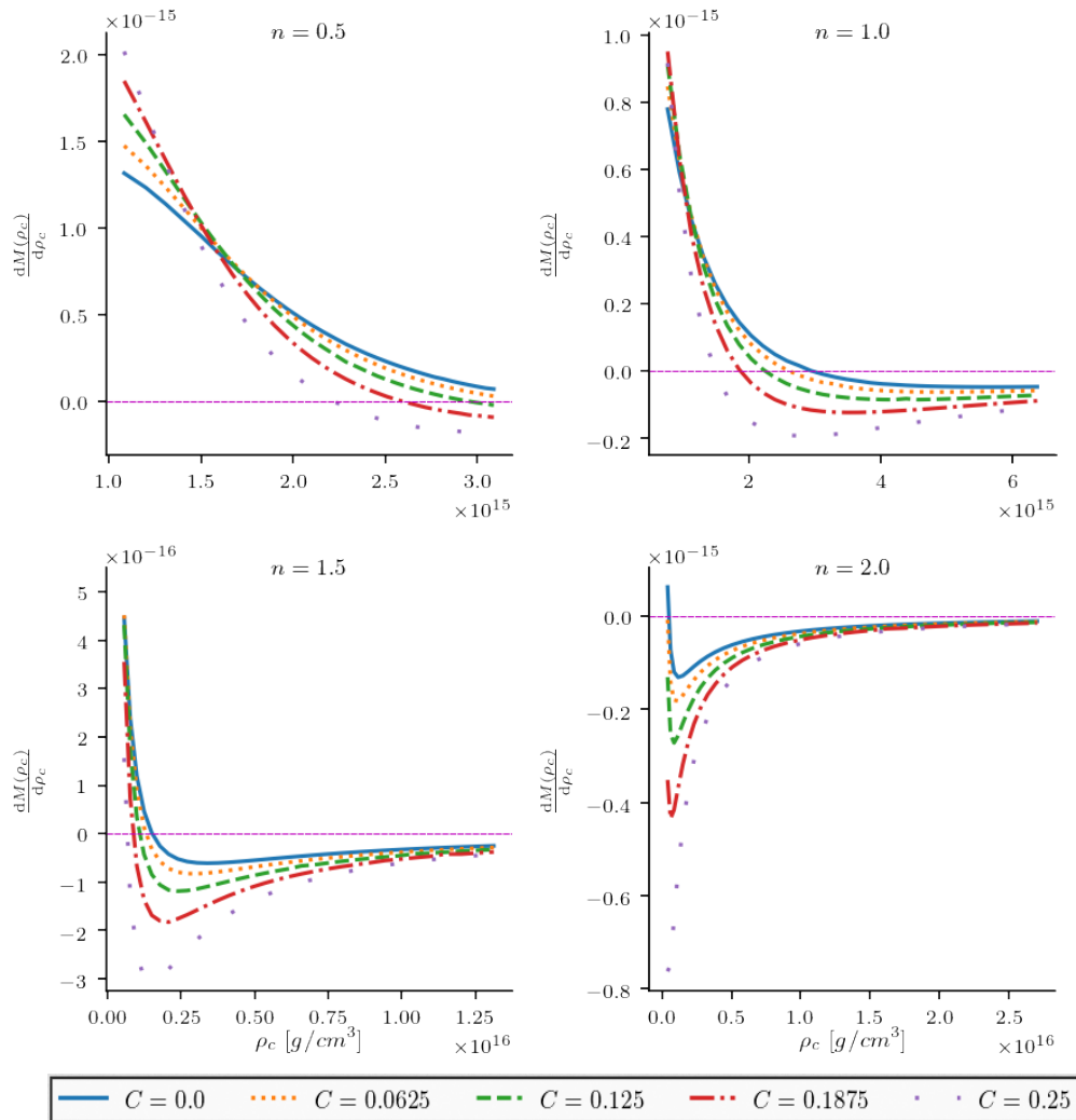
Figura 5.7: dM(\rho_c)/d\rho_c en función de \rho_c para modelos Lane-Emden maestra.
