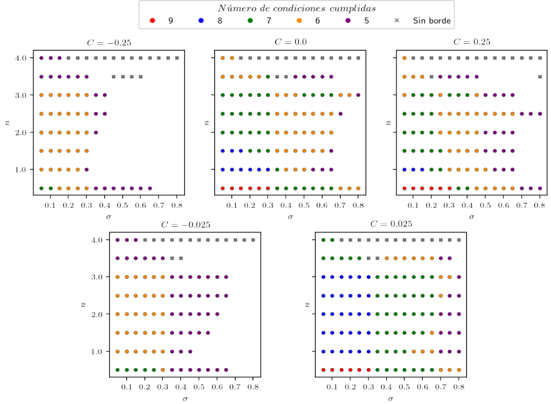
Figura 5.12: Rebanadas del espacio de parámetros de la EoS polítropa II para distintos valores de C .
