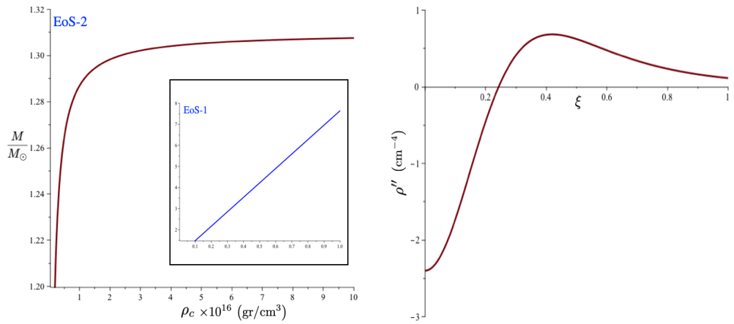
Figura 5.16: Masa total en función de la densidad central, y segunda derivada de la densidad de energía para modelos EoS-1 y EoS-2.
