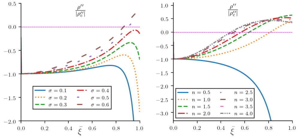
Figura 5.9: Segunda derivada de la densidad adimensional para modelos Lane-Emden maestra.
