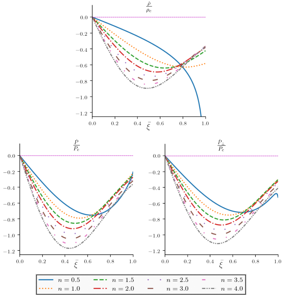
Figura 5.3: Gradientes de densidad de energía, de presión radial y de presión tangencial para modelos Lane-Emden maestra.
