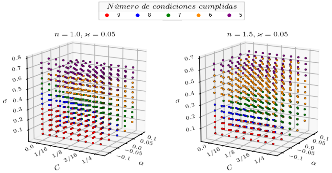
Figura H.4: Espacio de parámetros para la EoS polítropa maestra. Modelos con índice polítropo n = 1.0 y 1.5 .
