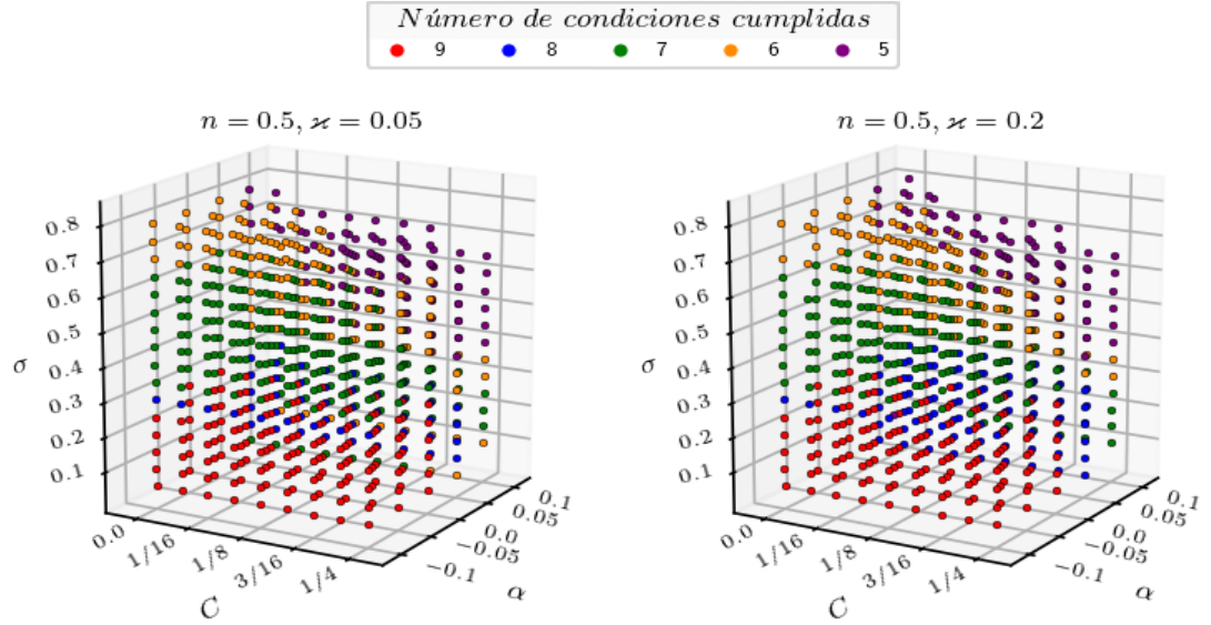
Figura 5.11: Espacio de parámetros para la EoS polítropa maestra, para modelos con índice polítripo n = 0.5 .
