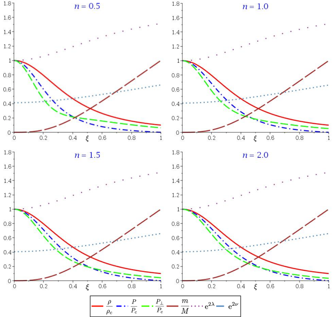
Figura 4.3: Variables físicas adimensionales y funciones métricas para modelos EoS-2.
