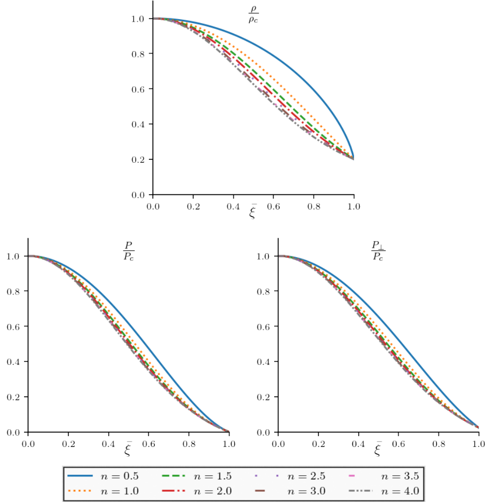
Figura 5.2: Densidad de energía, presión radial y presión tangencial para modelos Lane-Emden maestra.
