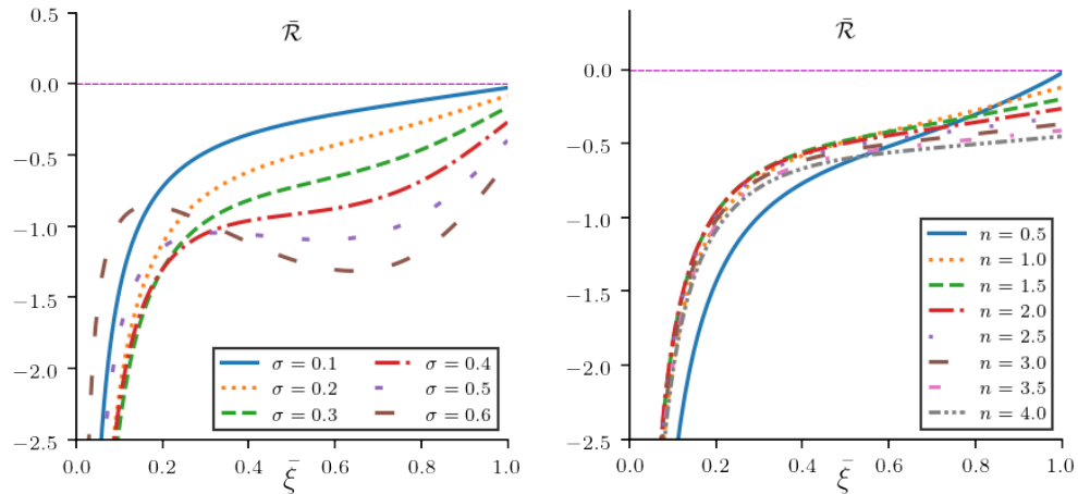
Figura 5.8: Ecuación de equilibrio hidrostático perturbada adimensional para modelos Lane-Emden maestra.
