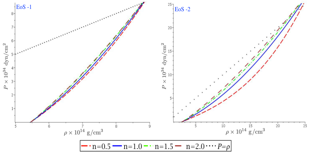
Figura 5.13: Presión radial como función de la densidad de energía para modelos EoS-1 (izquierda) y EoS-2 (derecha).
