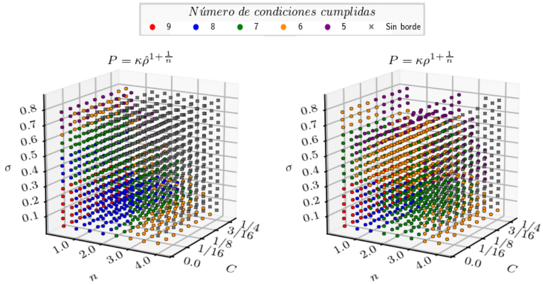
Figura 5.10: Espacio de parámetros para las EoS polítropa estándar.
