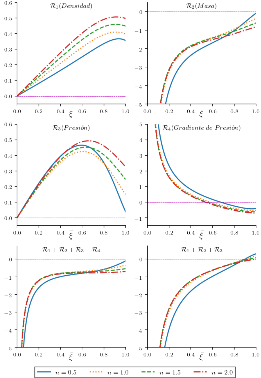
Figura H.3: Términos de la ecuación de equilibrio hidrostático perturbada para modelos Lane-Emden maestra.
