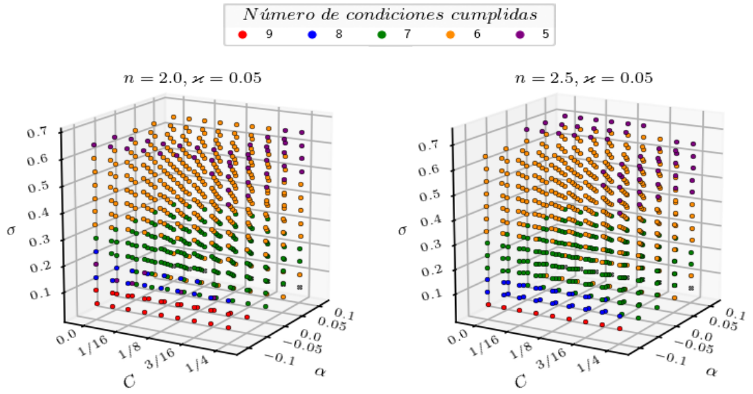
Figura H.5: Espacio de parámetros para la EoS polítropa maestra. Modelos con índice polítropo n = 2.0 y 2.5 .
