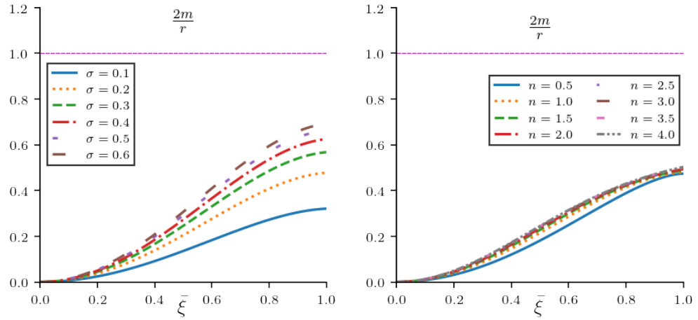
Figura 5.1: Compacidad para modelos Lane-Emden maestra.
