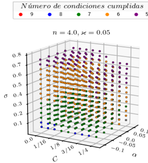
Figura H.7: Espacio de parámetros para la EoS polítropa maestra. Modelos con índice polítropo n = 4.0 .
