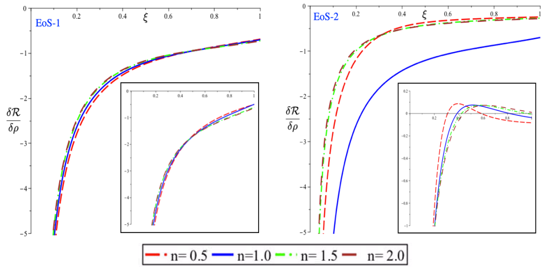
Figura 5.17: Ecuación de equilibrio perturbada para modelos EoS-1 y EoS-2.
