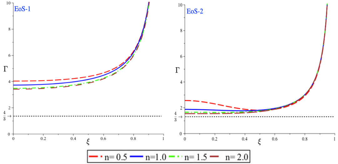
Figura 5.14: Índice adiabático para modelos EoS-1 y EoS-2.
