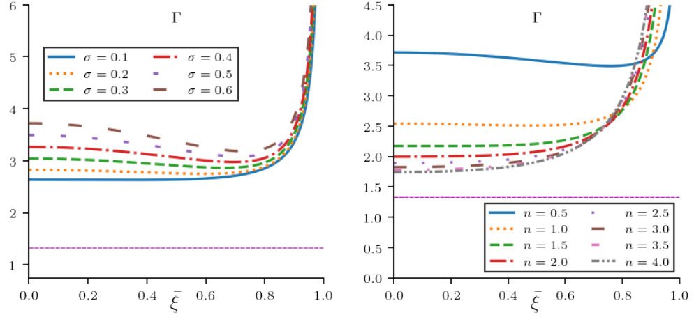
Figura 5.6: Índice adiabático para modelos Lane-Emden maestra.
