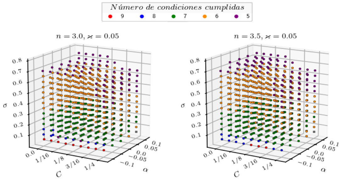
Figura H.6: Espacio de parámetros para la EoS polítropa maestra. Modelos con índice polítropo n = 3.0 y 3.5 .
