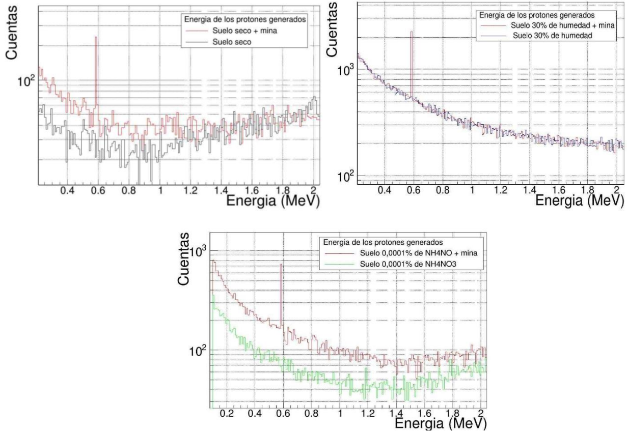
Figura 9. Espectro de energía de los protones generados en la interacción de tres sistemas suelo-mina con un flujo de secundarios de 24 hr. Se puede observar con claridad que el pico alrededor de 0.58 MeV se produce en presencia de la mina. Este criterio se podría utilizar para la detección de estos dispositivos.
