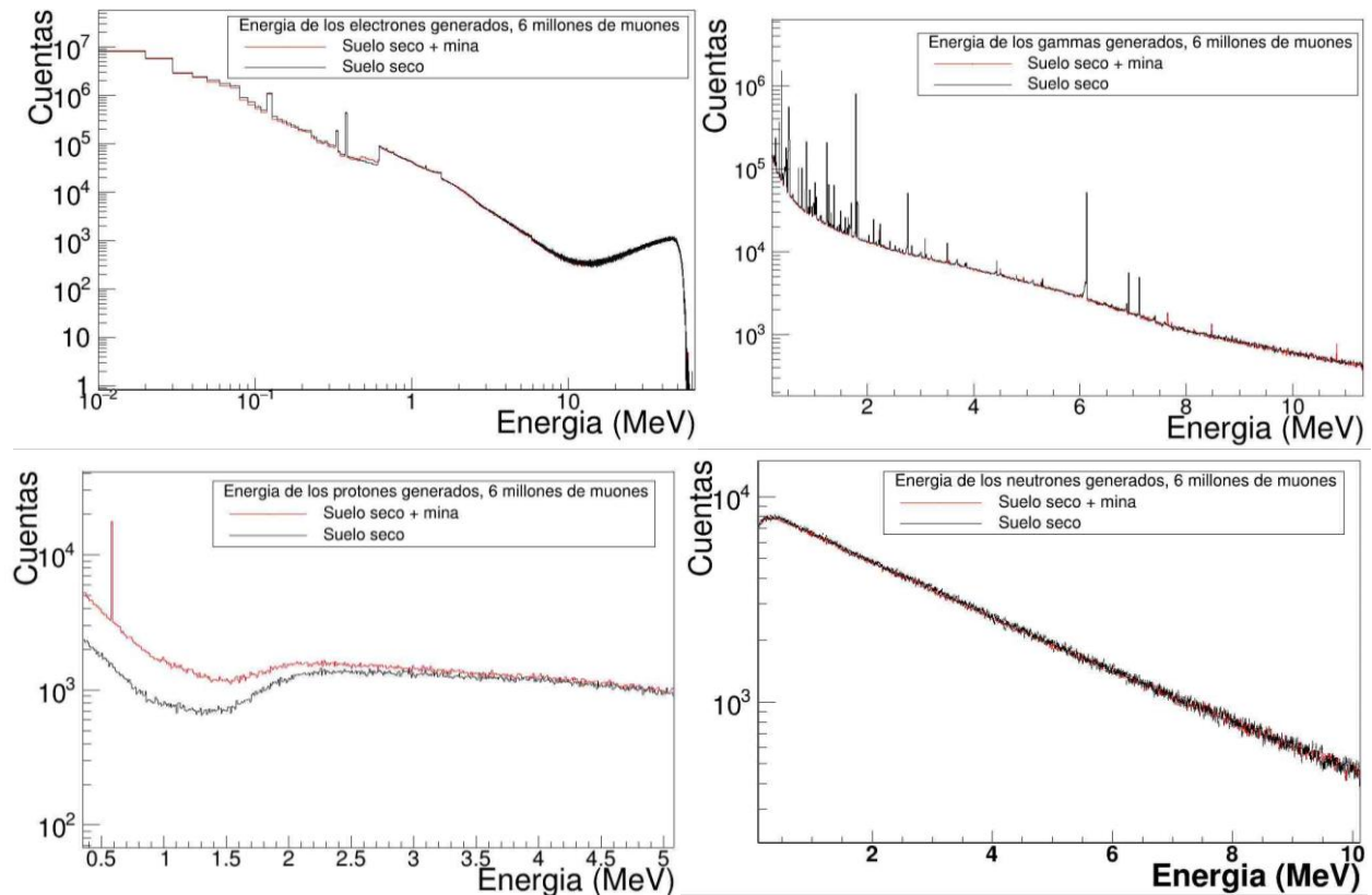
Figura 12. Espectros de energía de las partículas generadas en la interacción de los muones de 500 MeV con las diferentes configuraciones del sistema suelo modelo seco-mina. Espectro de energía de los electrones (Arriba izquierda). Espectro de energía de los fotones (Arriba derecha). Espectro de energía de los neutrones (Abajo izquierda). Espectro de energía de los protones (Abajo derecha). En las gráficas de los electrones y neutrones, las líneas se superponen a lo largo de todo el espectro, indicando que no es posible diferenciar las energías de estas partículas. Por otro lado, en las gráficas de los gamma y los protones, existen puntos en los cuales se diferencian los espectros; para los gamma se presenta en los picos de energía de 6.13 MeV, 8.4 MeV y 10.826 MeV; para los protones la diferencia está en el rango de 0.1 MeV hasta los 2 MeV, con un pico alrededor de 0.58 MeV que aparece en el suelo minado.
