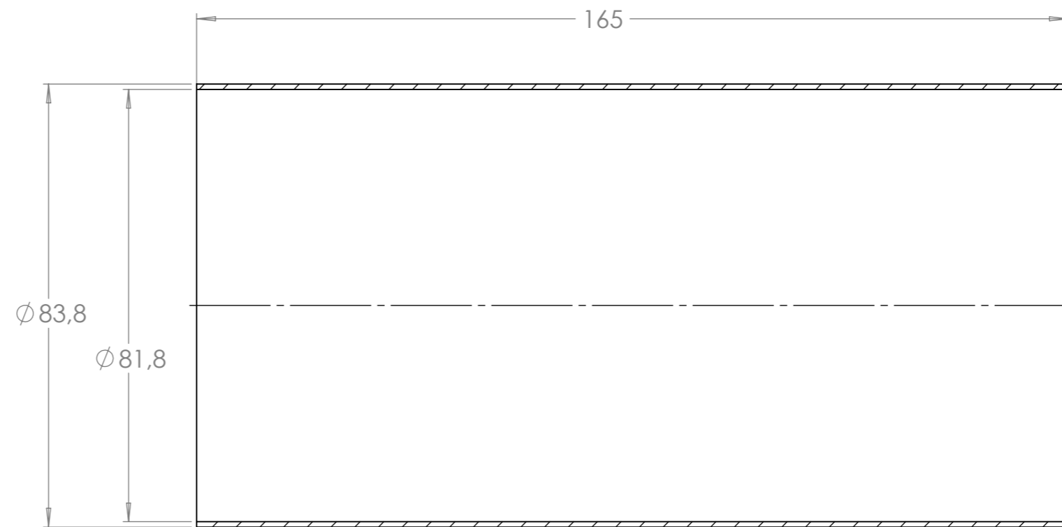
SECCIÓN F-F
