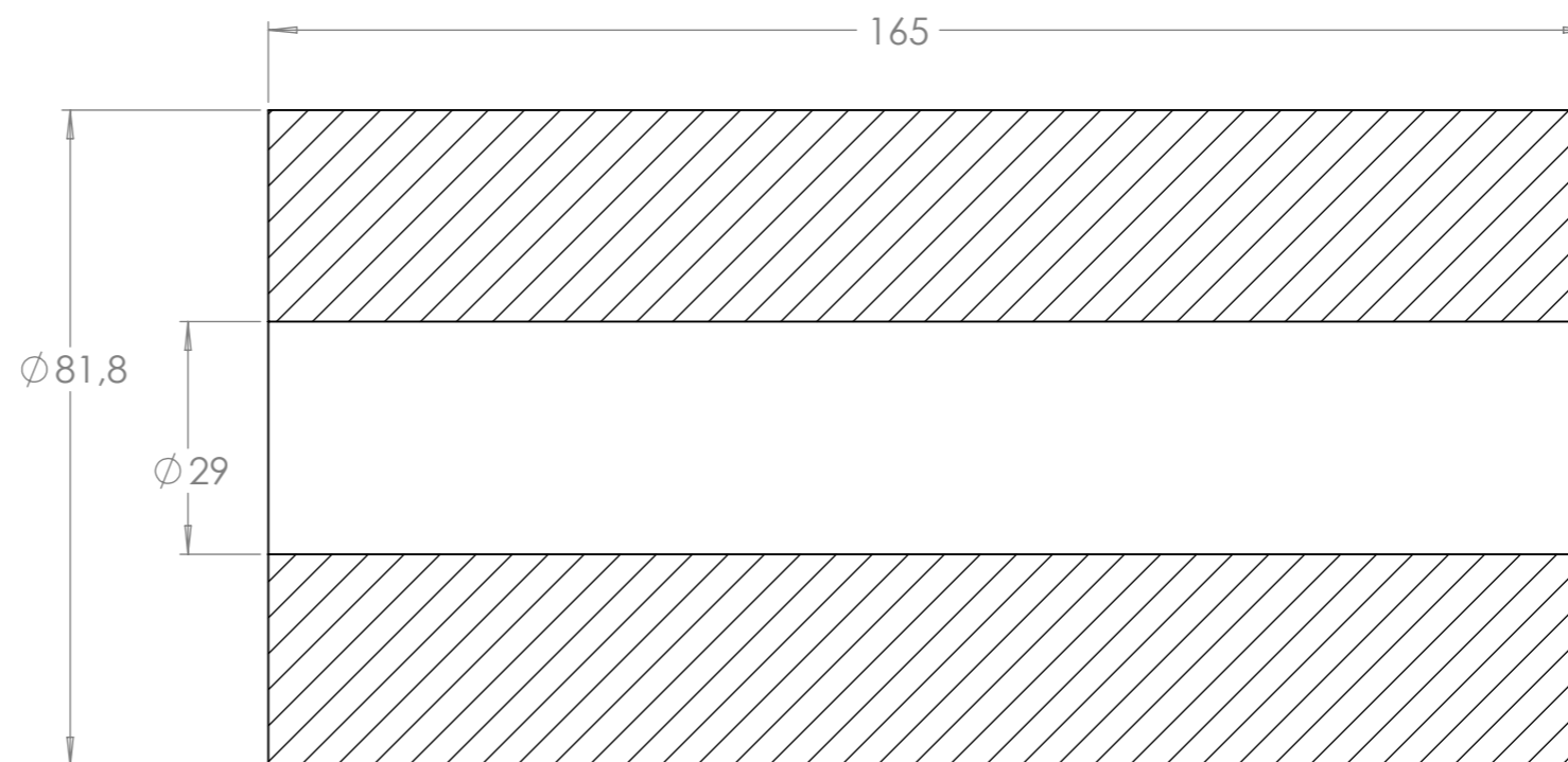
SECCIÓN G-G
