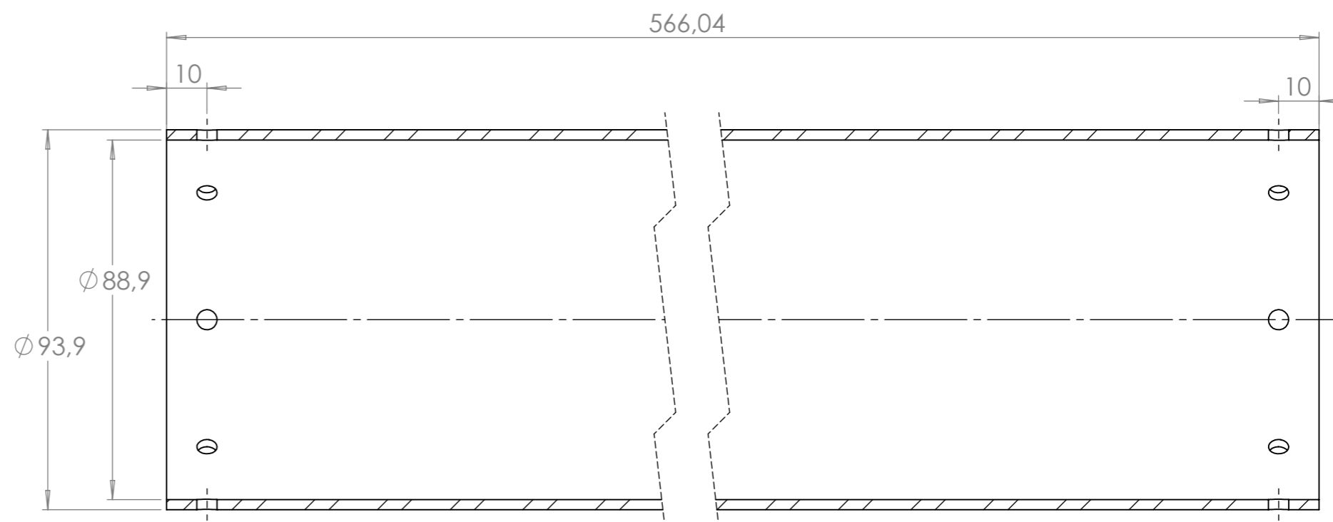
SECCIÓN B-B
