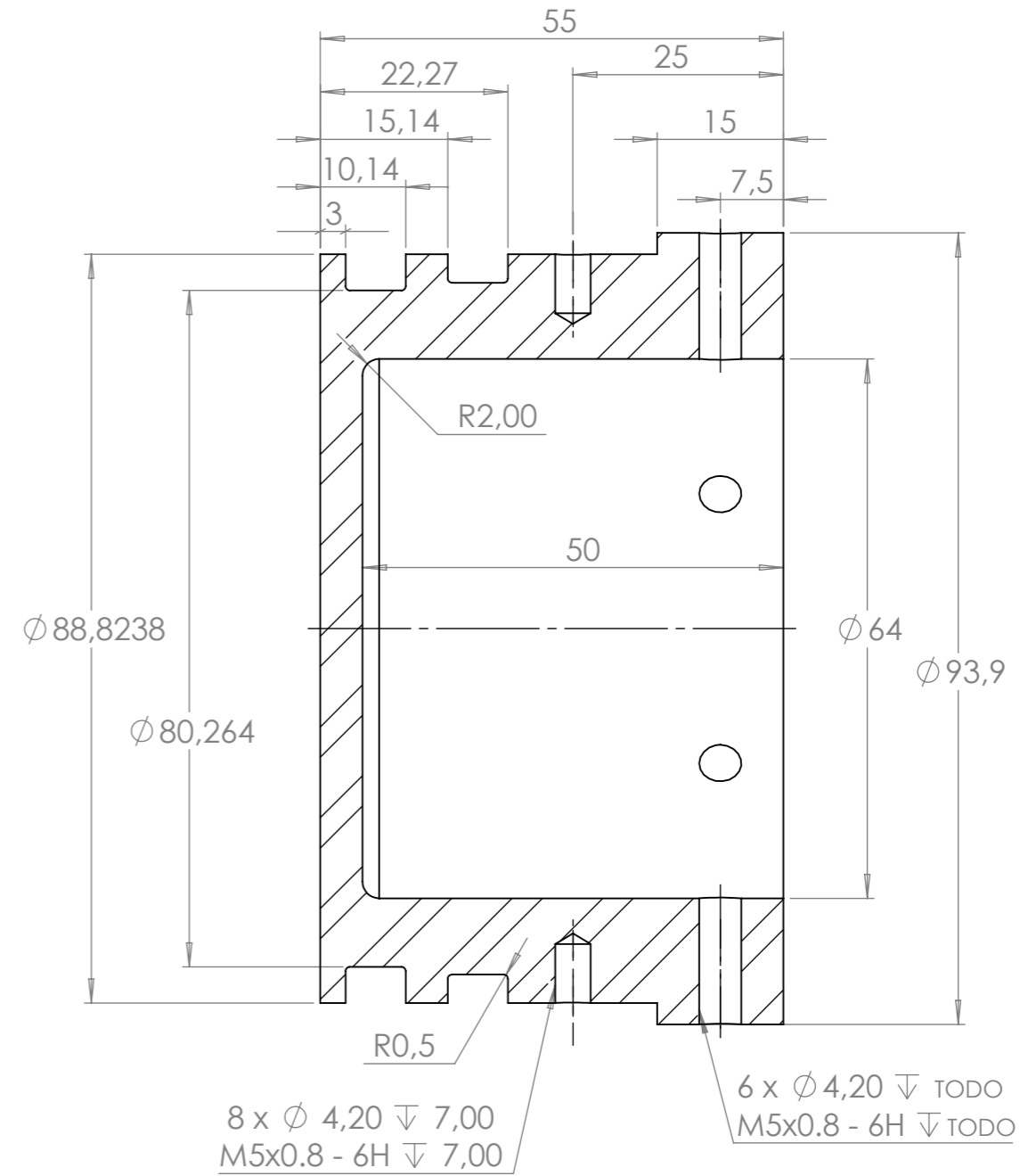
SECCIÓN D-D
