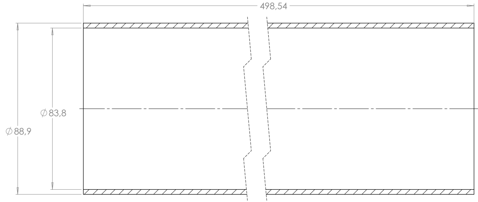
SECCIÓN E-E
