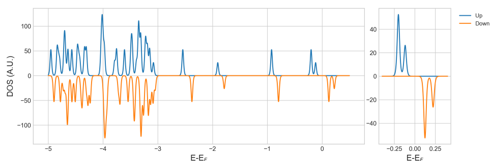
Figura 18. Densidad de estados para cluster Ag_{12}Bi_L y zoom cerca al nivel de Fermi
