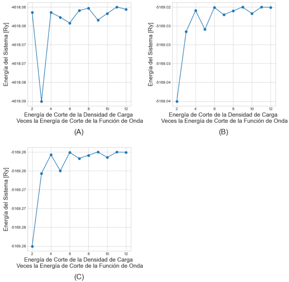
Figura 13. Gráfico de convergencia de la energía de corte ( E_{cutrho} ) respecto a la energía del sistema para: Cluster Ag_{13} (A), Cluster Ag_{12}Bi_C (B) y Cluster Ag_{12}Bi_L (C)
