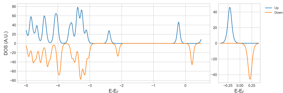
Figura 16. Densidad de estados para cluster Ag_{13} y zoom cerca al nivel de Fermi
