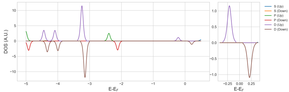
Figura 20. Densidad de estados proyectada por orbital atómico del átomo central del cluster Ag_{13} y zoom cerca al nivel de Fermi
