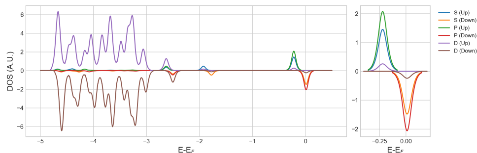
Figura 21. Densidad de estados proyectada por orbital atómico de un átomo lateral del cluster Ag_{12}Bi_C y zoom cerca al nivel de Fermi
