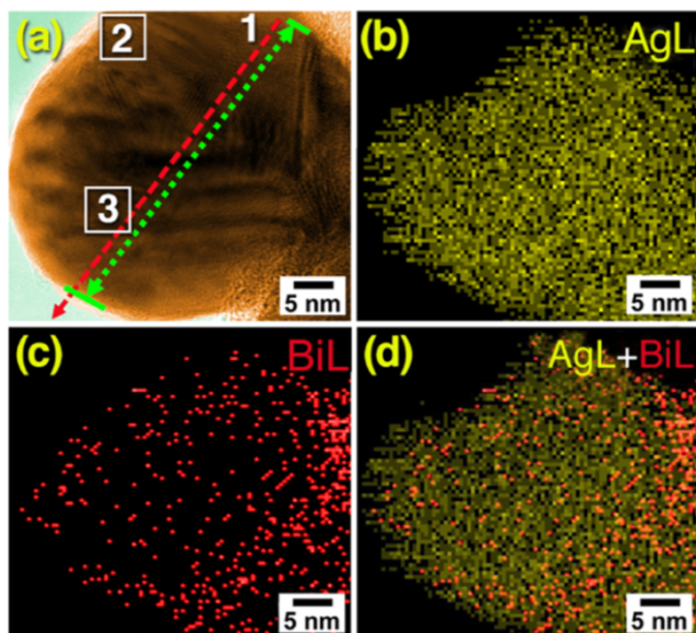
Figura 4. Caracterización de nanopartículas de plata con bismuto: (a) HR-TEM de Na de plata y bismuto de 43 nm de tamaño. (b) EDS de los átomos de plata en la Na. (c) EDS de los átomos de bismuto en la Na. (d) Sobreposición de los resultados de EDS de los átomos de plata y bismuto en la Na.
