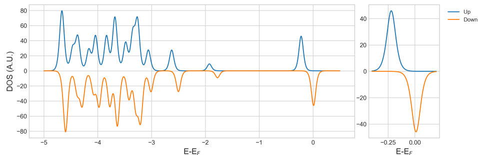
Figura 17. Densidad de estados para cluster Ag_{12}Bi_C y zoom cerca al nivel de Fermi
