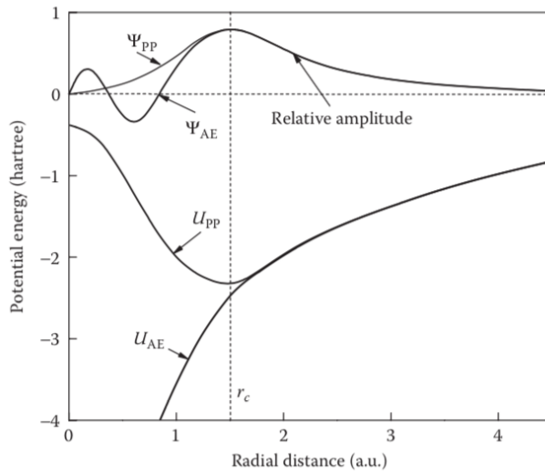
Figura 8. Pseudofunción de onda, generada a partir de un Norm-conserving PPs, comparada con su respectiva auto función de Kohn-Sham
