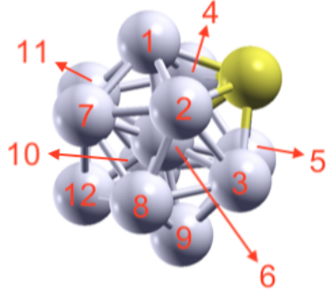
Figura 15. Enumeración de los átomos de plata respecto al átomo de bismuto para el cluster Ag_{12}Bi_L
