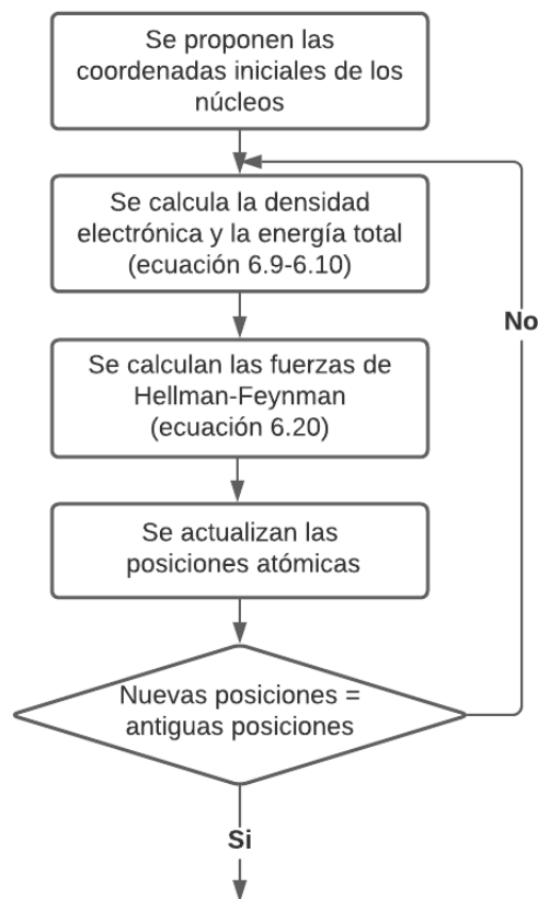
Figura 7. Ilustración del ciclo iterativo para el cálculo de las coordenadas finales de un material.
