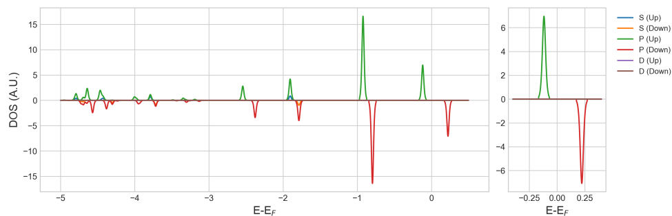
Figura 23. Densidad de estados proyectada por orbital atómico del átomo de bismuto del cluster Ag_{12}Bi_L y zoom cerca al nivel de Fermi
