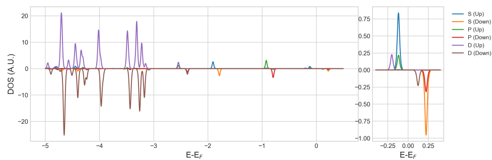
Figura 27. Densidad de estados proyectada por orbital atómico del átomo de plata lejano del cluster Ag_{12}Bi_L y zoom cerca al nivel de Fermi
