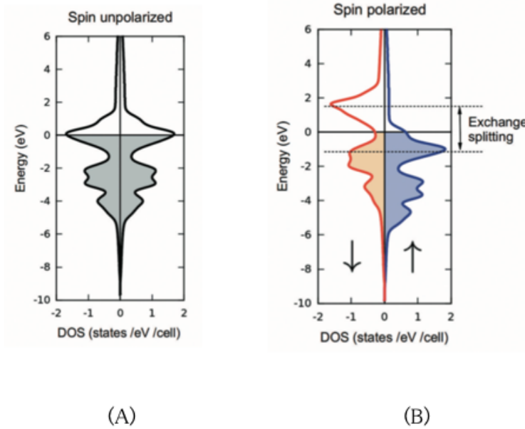
Figura 6. Densidad de estados spin up y down, para estructura de Hierro centrada en el cuerpo, sin polarización de spin (A) y con polarización del spin (B)
