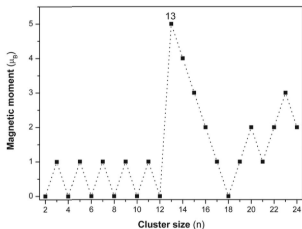
Figura 3. Momento magnético vs número de átomos del cluster de plata
