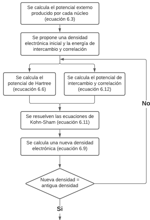
Figura 5. Ilustración del método autoconsistente empleado en DFT para el cálculo de la densidad electrónica
