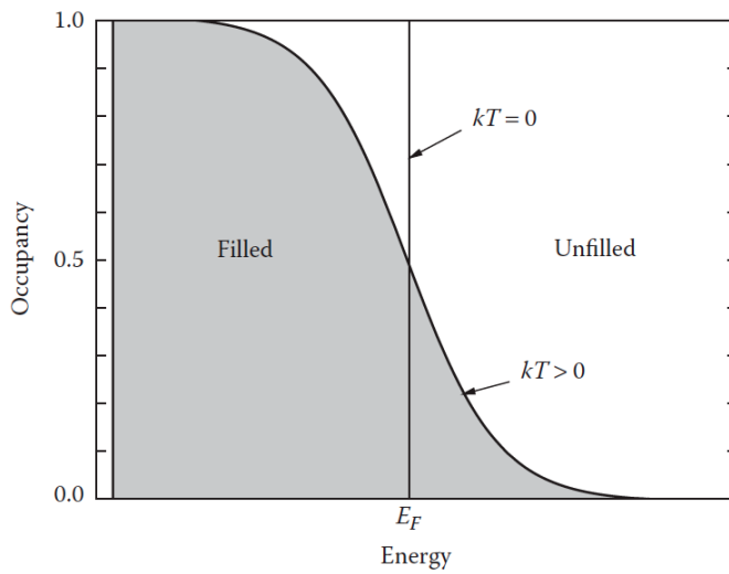
Figura 9. Ilustración de la distribución de Fermi-Dirac para K=0 y K>0 .
