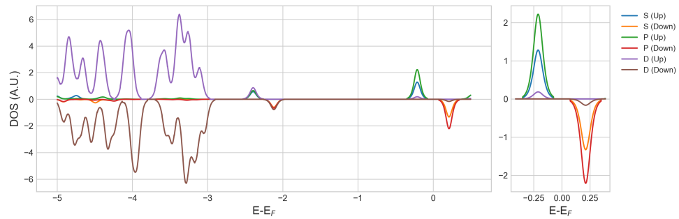
Figura 19. Densidad de estados proyectada por orbital atómico de un átomo lateral del cluster Ag_{13} y zoom cerca al nivel de Fermi
