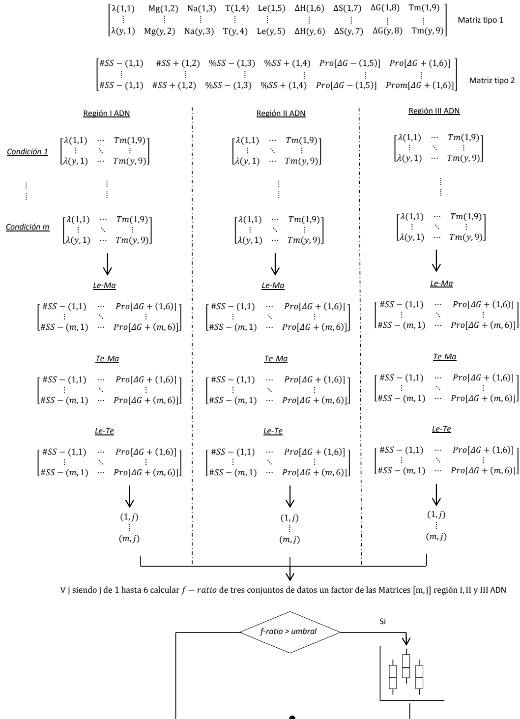
Figura 14. Esquema del proceso algorítmico de cálculos estadísticos y análisis inferencial
