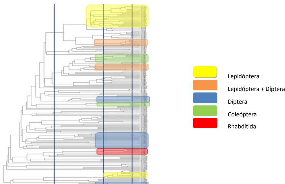
Figura 20. Filogenia de las toxinas Cry y letalidad asociada. Este Dendograma de toxinas Cry de tres dominios fue adaptado de http://www.lifesci.sussex.ac.uk/home/Neil_Crickmore/Bt/ y coloreado para indicar la especificidad insecticida de las toxinas, según la información registrada en las bases de datos del Natural Resources Canada, http://www.glfc.forestry.ca/bacillus/ .
