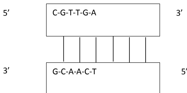
Figura 3. Representación de un fragmento de ADN
