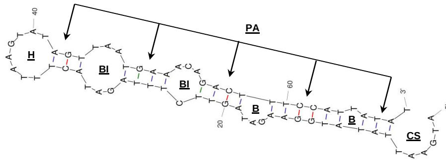
Figura 7. Motivos estructurales de un fragmento de la región I del gen cry11A.a. De izquierda a derecha: Horquilla (H), pares apilados (PA), bucle interno (BI), pares apilados (PA), bucle interno (BI), pares apilados (PA), bulto (B), pares apilados (PA), bulto (B), pares apilados (PA), ADN cadena sencilla (CS).
