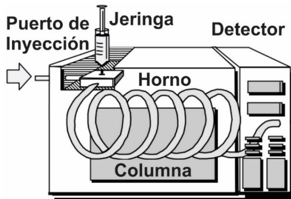
Figura 6. Esquema general de un cromatógrafo de gases.
