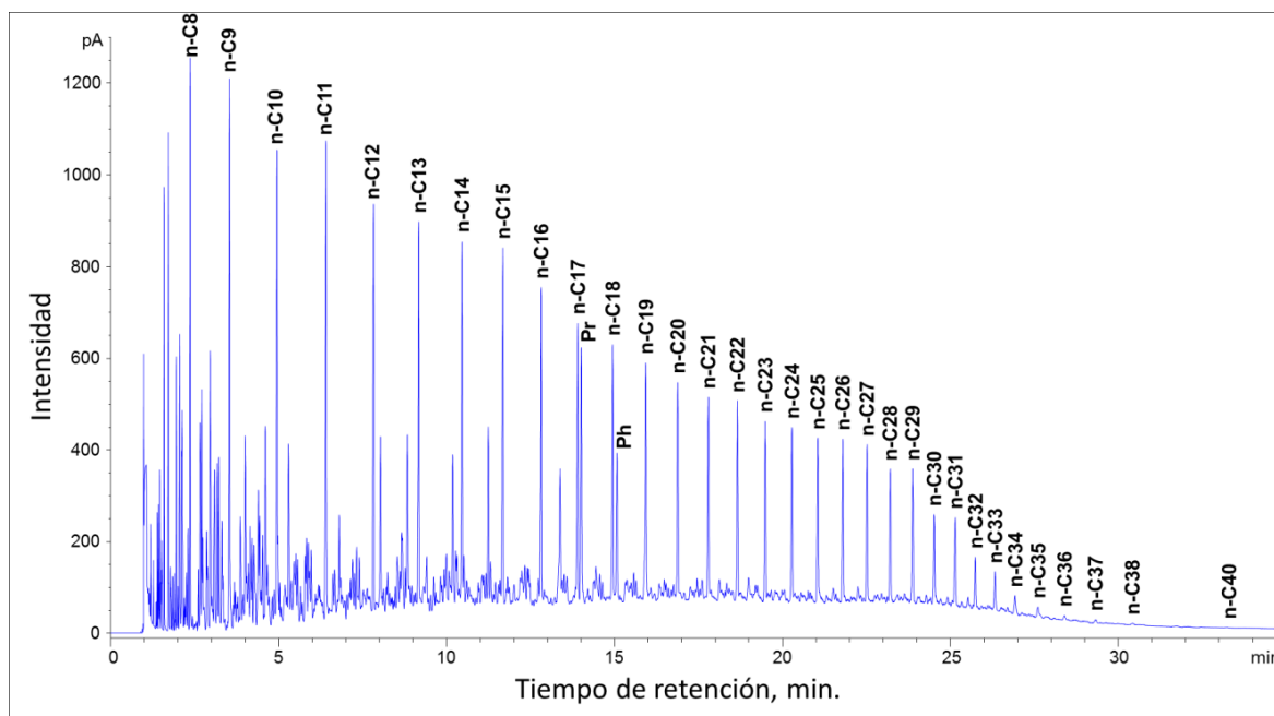
Figura 17. Perfil cromatográfico de la muestra de crudo ICAS 1695. Obtenido por GC-FID, columna DB-1 (30 m x 0.32 mm x 0.25 \mu m).
