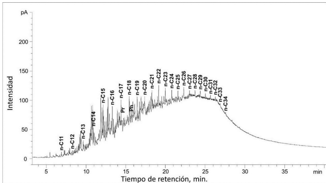
Figura 40. Perfil cromatográfico del extracto de bitumen después de hidropirólisis a 345 °C, por 48 h (EB 1211), obtenido por GC-FID. Columna DB-1 (30m x 0.32 mm x 0.25 \mu m).
