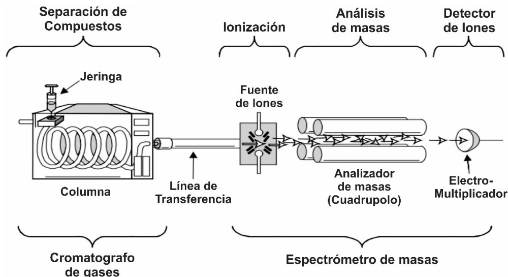
Figura 8. Esquema de un cromatografo de gases acoplado a un espectrómetro de masas, con analizador cuadrupolo.
