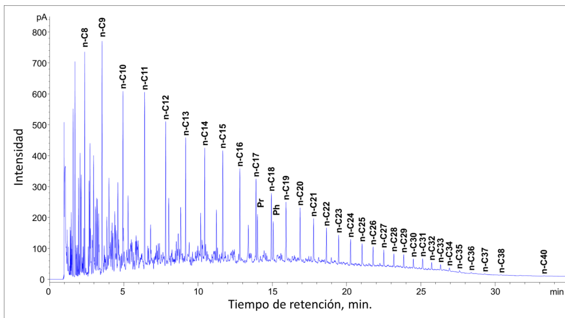
Figura 18. Perfil cromatográfico de la muestra de crudo ICAS 1118. Obtenido por GC-FID, columna DB-1 (30 m x 0.32 mm x 0.25 \mu m).
