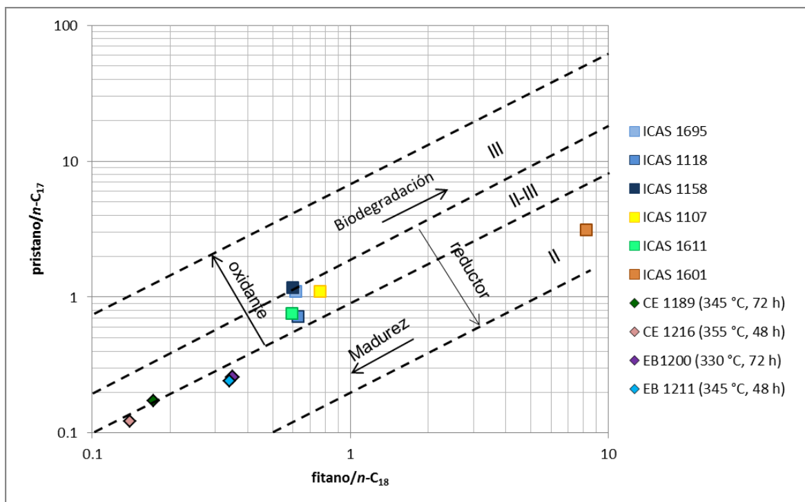
Figura 48. Gráfico de las relaciones pristano/ n -C 17 Vs fitano/ n -C 18 , para tipos de querógeno de cada una de las muestras analizadas.
