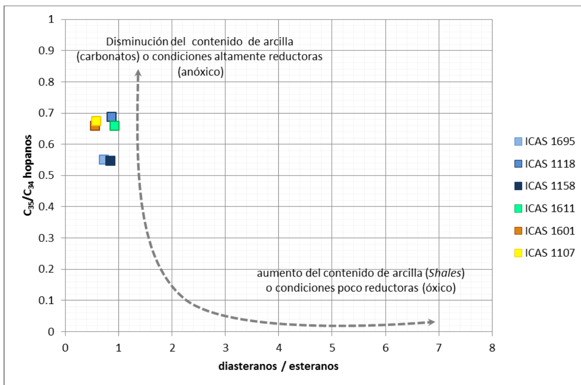
Figura 30. Gráfica C_{35} / C_{34} hopanos Vs diasteranos / esteranos.
