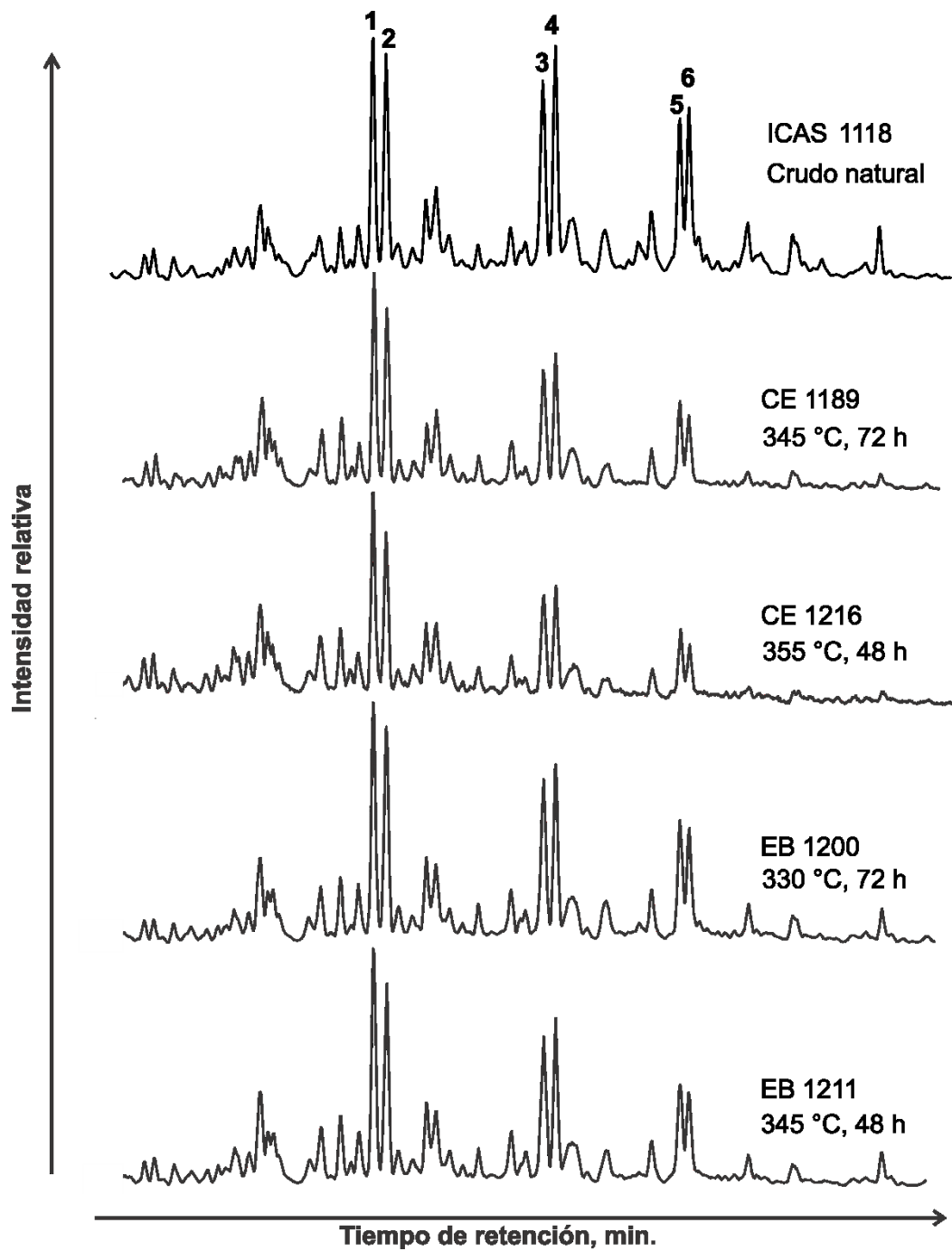
Figura 45. Corriente iónica extraída (ion m/z 218), de la fracción saturada, de muestras de crudo natural y productos obtenidos por hidropirólisis, pertenecientes a la formación la luna.
