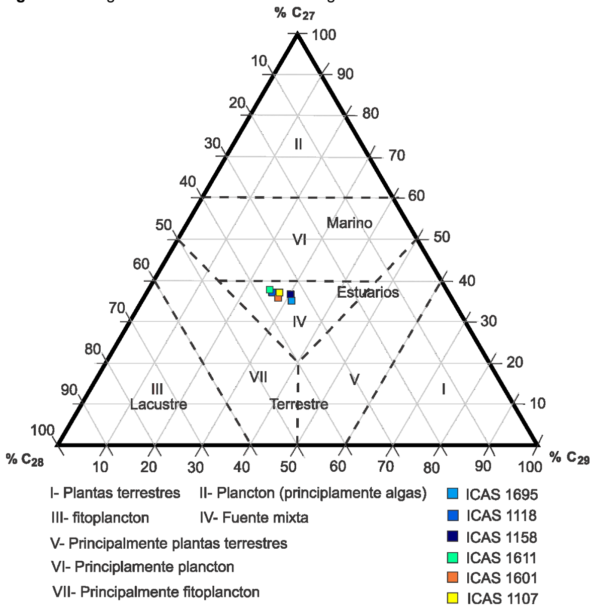
Figura 27. Diagrama ternario de esteranos regulares.
