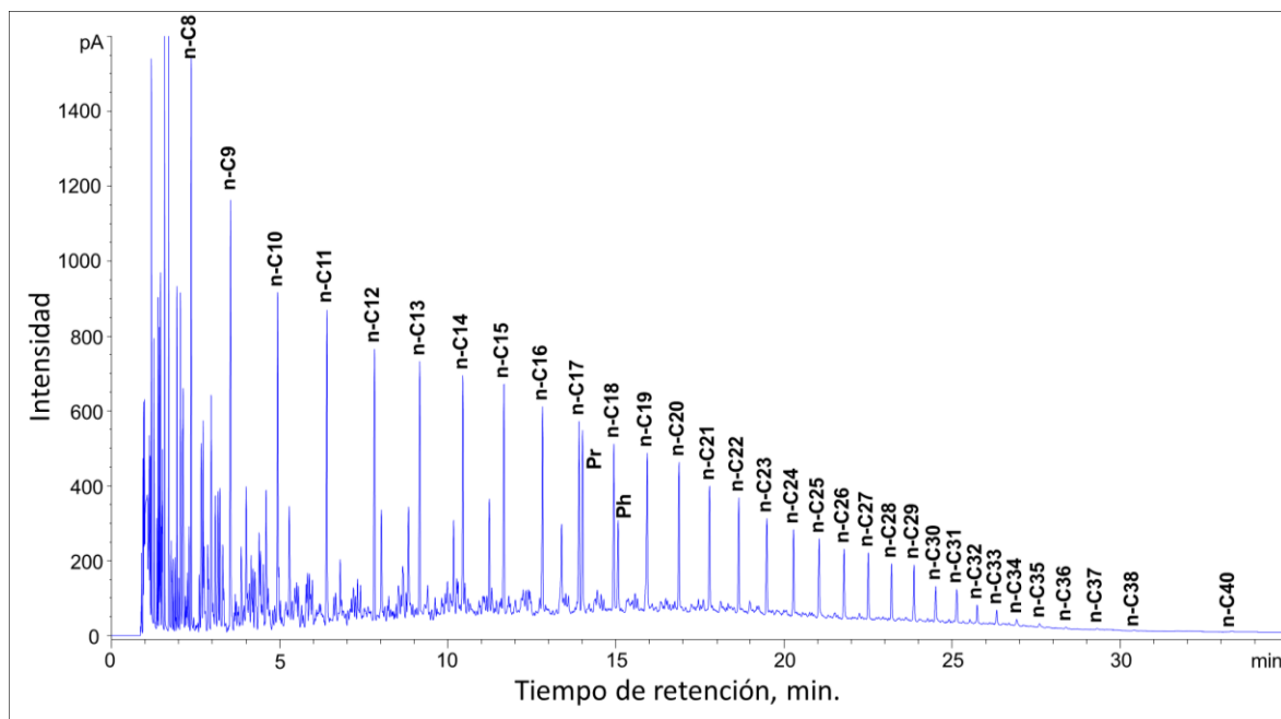
Figura 19. Perfil cromatográfico de la muestra de crudo ICAS 1158. Obtenido por GC-FID, columna DB-1 (30 m x 0.32 mm x 0.25 \mu m).
