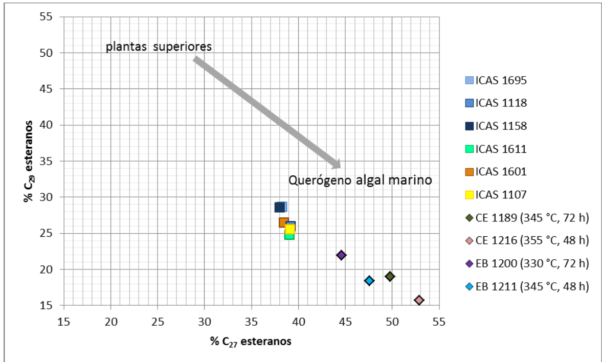
Figura 49. Grafica % C 29 esteranos Vs % C 27 esteranos.
