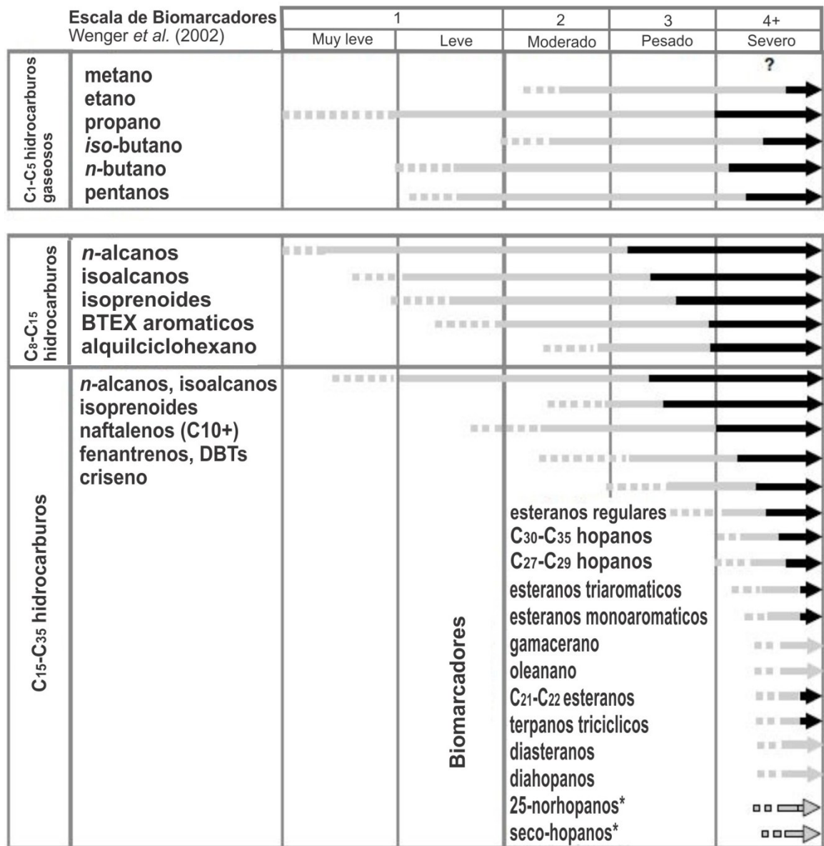
Figura 26. Secuencia generalizada de eliminación de los grupos moleculares seleccionados al aumentar los niveles de biodegradación.
