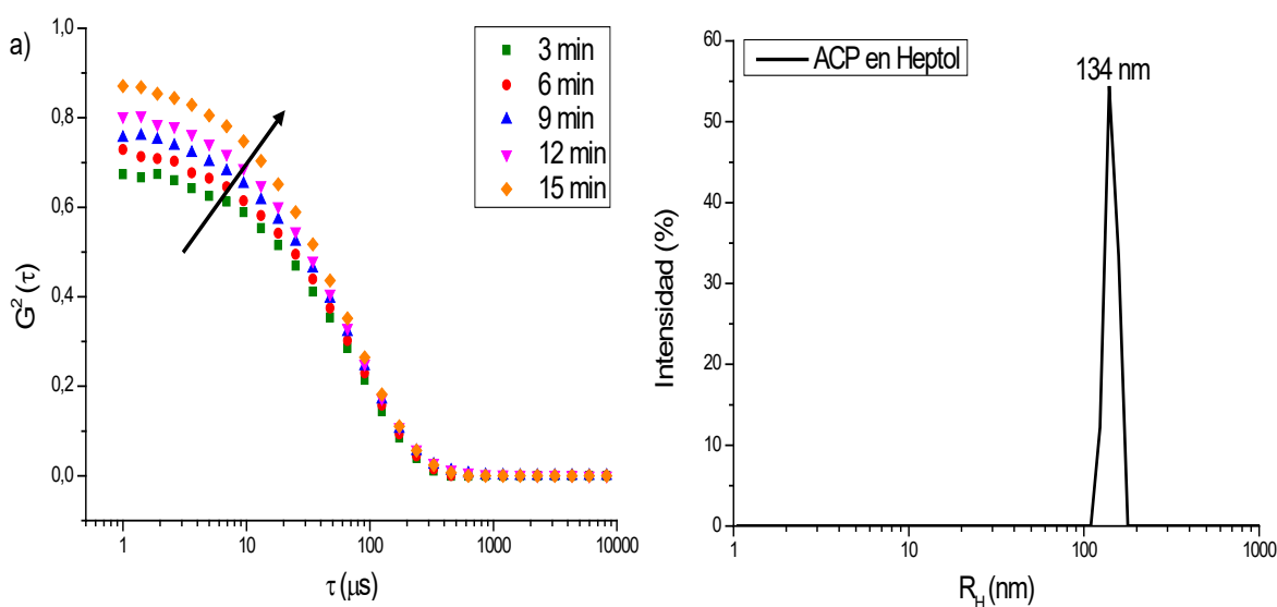
Figura 3.11 Funciones de correlación (a) y distribución de tamaño de partícula (b) del ACP en heptol (50% en volumen de n -heptano) a 25 °C.
