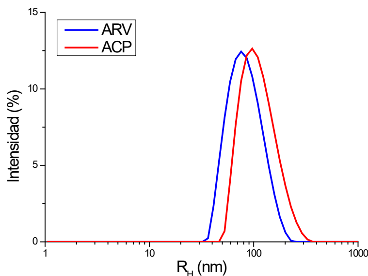
Figura 3.5 Distribuciones de tamaño de partícula de los asfaltenos en tolueno (0.1% p/v) medidas a 25 °C y 30 min de tiempo de envejecimiento
