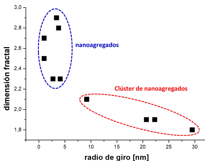
Figura 3.9 Correlación entre R_g y d_f derivados del ajuste del modelo unificado multinivel.
