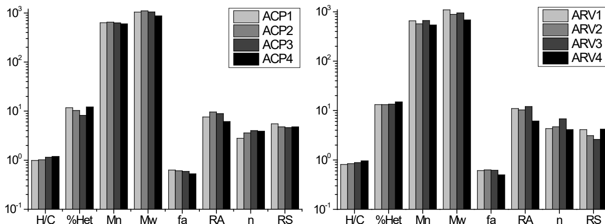
Figura 3.4 Propiedades moleculares de las sub-fracciones ACP (izquierda) y ARV (derecha) obtenidas del análisis elemental, MS y NMR
