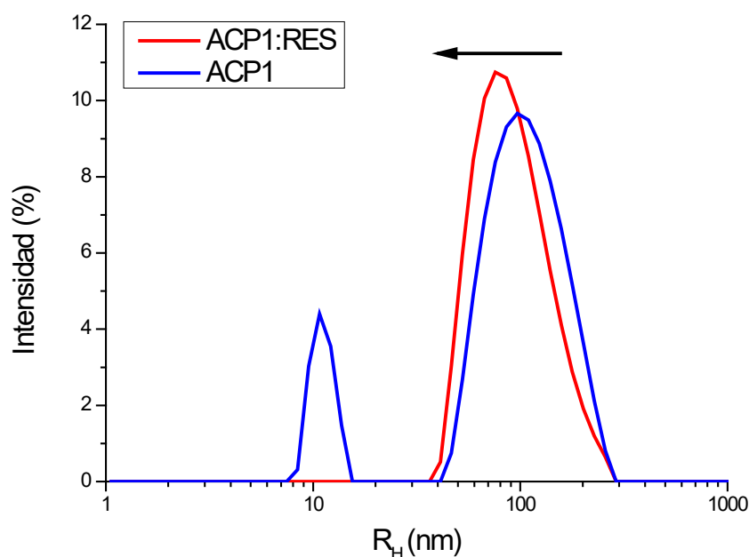
Figura 3.13 Comparación de la distribución de tamaño de partícula para soluciones en tolueno de la sub-fracción ACP1 (azul) y de la mezcla ACP1:RES (rojo)
