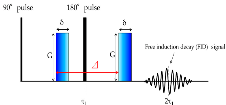
Figura 2.3 Secuencia de pulsos eco de espín de gradiente de campo pulsado. Adaptado de Johnson (1999a)
