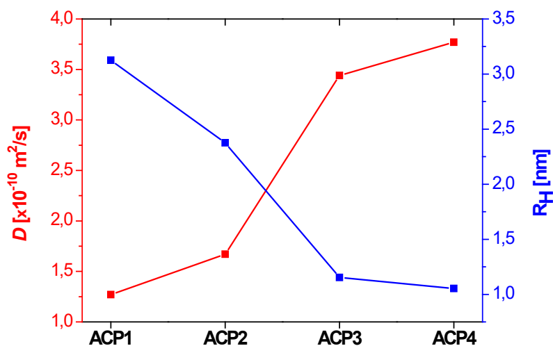
Figura 2.5 Correlación entre D y R_H para el componente-I de las sub-fracciones de asfaltenos
