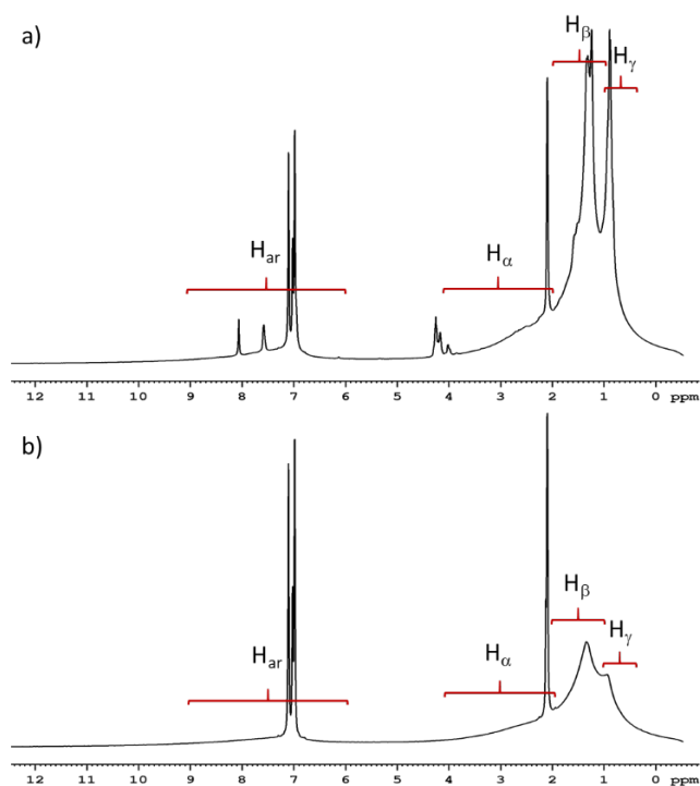
Figura 1.5 Espectro de protones ( ^1\text{H} -NMR) de los asfaltenos: a) ACP y b) ARV
