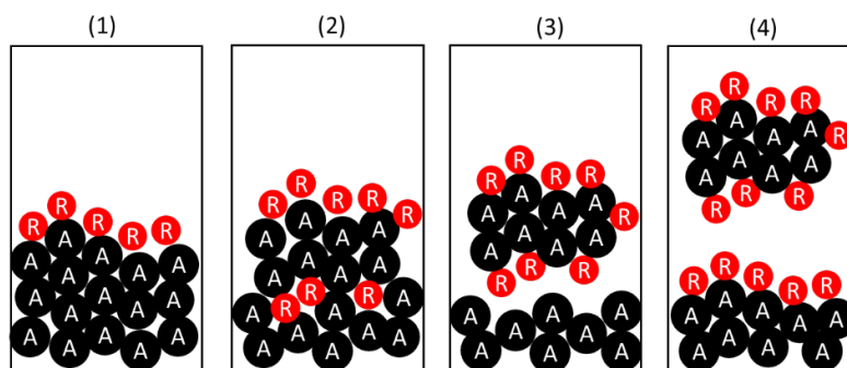
Figura 3.15 Representación del modelo de agregación propuesto para los asfaltenos en tolueno en presencia de resinas
