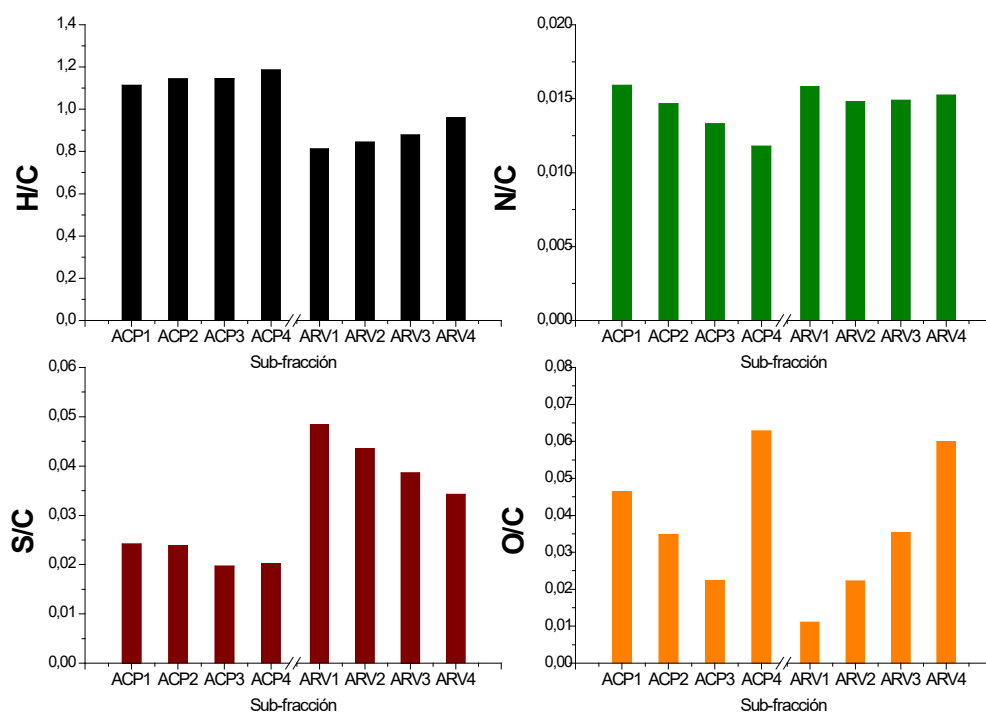
Figura 1.3 Composición elemental de las sub-fracciones de asfaltos
