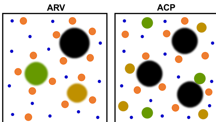
Figura 3.10 Representación hipotética del estado coloidal de los asfaltenos no fraccionados: ARV1/ACP1 en negro, ARV2/ACP2 en verde, ARV3/ACP3 en amarillo, ARV4/ACP4 en naranja. Los puntos azules representan el solvente (tolueno).
