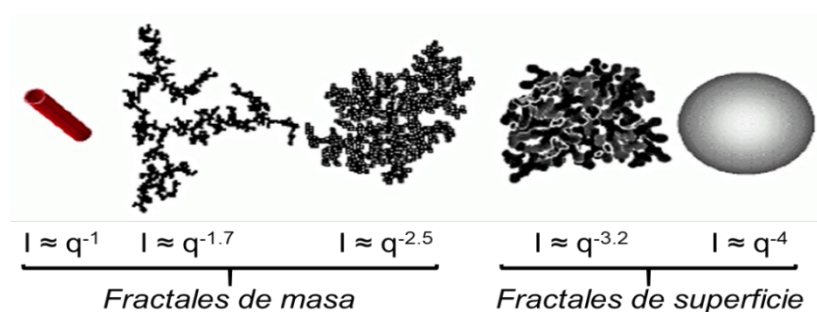
Figura 3.8 Representación de la estructura fractal de los agregados
