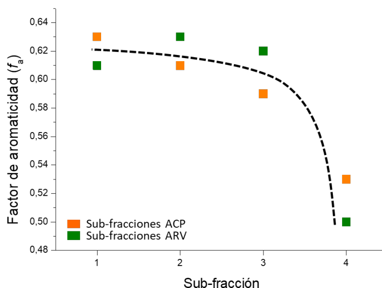
Figura 1.8 Tendencias del factor de aromaticidad f_a para las sub-fracciones
