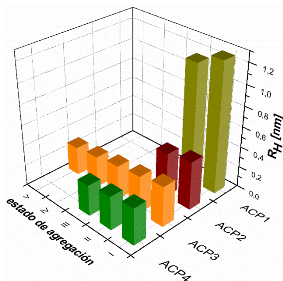
Figura 2.9 Distribución del radio hidrodinámico de las sub-fracciones en tolueno (1% p/v, 50°C)
