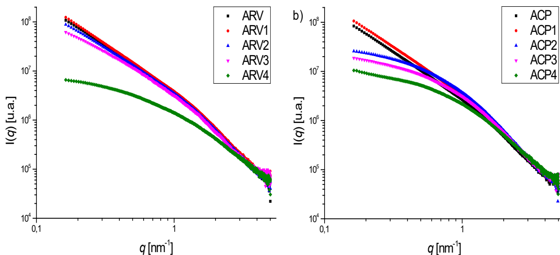
Figura 3.7 Espectros SAXS de los asfaltenos y las sub-fracciones en tolueno (1% p/v) medidos a 25 °C y 1 semana de tiempo de envejecimiento
