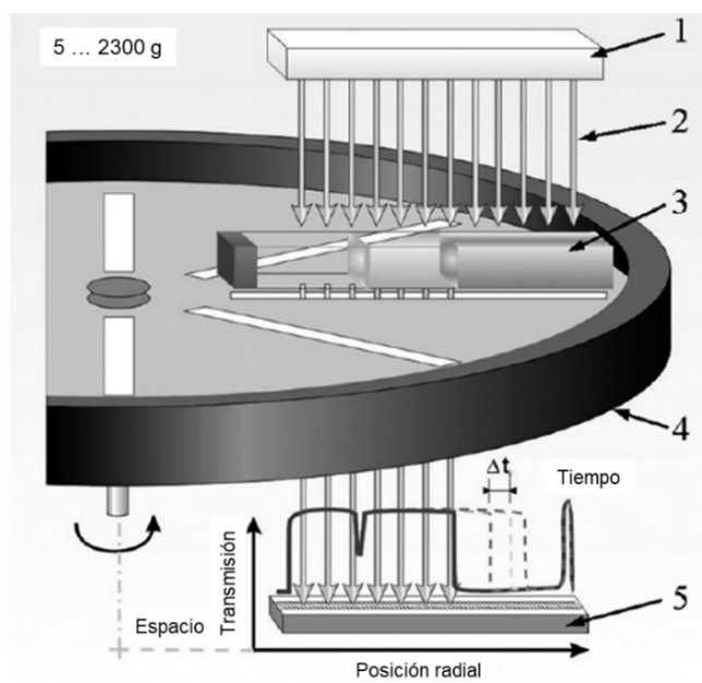
Figura 4.1 Esquema de medición de la fotocentrífuga analítica LUMiSizer. Adaptado de Detloff et al., (2007).
