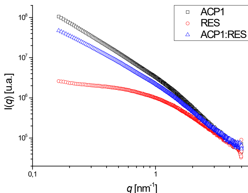
Figura 3.14 Comparación de los espectros SAXS de los sistemas ACP1 (negro), RES (rojo) y ACP1:RES (azul) en tolueno medidos a 25 °C y 1 semana de envejecimiento
