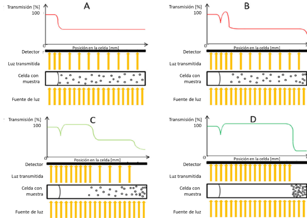
Figura 4.2 Evolución del perfil de transmisión durante la medición. Adaptado de Knoth y Keck, (2018)
