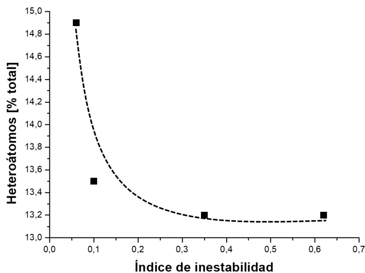
Figura 4.8 Correlación entre el índice de inestabilidad y el contenido de heteroátomos de las sub-fracciones
