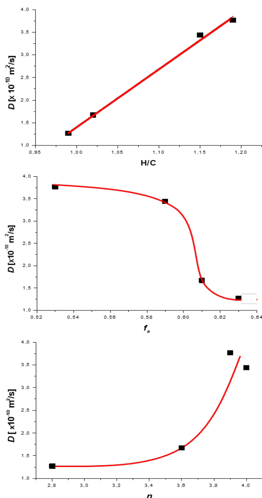
Figura 2.6 Correlación de los parámetros moleculares promedio y los coeficientes de difusión de las sub-fracciones
