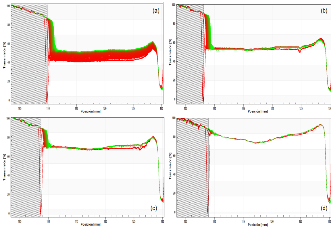
Figura 4.5 Perfiles de transmisión de las sub-fracciones de asfaltenos en tolueno obtenidos por fotocentrifugación: (a) ARV1, (b) ARV2, (c) ARV3 y (d) ARV4
