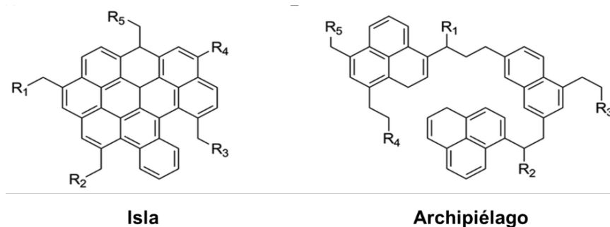
Figura 1.1 Ejemplos de estructuras isla y archipiélago de los asfaltenos. Adaptado de Santos et al. (2016)
