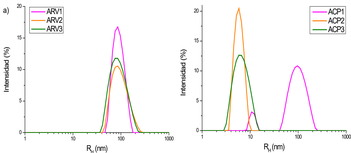
Figura 3.6 Distribución de tamaño de partícula de las sub-fracciones ARV (a) y ACP (b) en tolueno (0.1% p/v) a 25 °C y 30 min de tiempo de envejecimiento
