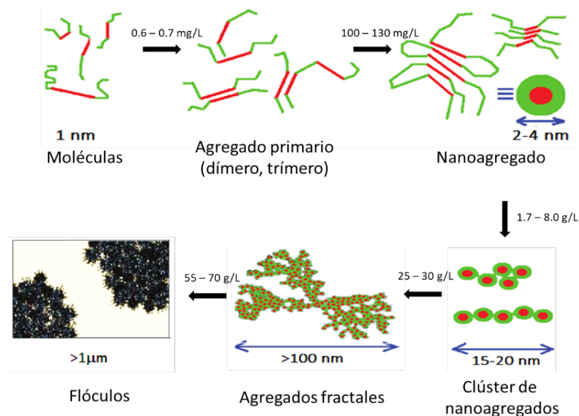
Figura 3.3 Estados de agregación propuestos para los asfaltenos en solución en función de la concentración
