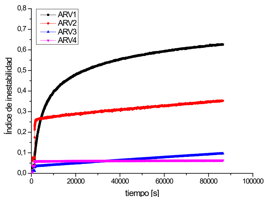
Figura 4.6 Perfiles de estabilidad de las sub-fracciones en términos del índice de inestabilidad en función del tiempo
