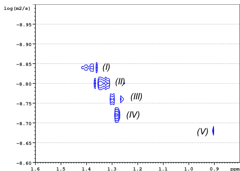
Figura 2.8 Espectro ^1\text{H} DOSY NMR de la sub-fracción ACP3 en tolueno (1% p/v) a 50 °C
