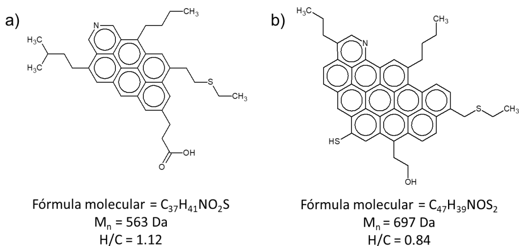
Figura 1.7 Modelos propuestos para representar las estructuras promedio de los asfaltenos: a) ACP y b) ARV
