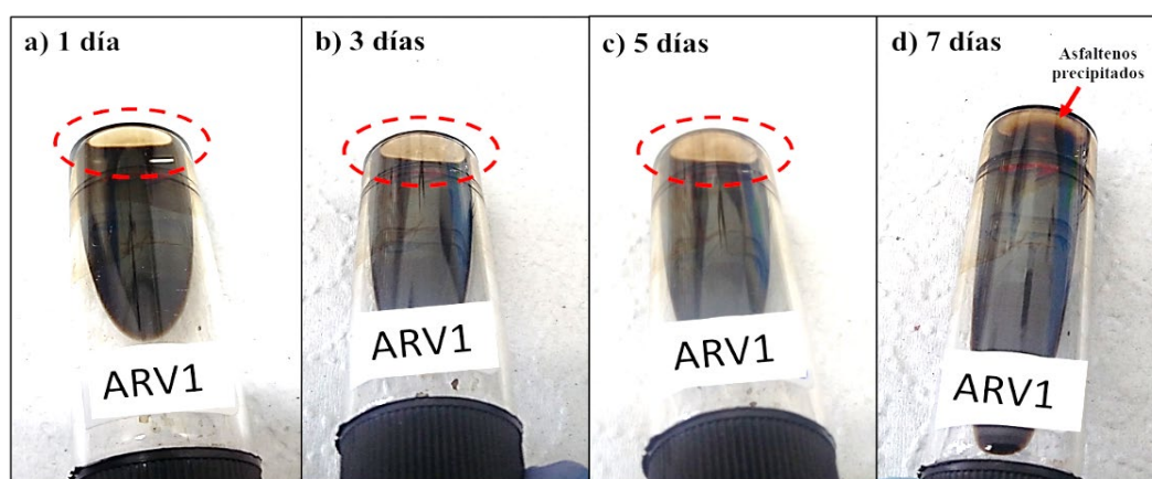
Figura 4.4 Progreso de la precipitación de los asfaltenos de la sub-fracción ARV1 a condiciones ambiente en función del tiempo
