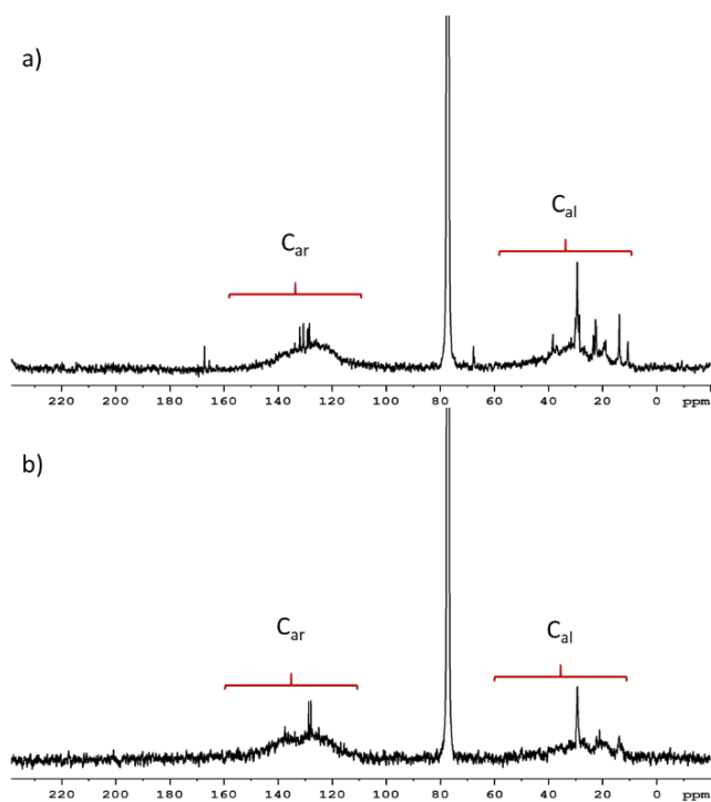
Figura 1.6 Espectro de carbonos ( ^{13}\text{C} -NMR) de los asfaltenos: a) ACP y b) ARV
