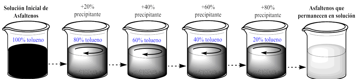
Figura 1.2. Representación del método de separación de los asfaltenos en sub-fracciones por precipitación secuencial en mezclas tolueno/acetona.
