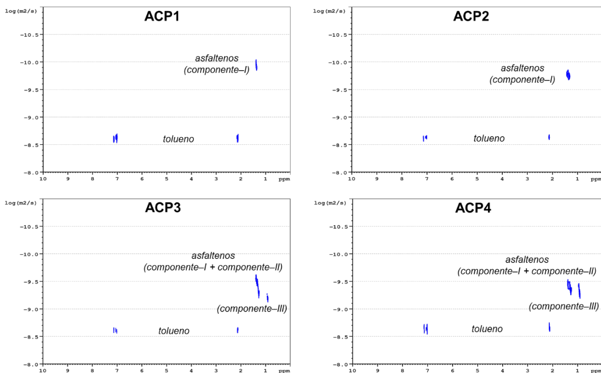
Figura 2.4 Espectros 1 H DOSY NMR de soluciones al 1% p/v de las sub-fracciones de asfaltenos en tolueno-d 8 medidos a 25 °C
