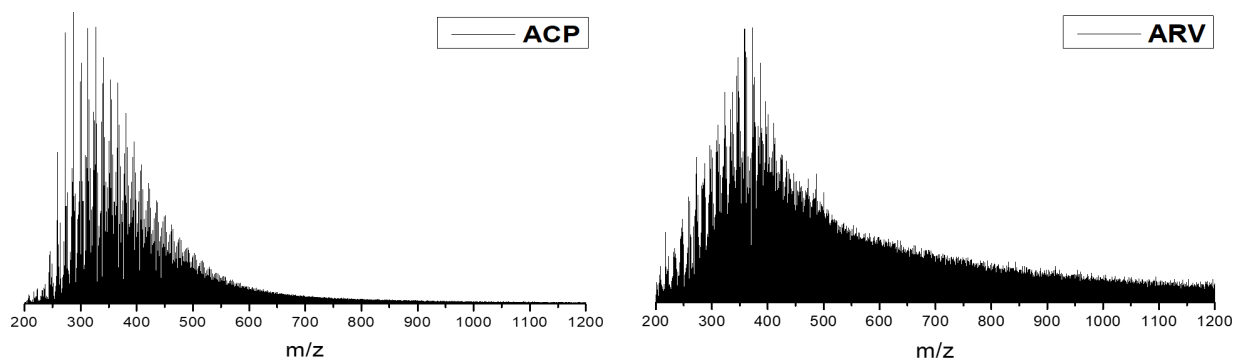
Figura 1.4. Distribuciones de peso molecular de los asfaltenos no fraccionados
