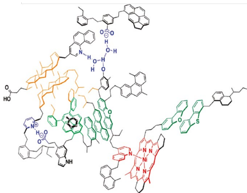
Figura 2.1 Modelo de agregación de asfaltenos propuesto por Gray et al. (2011)
