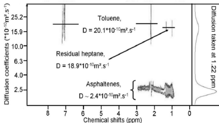
Figura 2.2 Espectro ^1\text{H} DOSY NMR de los asfaltenos en tolueno. Adaptado de Durand et al., (2008)
