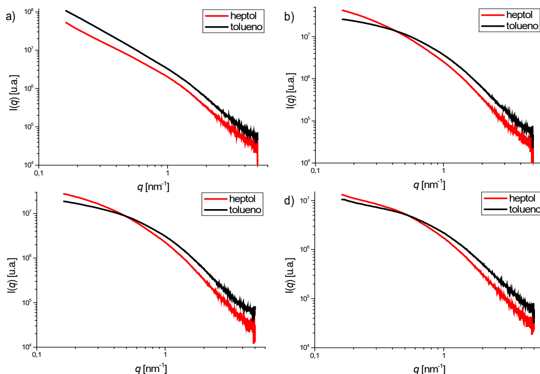
Figura 3.12 Comparación de los espectros SAXS de las sub-fracciones ACP en tolueno (línea negra) y en heptol (línea roja) medidos a 25 °C
