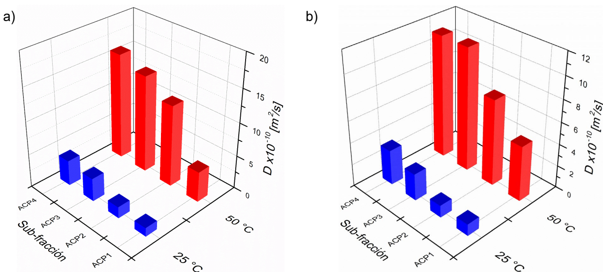
Figura 2.7 Efecto de la temperatura sobre el coeficiente de difusión del componente-I para las sub-fracciones en tolueno: (a) 1% p/v y (b) 5% p/v
