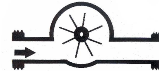
Figura 2. Esquema de flujo de chorro único y turbina de paleta simple. Fuente [18]
