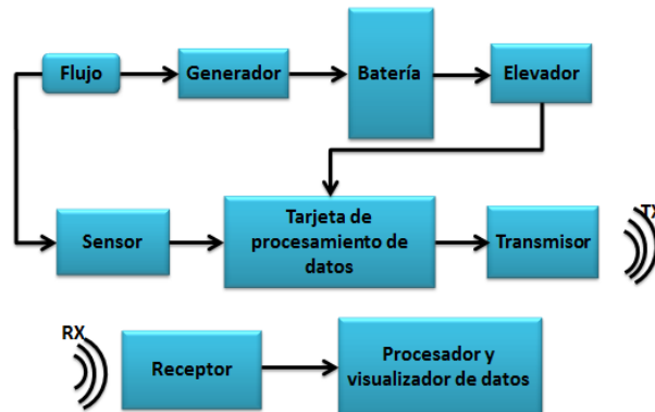
Figura 1. Diagrama de bloques de procesos del medidor
