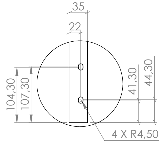
DETALLE M ESCALA 2 : 9
