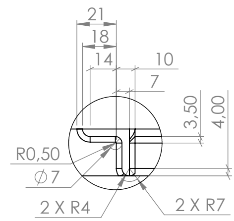
DETALLE U ESCALA 1 : 2
