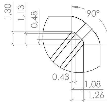
DETALLE S ESCALA 5 : 1
