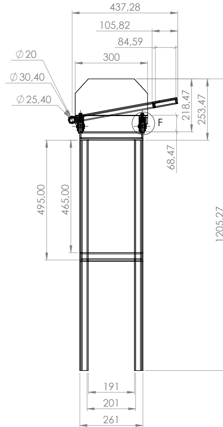
SECCIÓN C-C ESCALA 1 : 9
