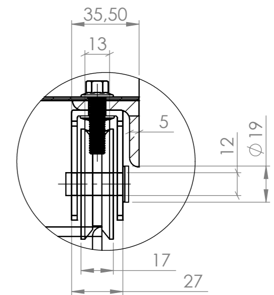
DETALLE F ESCALA 1 : 2
