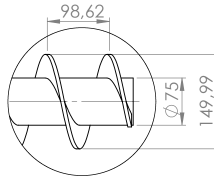
DETALLE L ESCALA 1 : 6
