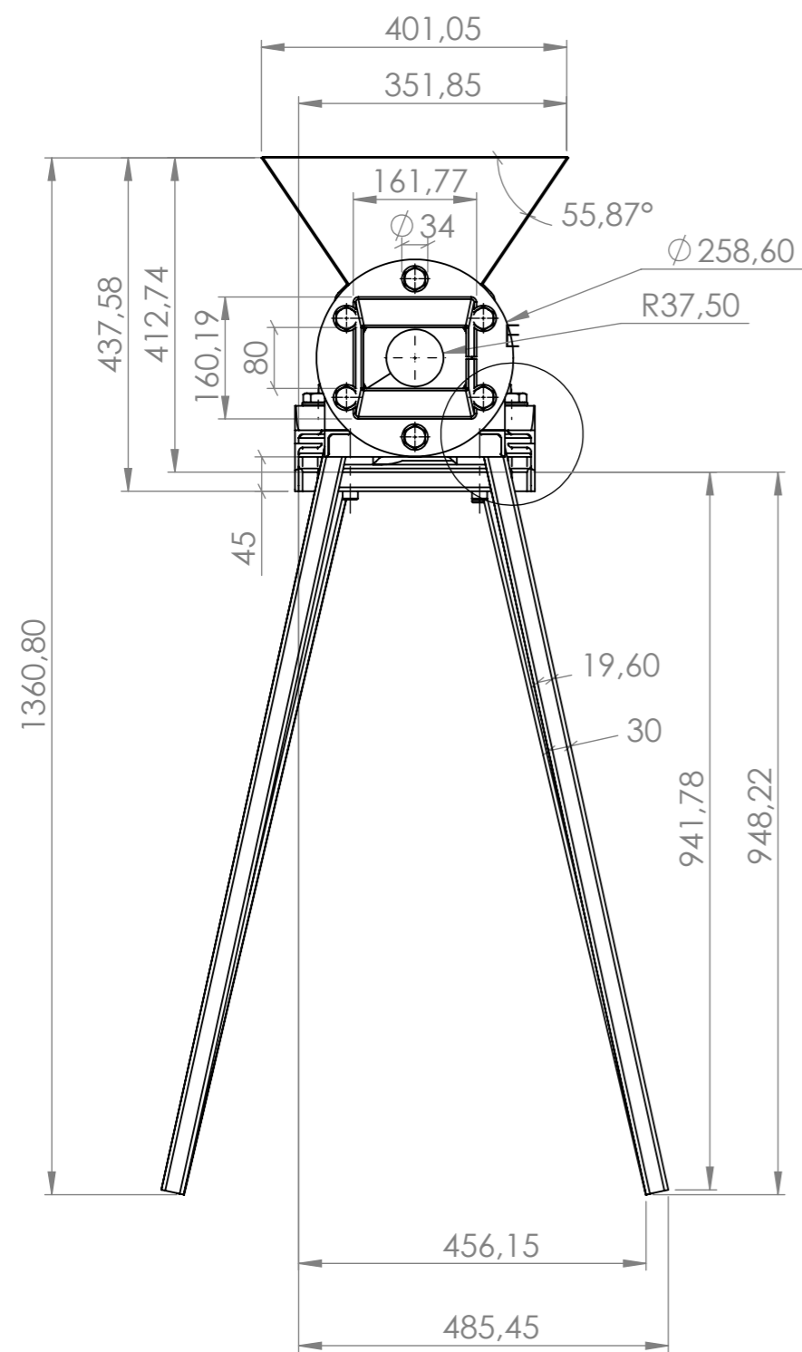
SECCIÓN B-B ESCALA 1 : 9
