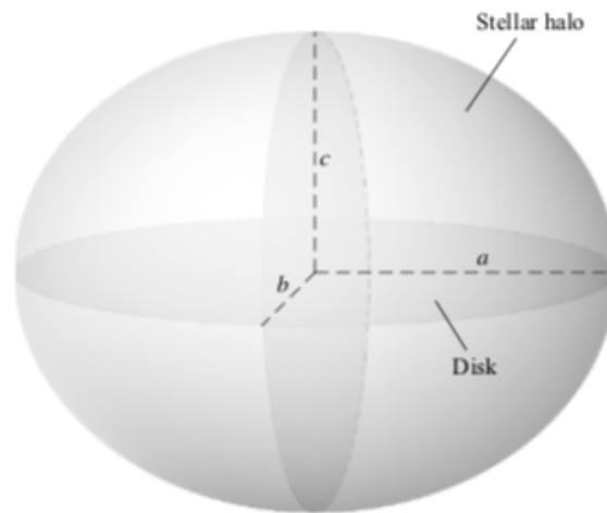
Figura 3. La forma general de un sistema esferoidal triaxial, donde se supone que tienen los tres ejes del esferoide. El disco galáctico es aproximadamente circular Carroll and Ostlie (2007).
