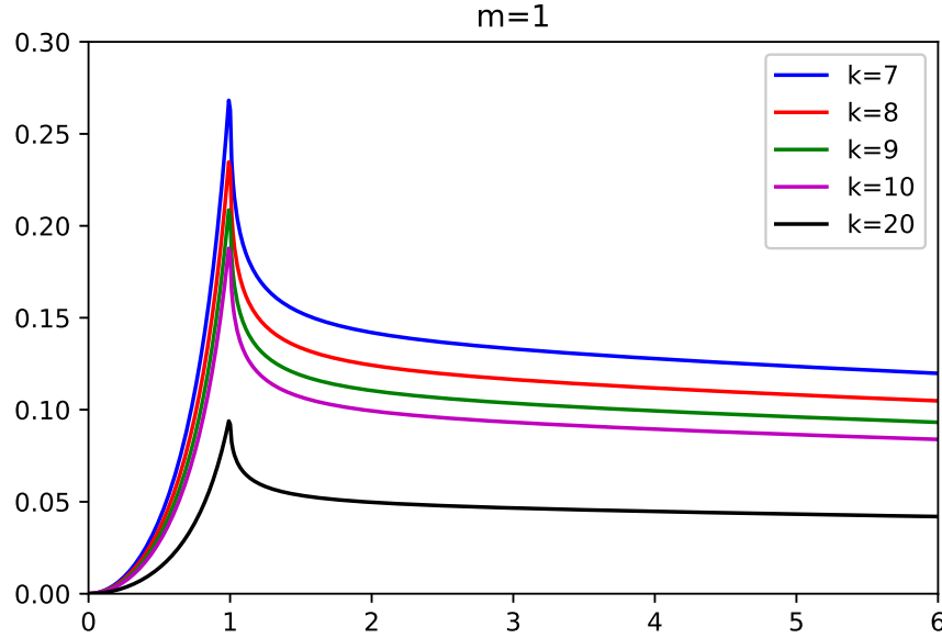
Figura 22. curvas de rotación v_1^2 en función de R/a , para el primer modelo de la familia de soluciones. Estas curvas de rotación se obtienen con los mismos parámetros de la figura 5-1.
