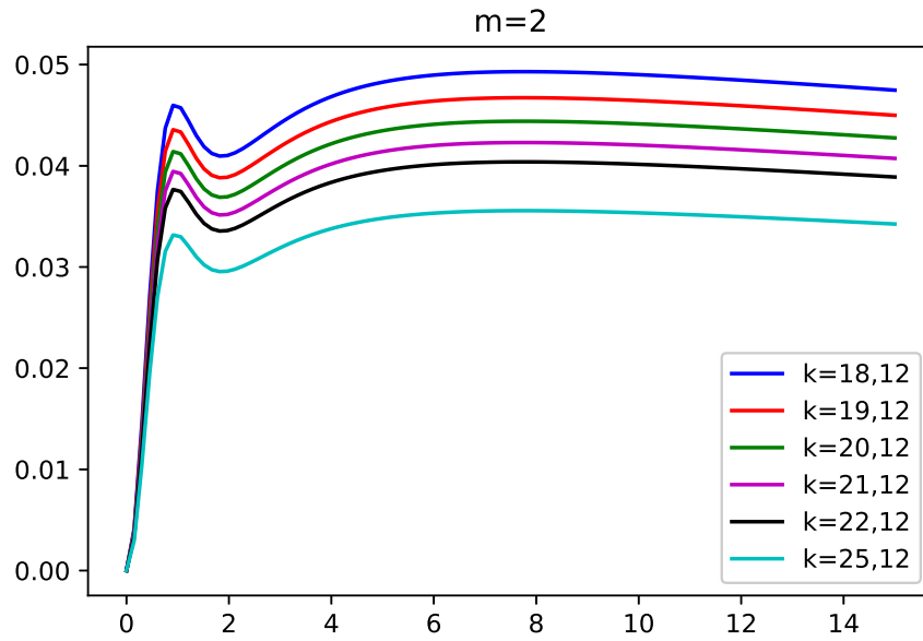
Figura 16. curvas de rotación v_2^2 en función de R/a , para el segundo modelo de la familia de soluciones.
