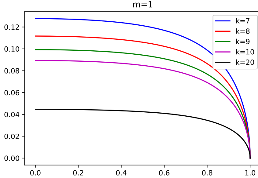
Figura 20. Densidad de masa superficial del disco \tilde{\sigma}_1 en función de R/a para el modelo m = 1 de la familia de soluciones.
