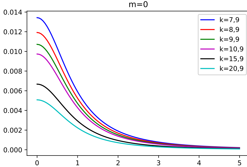
Figura 6. Densidad de masa superficial del disco \tilde{\sigma}_0 en función de R/a para el modelo m = 0 de la familia de soluciones.
