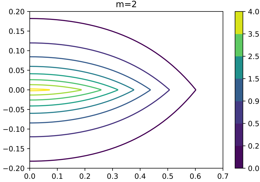
Figura 15. Densidad de masa del halo \rho_2 en función de R/a y z/a para el modelo m = 2 de la familia de soluciones.
