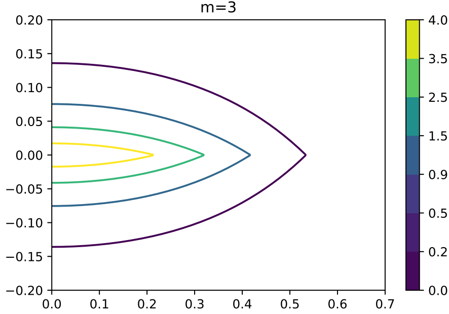
Figura 27. Contorno de densidad de masa del halo en función de R/a (eje horizontal) y z/a (eje vertical). Los contornos corresponden al modelo m = 3 , con las constantes \tilde{C}_0 = 2 , \tilde{C}_2 = 5/3 , \tilde{C}_4 = 9/11 , \tilde{C}_4 = 5/33 y k = 17 .
