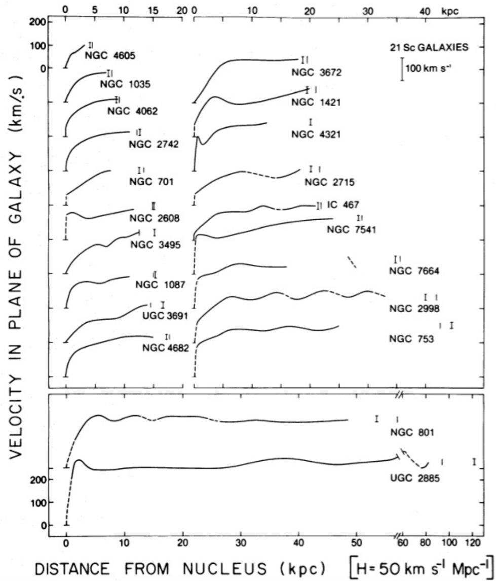
Figura 2. Curvas de rotación para una muestra de 21 galaxias espirales. Imagen tomada de ?.
