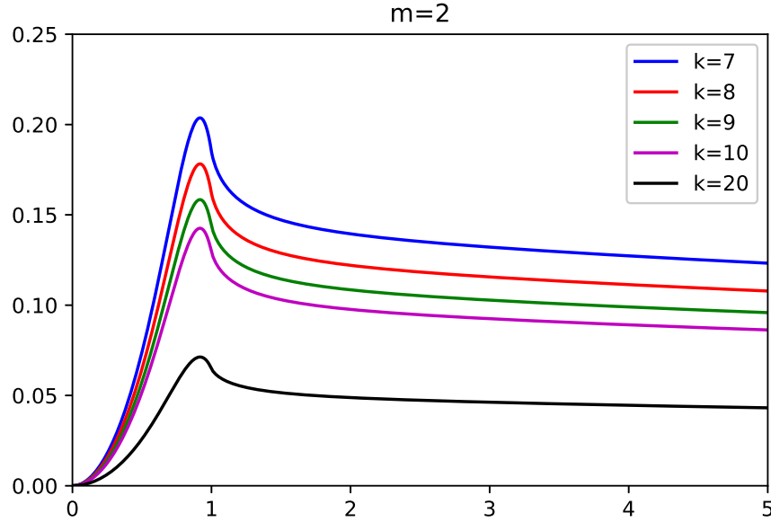
Figura 25. curvas de rotación v_2^2 en función de R/a , para el primer modelo de la familia de soluciones. Estas curvas de rotación se obtienen con los mismos parámetros de la figura 5-4.
