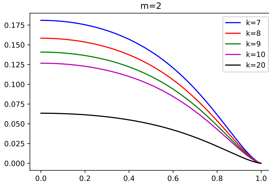
Figura 23. Densidad de masa superficial del disco \tilde{\sigma}_2 en función de R/a para el modelo m = 2 de la familia de soluciones.
