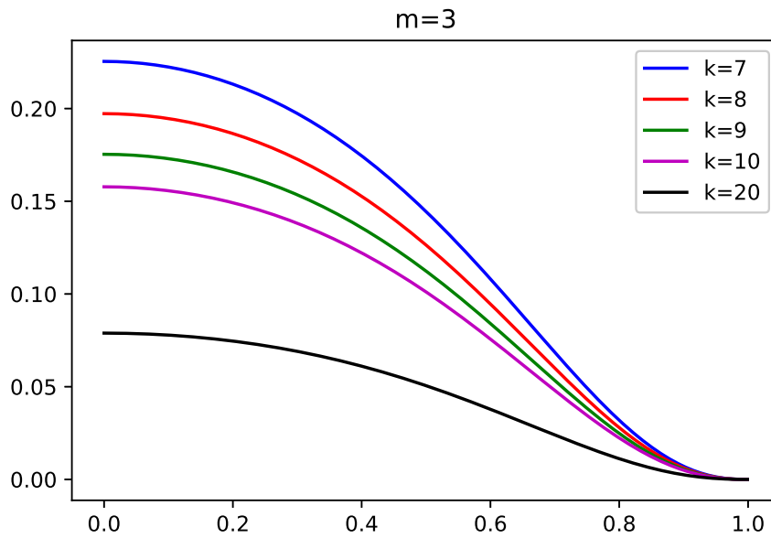
Figura 26. Densidad de masa superficial del disco \tilde{\sigma}_3 en función de R/a para el modelo m = 3 de la familia de soluciones.
