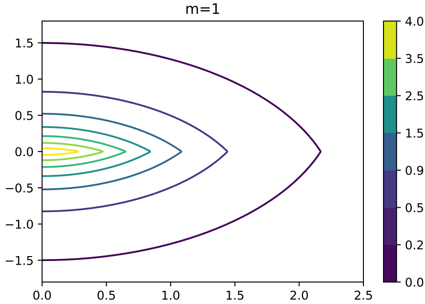
Figura 12. Densidad de masa del halo \tilde{\rho}_1 en función de R/a y z/a para el modelo m = 1 de la familia de soluciones.
