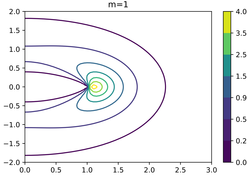
Figura 21. Contorno de densidad de masa del halo en función de R/a (eje horizontal) y z/a (eje vertical). Los contornos corresponden al modelo m = 1 , con las constantes \tilde{C}_0 = 1 , \tilde{C}_2 = 1 y k = 20 .
