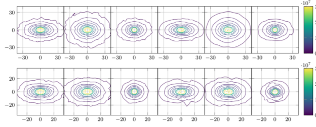
Figura 8. De izquierda a derecha: contornos de densidad en los tres planos principales del halo numérico original, luego contornos de densidad en los mismos tres planos principales del halo reconstruidos con funciones básicas hasta n = 20 y l = 12 Lilley et al. (2018b).
