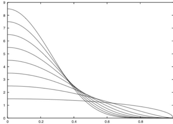
Figura 11. Densidad de superficie \sigma_m en función de \tilde{R} para modelos de discos de Kalnajs generalizados con m = 1 (curva inferior) hasta m = 8 (curva superior). González and Reina (2006).
