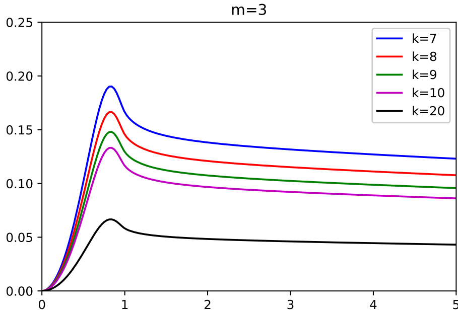
Figura 28. curvas de rotación v_3^2 en función de R/a , para el primer modelo de la familia de soluciones. Estas curvas de rotación se obtienen con los mismos parámetros de la figura
