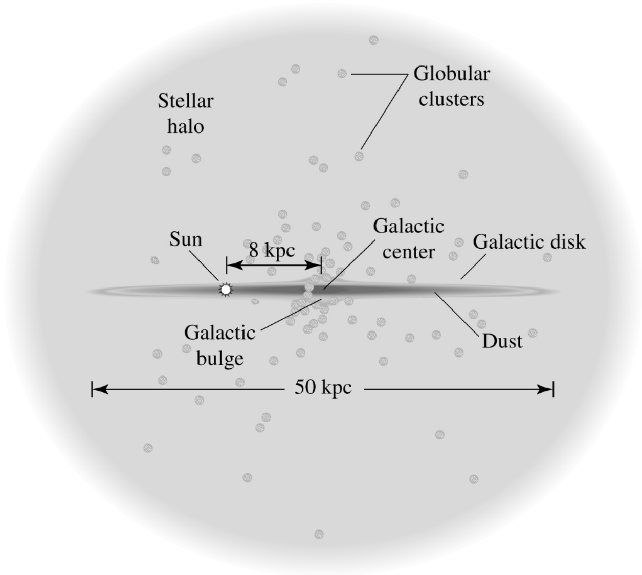
Figura 1. Componentes de una galaxia espiral Carroll and Ostlie (2007). Es importante notar que esta imagen no se encuentra a escala.
