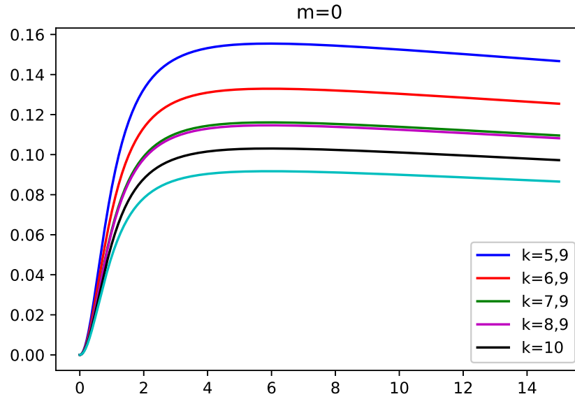
Figura 9. Dcurvas de rotación v_0^2 en función de R/a , para el primer modelo de la familia de soluciones. Estas curvas de rotación se obtienen con los mismos parámetros de la figura 4-1.
