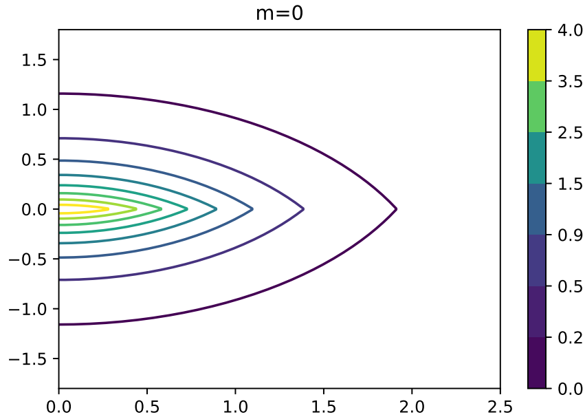
Figura 7. Contorno de densidad de masa del halo en función de R/a (eje horizontal) y z/a (eje vertical). Los contornos corresponden al modelo m = 0 , con las constantes \tilde{C}_0 = 2 y k = 7.9 .
