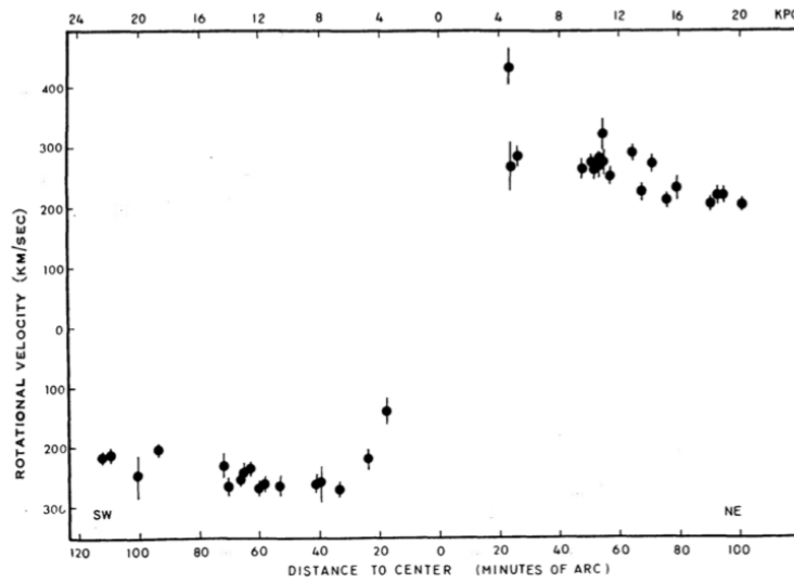
Figura 18. Curvas de rotación medias para treinta y cuatro asociaciones OB más tres regiones externas en M31, en función de la distancia desde el centro. Las barras de error indican el error promedio de la velocidad de la asociación, calculado a partir de las velocidades de las regiones de emisión individuales en la asociación, o de los errores de observación, cualquiera que sea mayor Rubin and Ford (1970).
