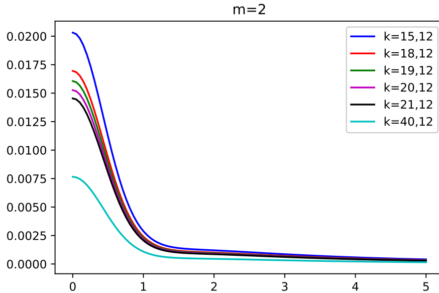
Figura 14. Densidad de masa superficial del disco \tilde{\sigma}_2 en función de R/a para el modelo m = 2 de la familia de soluciones.
