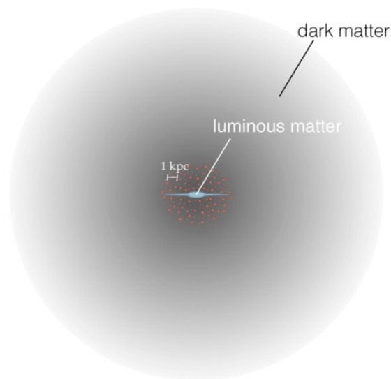
Figura 4. extensión del halo de materia oscura Carroll and Ostlie (2007).
