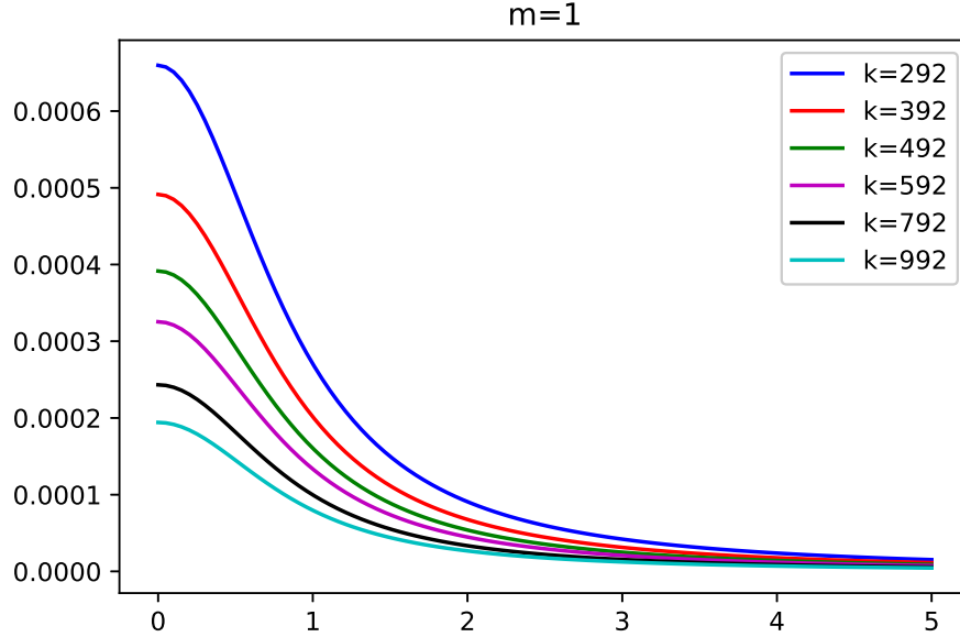
Figura 10. Densidad de masa superficial del disco \tilde{\sigma}_1 en función de R/a para el modelo m = 1 de la familia de soluciones.
