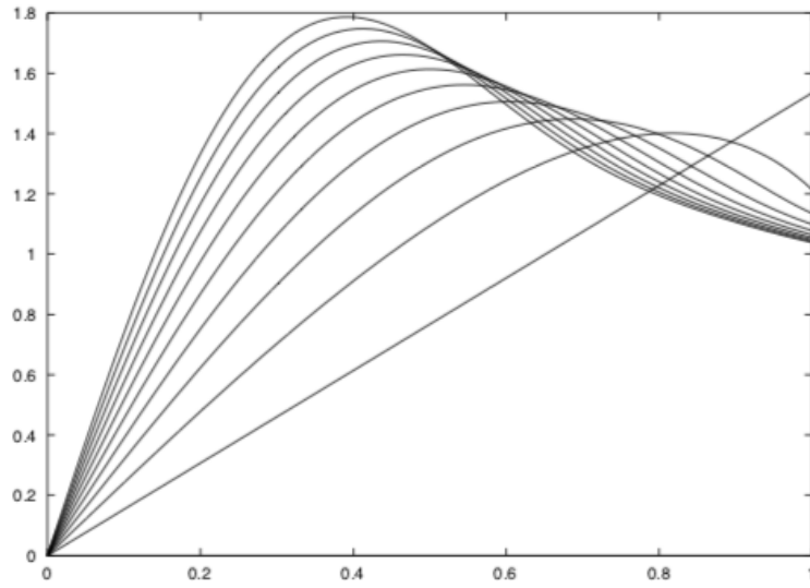
Figura 17. Curvas de rotación v_m como funciones de \tilde{R} para modelos de discos de Kalnajs generalizados con m = 1 (línea derecha) hasta m = 10 (curva superior) González and Reina (2006).
