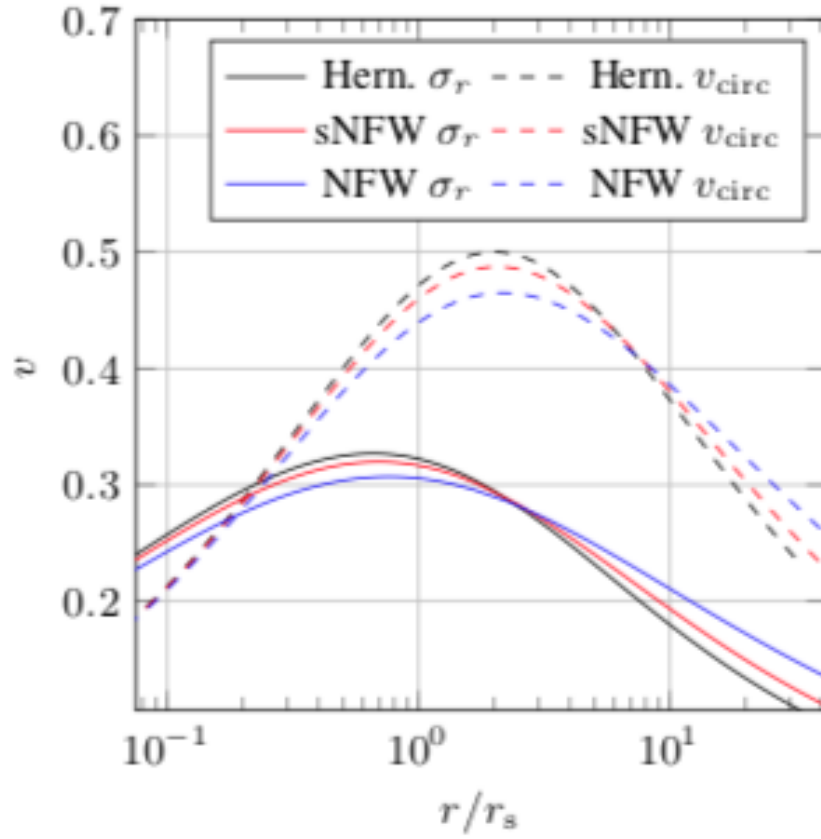
Figura 19. La dispersión de velocidad (completa) y la curva de rotación (punteada) del modelo sNFW (rojo) en comparación con los modelos Hernquist (negro) y NFW (azul) trazados contra el radio (en unidades de r_s ). Tenga en cuenta que los picos de la curva de rotación y la dispersión de la velocidad de los modelos son comparables, pero la disminución para el modelo de Hernquist se produce más rápidamente que para los modelos sNFW y NFW Lilley et al. (2018a).
