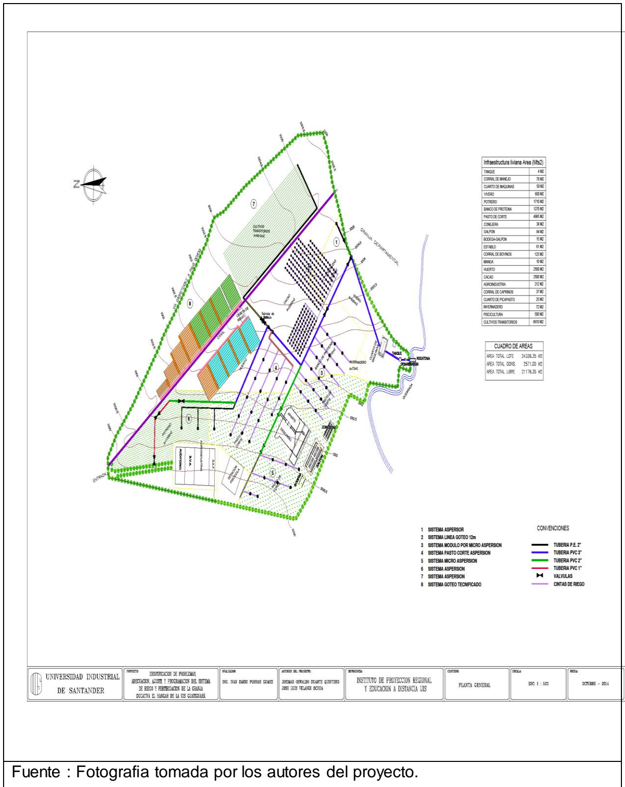
Imagen 18. Plano final sistema de riego granja educativa El Hangar
