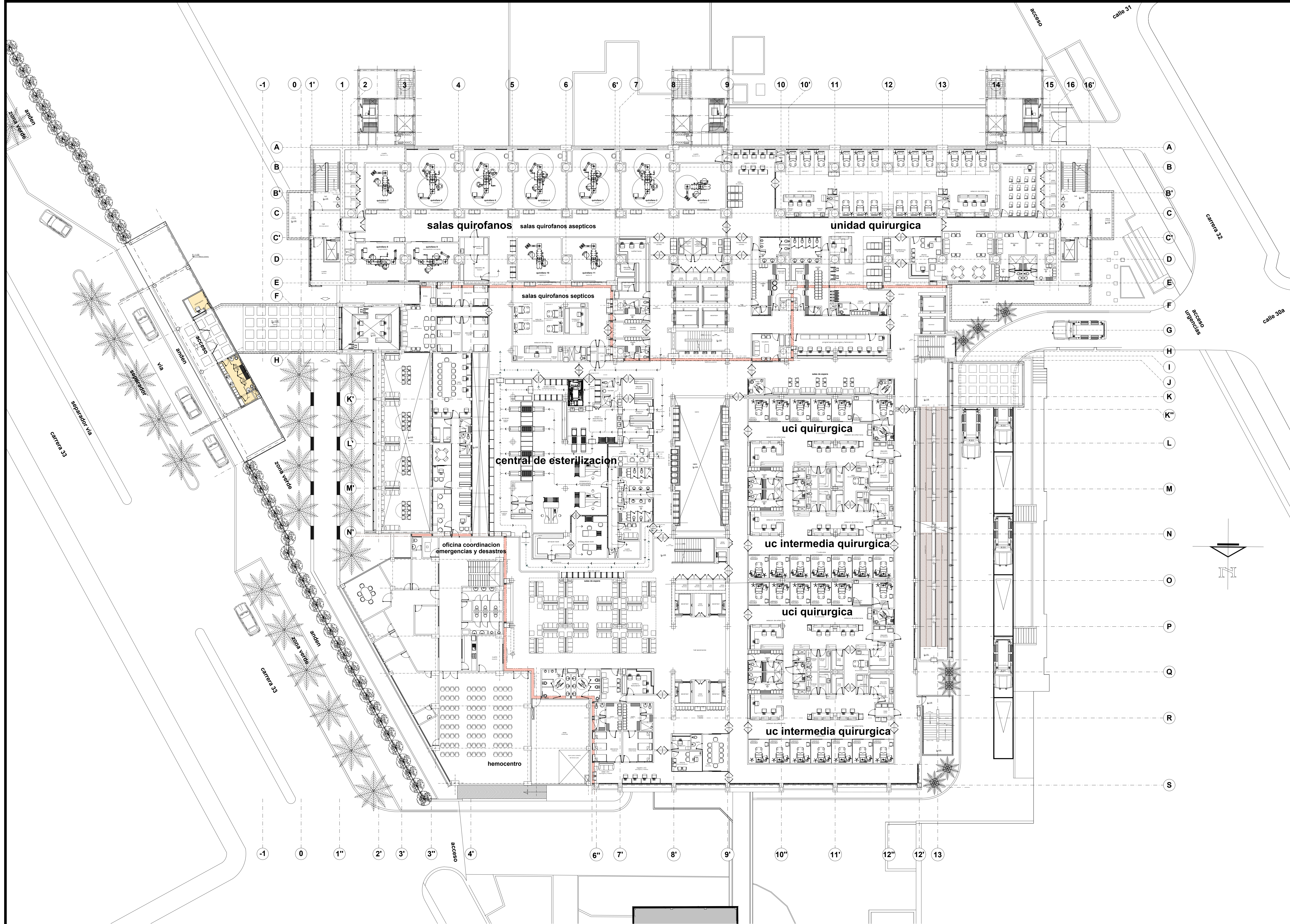
tercer piso torre plataforma esc. 1:200
