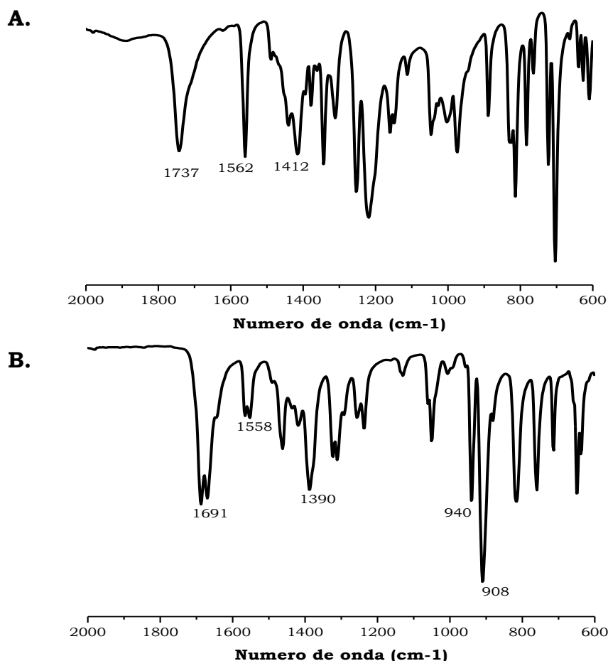
Figura 12. Espectro IR (KBr) de A. ácido bis-(3,5-dimetil-pirazol-1-il)-acético ( 1 ) y B. MoO 2 Cl-bis-(3,5-dimetil-pirazol-1-il)-acetato ( 7 ).
