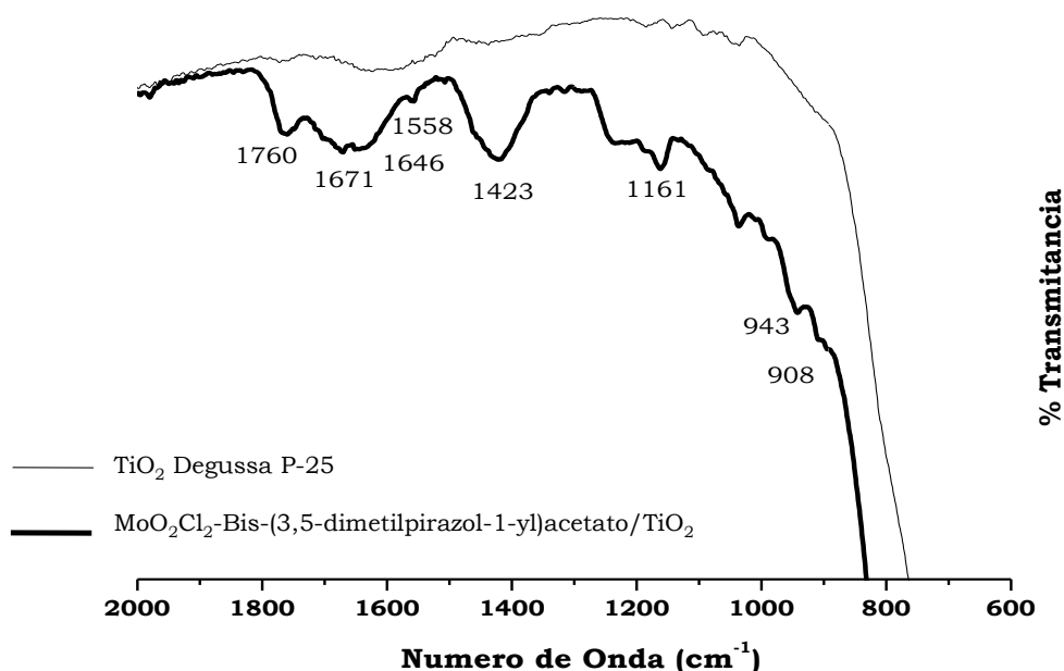
Figura 29. Espectro IR (KBr) del sistema MoO 2 Cl 2 -Bis-(3,5-dimetilpirazol-1-il) acetato anclado sobre TiO 2 .
