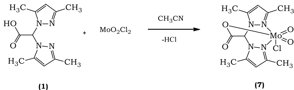
Esquema 17. Reacción entre el ácido bis-3,5-dimetilpirazolil acético ( 1 ) y \text{MoO}_2\text{Cl}_2 .
