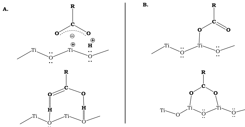
Figura 18. Tipos de enlace para el grupo carboxilato sobre la superficie del \text{TiO}_2 .
