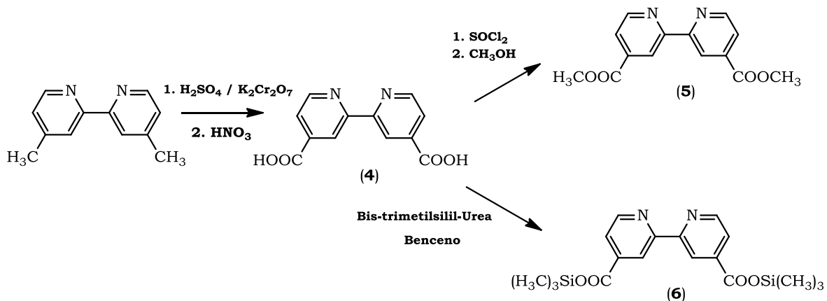
Esquema 14. Procedimiento empleado para la síntesis de bipyridinas disustituidas: 4,4'-dicarboxi-2,2'-bipyridina (4), 4,4'-dicarbometoxi-2,2'-bipyridina (5) y 4,4'-dicarboxitrimetilsilil-2,2'-bipyridina (6).
