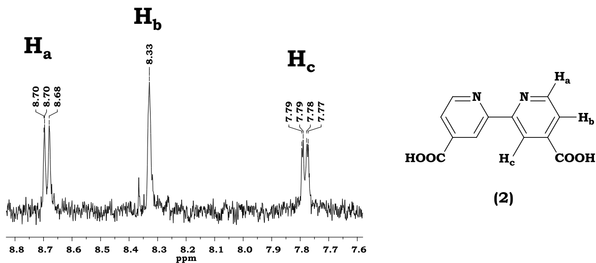
Figura 9. Espectro RMN ^1\text{H} de 4,4'-dicarboxi-2,2'-bipiridina (2) en \text{CD}_3\text{OD} .
