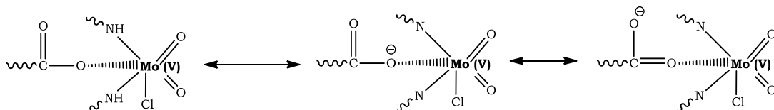
Esquema 28. Posibles estructuras propuestas que favorecen la reversibilidad de la unidad Mo(VI) a Mo(V) en el complejo (7).
