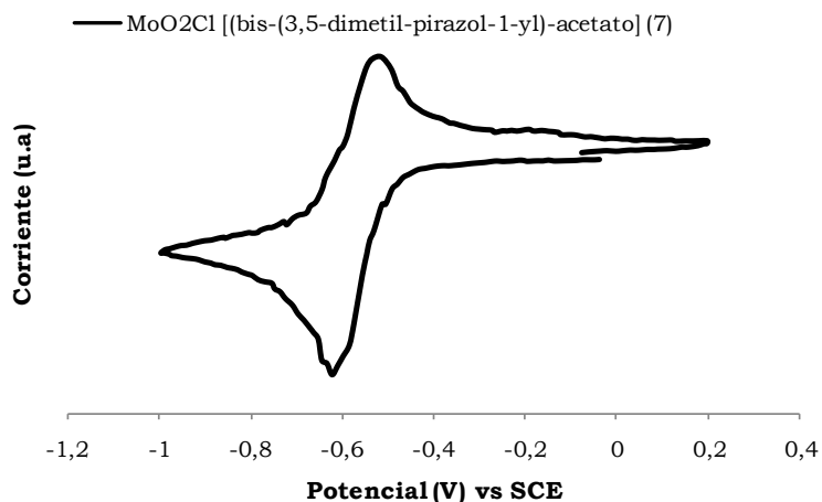
Figure 37. Voltamograma Cíclico para el complejo MoO 2 Cl-bis-(3,5-dimetil-pirazol-1-il)-acetato ( 7 ) en acetonitrilo.
