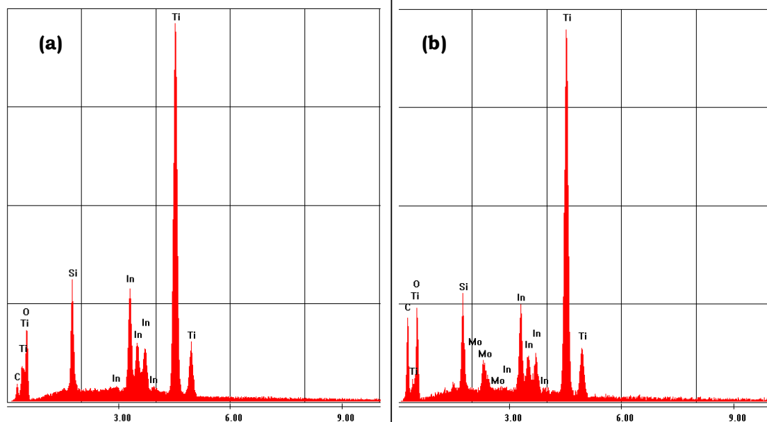
Figure 41. Análisis por espectroscopía EDX para los electrodos de ITO. a) \text{TiO}_2/\text{ITO} y b) \text{Mo-TiO}_2/\text{ITO} .
