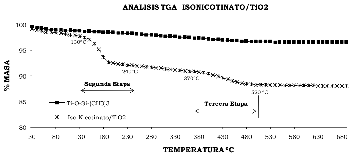
Figura 21. Perfil termogravimétrico obtenido para el sistema Ti-O-Si-(CH 3 ) 3 (-■-) y el isonicotinato/TiO 2 (-*-) en el rango de temperaturas entre 30 y 700°C.
