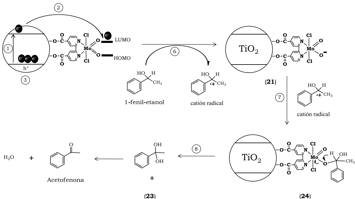
Esquema 43. Obtención de acetofenona a partir de 1-fenil-etanol por un proceso fotoinducido.
