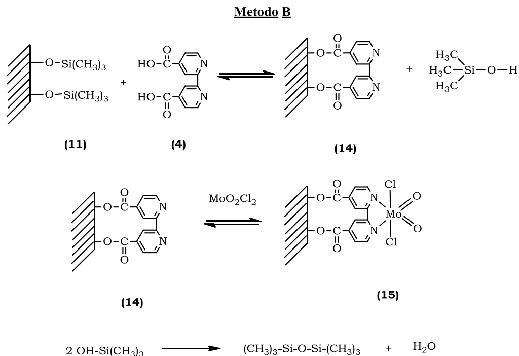
Esquema 24. Anclaje covalente por el método B del Complejo \text{MoO}_2\text{Cl}_2 -2,2'-bipiridin-4,4'-dicarboxilato en \text{TiO}_2 .
