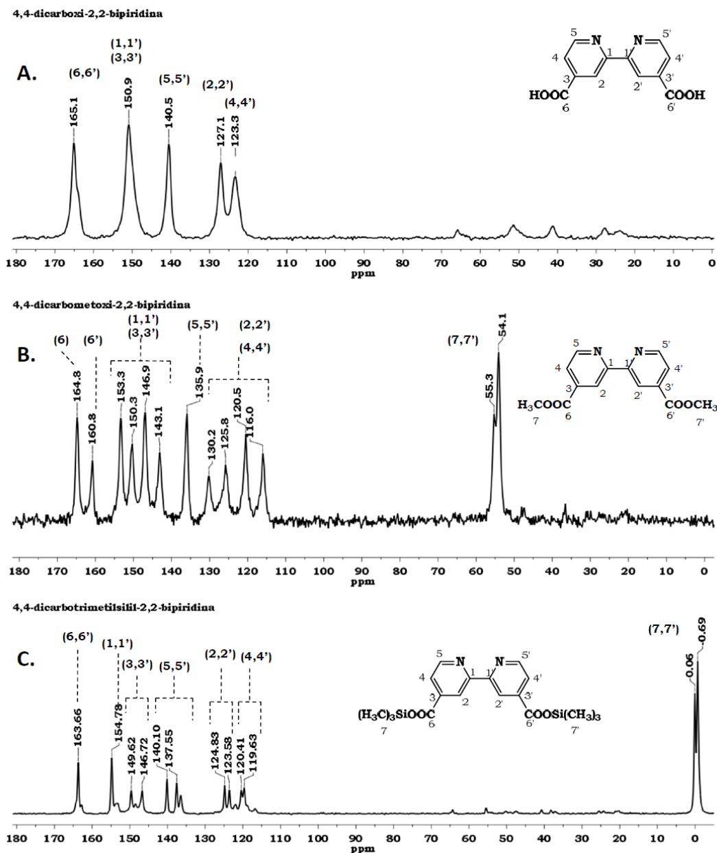
Figura 10. Espectros RMN- ^{13}\text{C} CP-MAS de los ligandos 4,4'-dicarboxi-2,2'-bipiridina ( 4 ), 4,4'-dicarbometoxi-2,2'-bipiridina ( 5 ) y 4,4'-dicarboxitrimetilsilil-2,2'-bipiridina ( 6 ).
