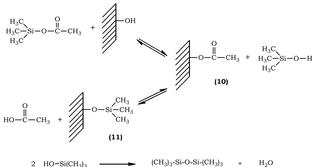
Esquema 20. Anclaje covalente de ácido acético en \text{TiO}_2 .
