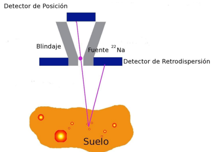
FIGURA 1: ESQUEMA DISPOSITIVO CÁMARA COMPTON.
