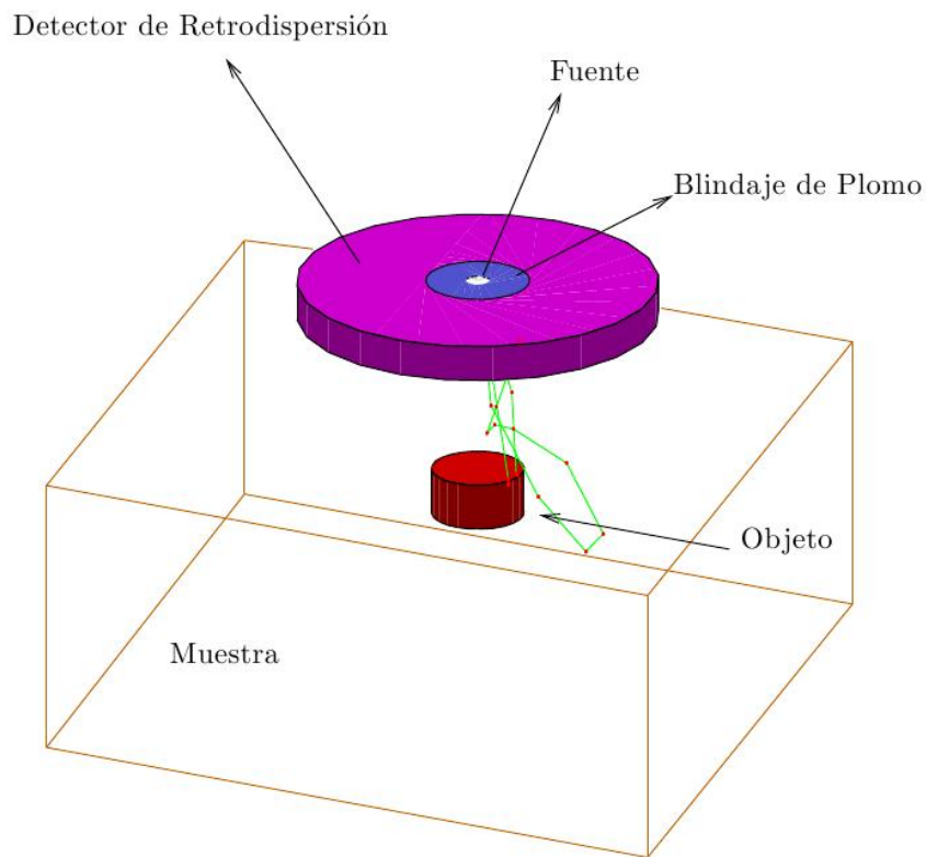
FIGURA 12: ESQUEMA DEL ARREGLO EXPERIMENTAL SIMULADO.
