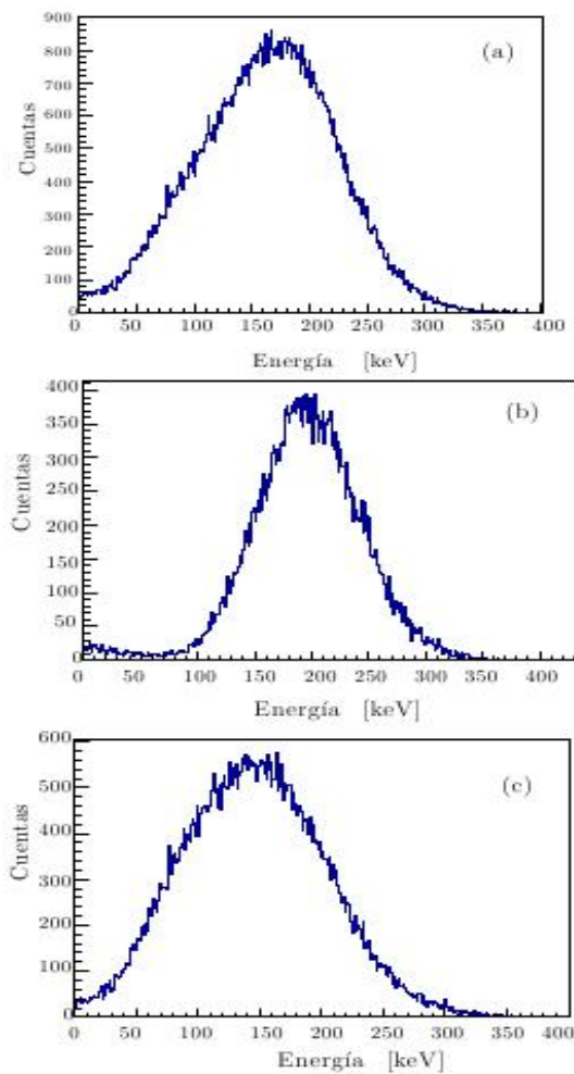
FIGURA 16: (A) ESPECTRO DE RETRODISPERSIÓN TOTAL PARA MINA EN FE INMERSA EN SUELO FRANCO, (B) ESPECTRO RETRODISPERSIONES COMPTON SIMPLES, (C) ESPECTRO RETRODISPERSIÓN COMPTON MÚLTIPLE.
