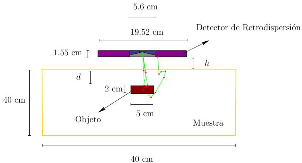
FIGURA 14: DIMENSIONES UTILIZADAS; D, DISTANCIA MUESTRA-OBJETO Y H, DISTANCIA MUESTRA-detector de retrodispersión.
