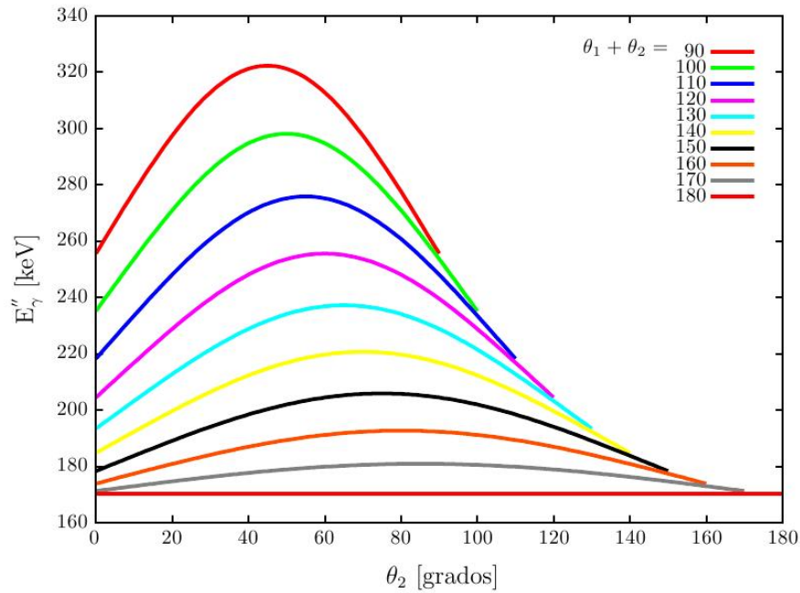
FIGURA 7: ENERGÍA DEL RAYO \Gamma QUE REALIZA DOS DISPERSIONES COMPTON ( E''_\gamma ) EN FUNCIÓN DEL ÁNGULO DE DISPERSIÓN PARA UN RAYO \Gamma INCIDENTE DE 511 KEV.
