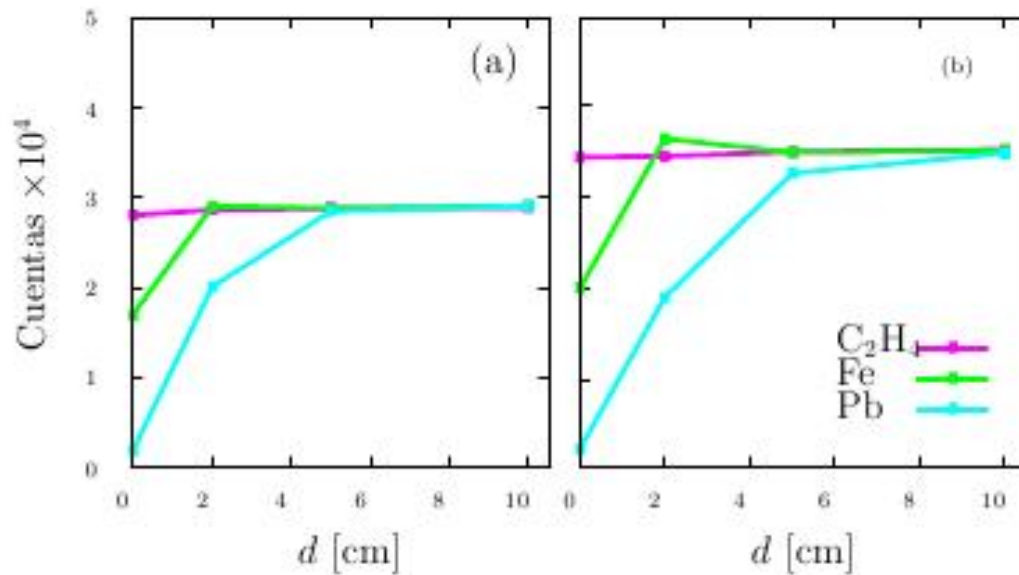
FIGURA 21: NUMERO DE RETRODISPERSIONES COMPTON SIMPLES EN A) ARENA Y B) SUELO FRANCO para los tres materiales del objeto.
