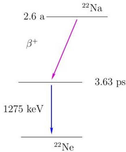
Figura 1.8: Esquema de decaimiento del ^{22}\text{Na} .
