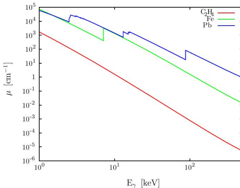
FIGURA 2: SECCIÓN EFICAZ DE ABSORCIÓN FOTOELÉCTRICA PARA EL C _2 H _4 , FE Y PB. 3
