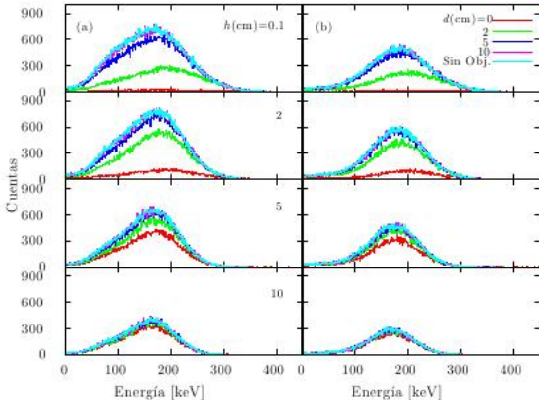
FIGURA 20 ESPECTRO DE RETRODISPERSIÓN PARA OBJETO DE PLOMO INMERSO EN: (A) ARENA Y (B) SUELO FRANCO CON LA RESPECTIVA VARIACIÓN DE LA POSICIÓN DEL DR ( h ) Y POSICIÓN DEL OBJETO ( d ).
