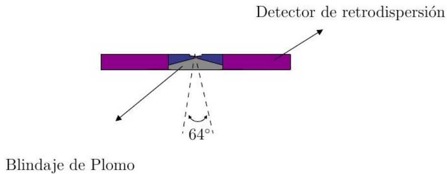
FIGURA 13: BLINDAJE DE PLOMO.
