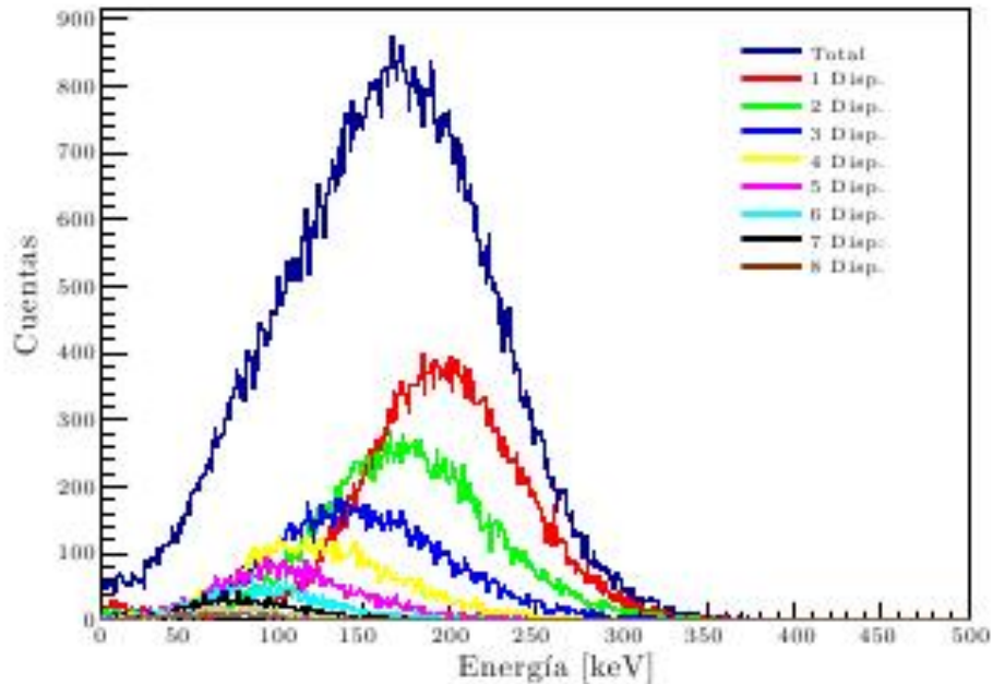
FIGURA 17: CONTRIBUCIÓN DE DISPERSIONES COMPTON SIMPLES Y MÚLTIPLES AL ESPECTRO DE RETRODISPERSIÓN DE OBJETO DE FE INMERSO EN SUELO FRANCO A UNA PROFUNDIDAD DE 2 CM Y EL DR A UNA ALTURA DE 2 CM.
