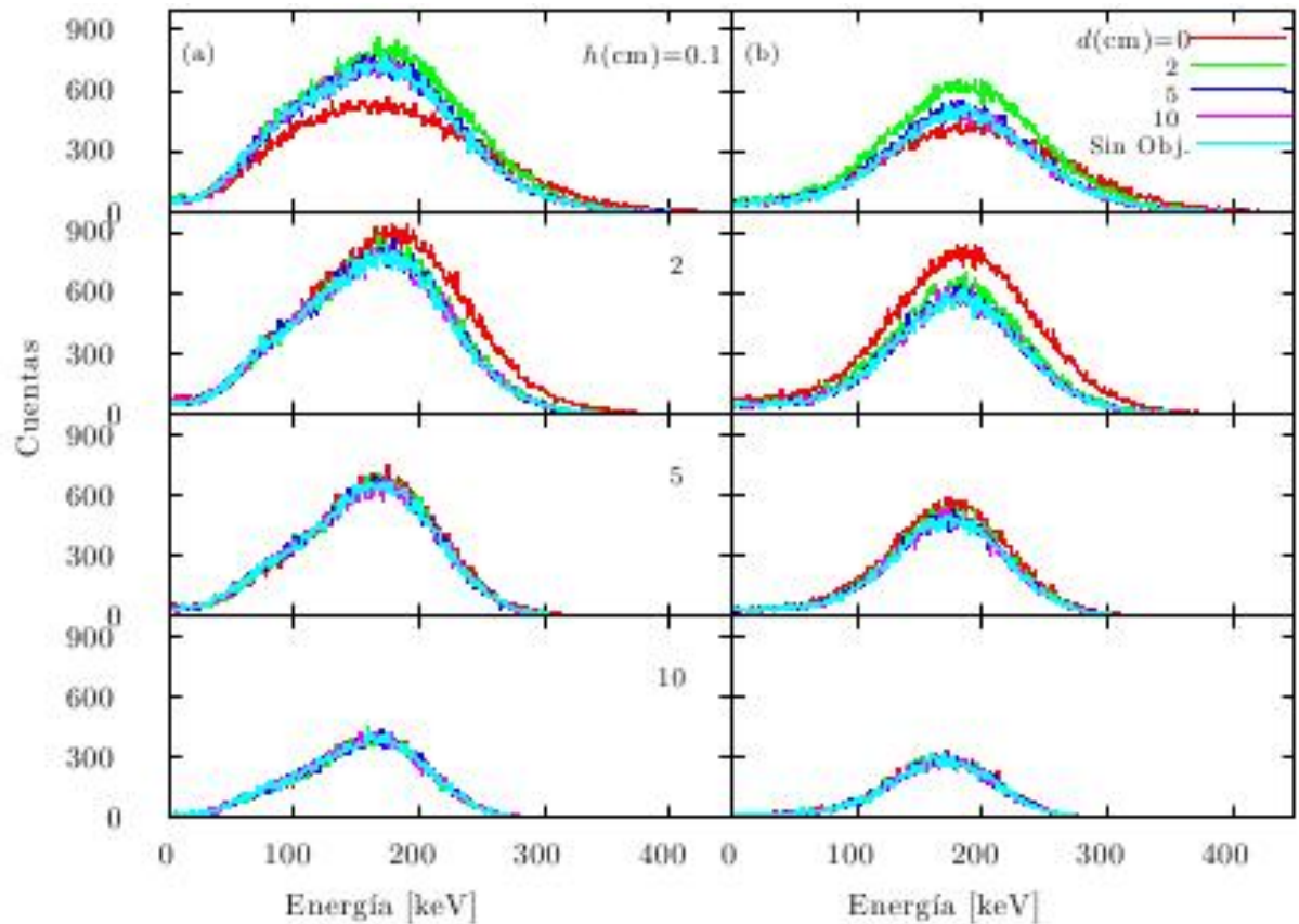
FIGURA 19: ESPECTRO DE RETRODISPERSIÓN PARA OBJETO DE HIERRO INMERSO EN: (A) ARENA Y (B) SUELO FRANCO CON LA RESPECTIVA VARIACIÓN DE LA POSICIÓN DEL DR (H) Y POSICIÓN DEL OBJETO (D).
