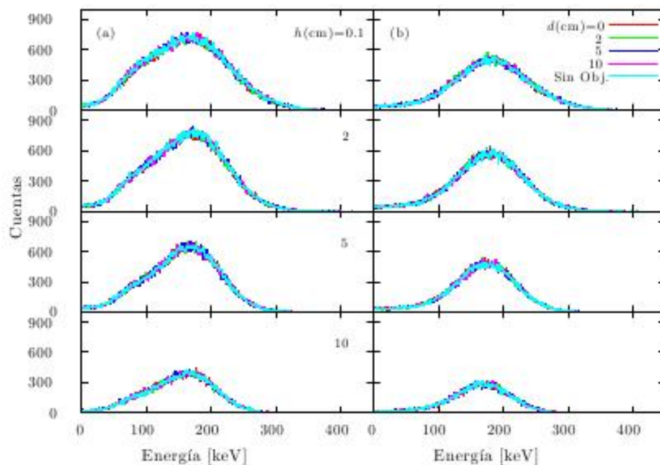
FIGURA 18: ESPECTRO DE RETRODISPERSIÓN PARA OBJETO DE POLIPROPILENO INMERSO EN A) ARENA Y B) SUELO FRANCO CON LA RESPECTIVA VARIACIÓN DE LA POSICIÓN DEL DR (H) Y POSICIÓN DEL OBJETO (D) VALIDAS PARA LAS DOS COLUMNAS.
