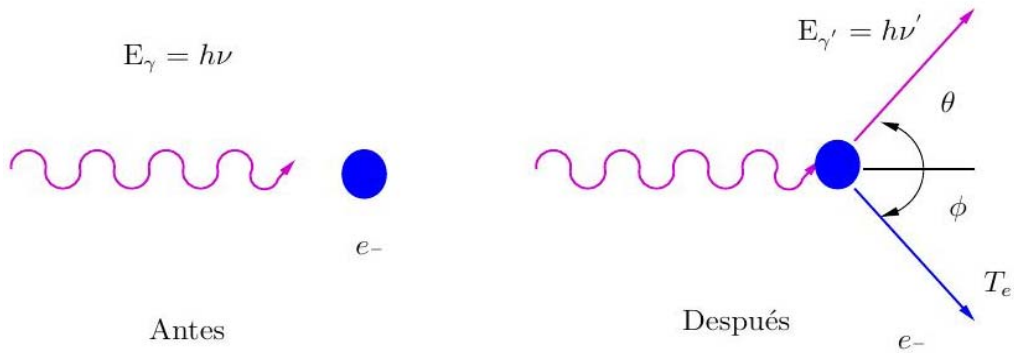
FIGURA 4: COLISIÓN ENTRE UN FOTÓN Y UN ELECTRÓN EN REPOSO.
