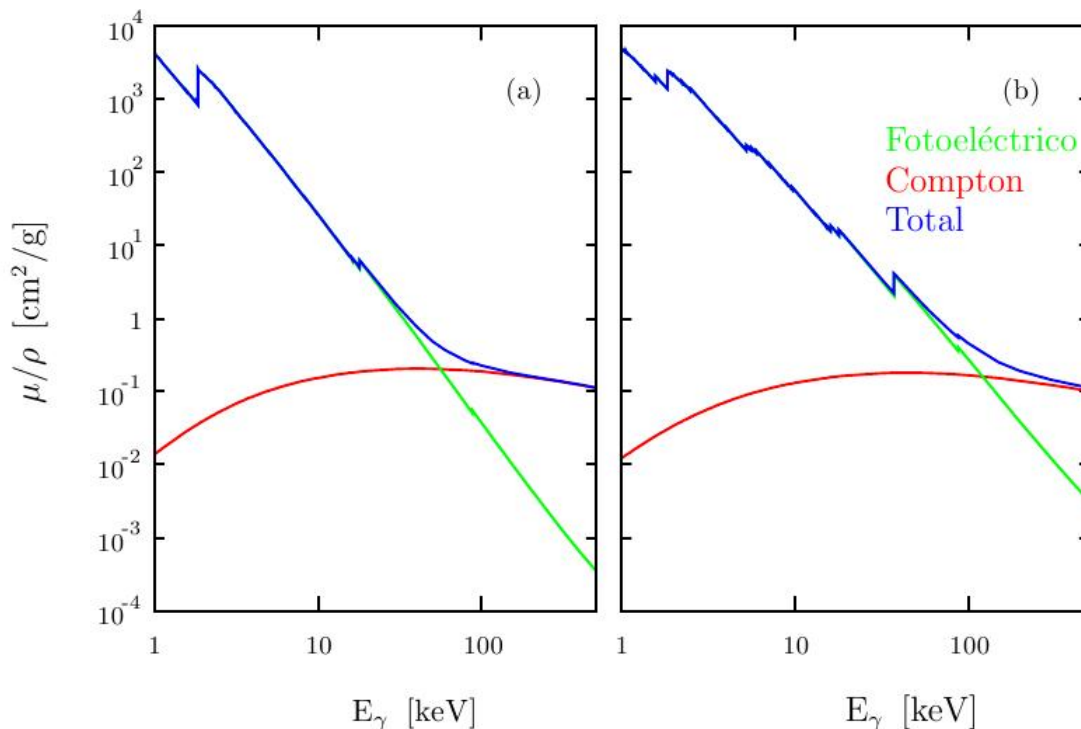
FIGURA 8 COEFICIENTE MÁSCICO DE ATENUACIÓN POR DISPERSIÓN COMPTON Y EFECTO FOTOELÉCTRICO en (a) arena y (b) suelo franco para rayos \gamma y entre [1-511] keV 6
