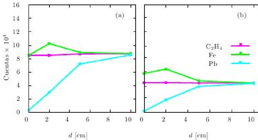
FIGURA 22 NUMERO DE RETRODISPERSIONES COMPTON MÚLTIPLES EN A) ARENA Y B) SUELO FRANCO PARA LOS TRES MATERIALES DEL OBJETO.
