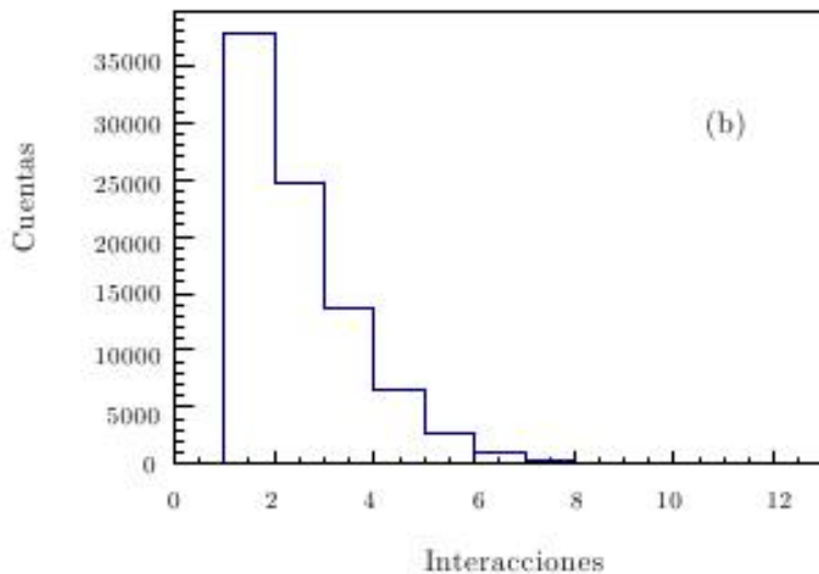
Figura 3.6: Numero de dispersiones que sufren los fotones antes de ser registrado en elDR.
