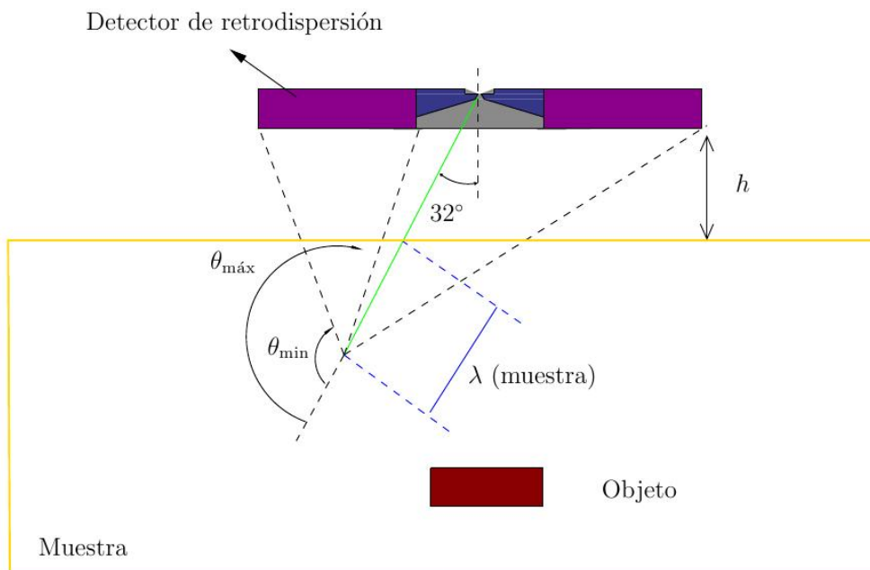
FIGURA 15: REPRESENTACIÓN DEL ÁNGULO MÍNIMO \theta_{\min} Y \theta_{\max} DE RETRODISPERSIÓN PARA LOS RAYOS \gamma QUE REALIZAN COMPTON
