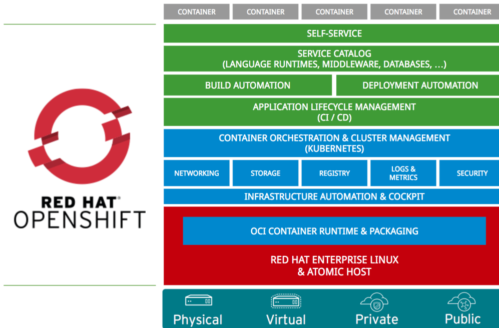
Figura 13. Arquitectura de Openshift. Adaptado de (Fernandes, 2017)
