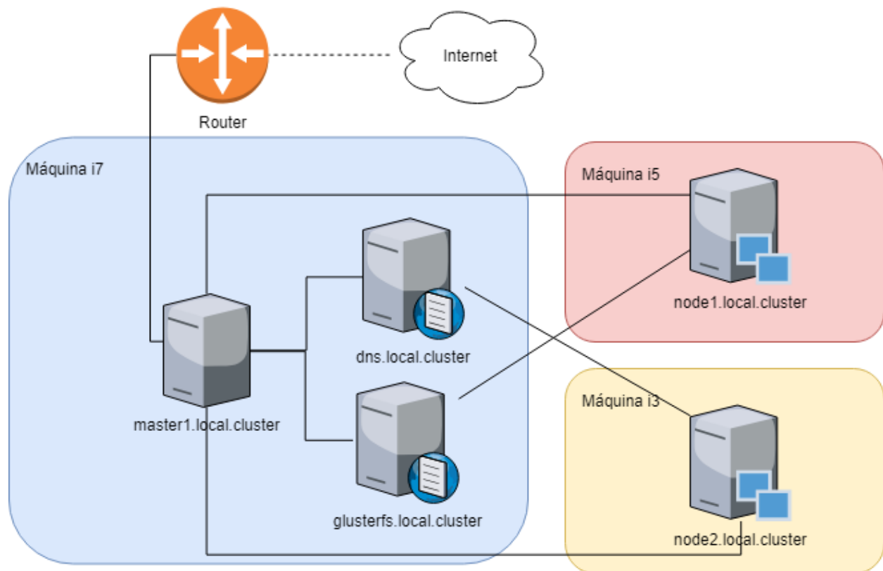
Figura 18. Infraestructura hardware del prototipo.
