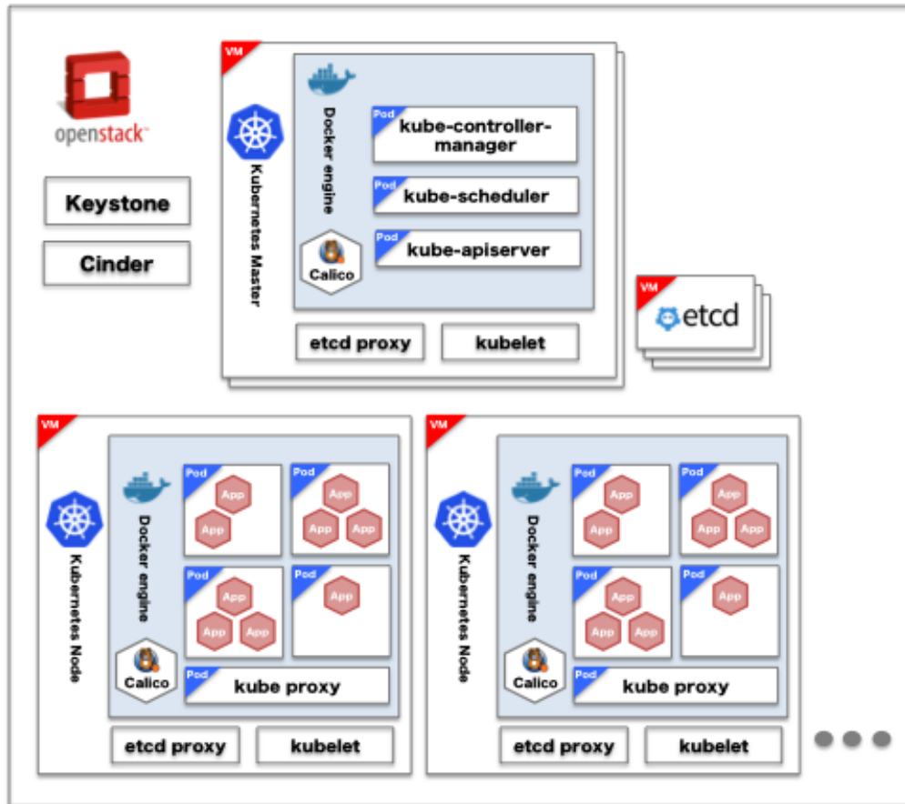
Figura 12. Arquitectura de un cluster Kubernetes. Adaptado de (Kubernetes, 2016a)
