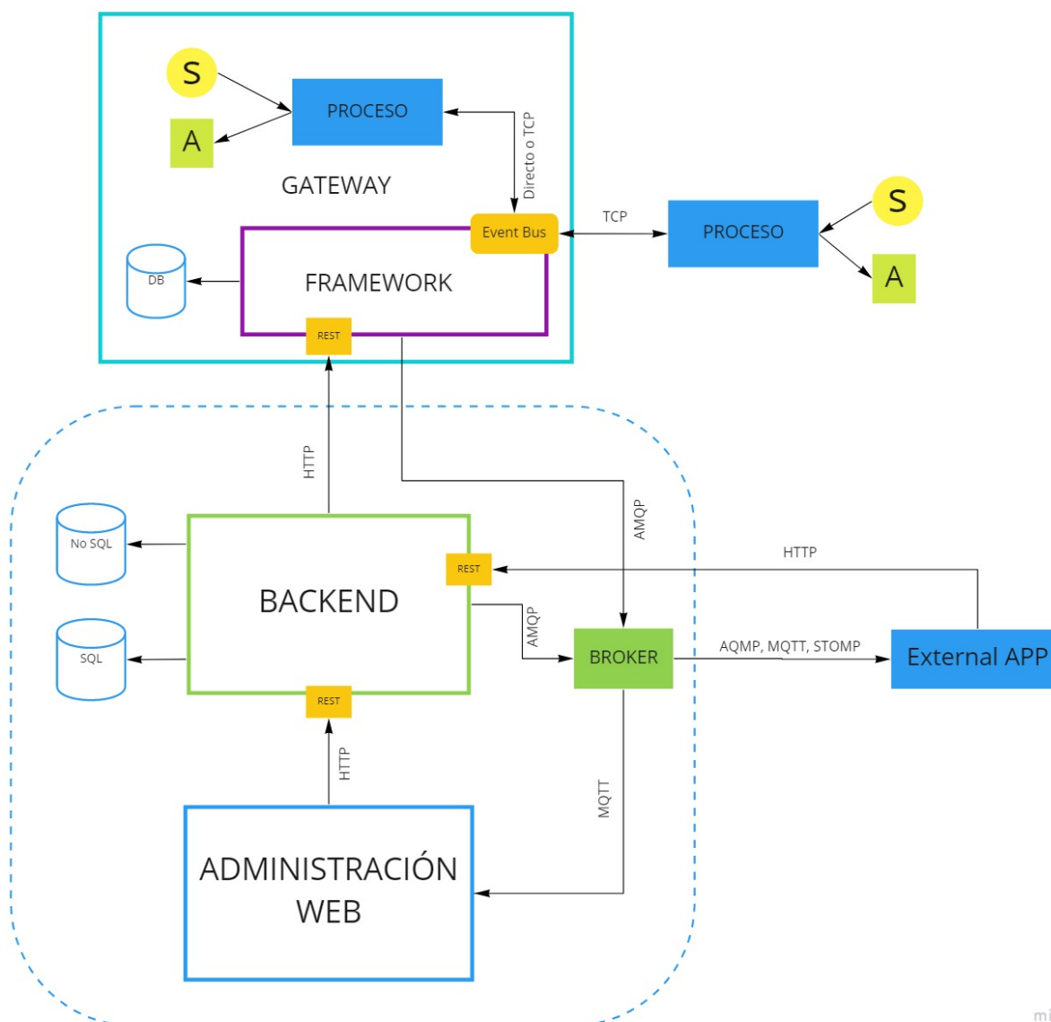
Figura 15. Arquitectura de la plataforma IoT.
