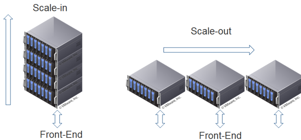
Figura 7. Escalabilidad vertical en contraste con escalabilidad horizontal. Adaptado de (Mauro, 2012)
