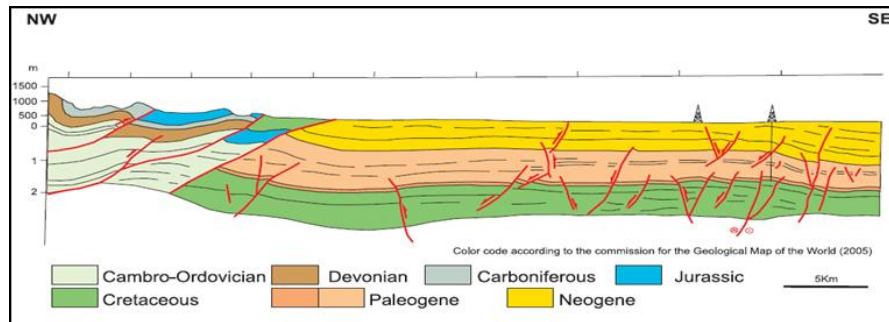
Ilustración 6. Esquema de la sección transversal, cuenca de los Llanos.
