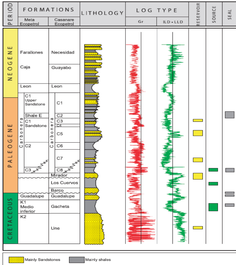
Ilustración 5. Columna litológica cuenca de los Llanos Orientales.
