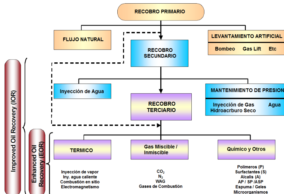
Ilustración 7. Etapas secuenciales de la recuperación de petróleo.
