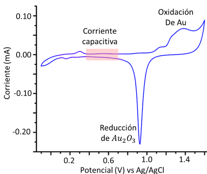
Figura 8. Voltamperograma cíclico de electrodo de oro en \text{H}_2\text{SO}_4 (0.5M). con una velocidad de barrido de 100mV/s y en una ventana de potencial de (-0.5 V a 1.6V).
