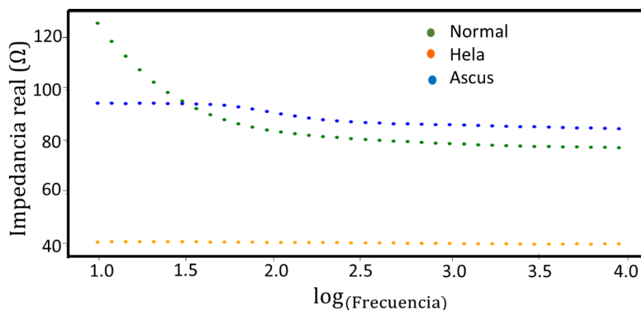
Figura 12. Formas de los Espectros de impedancia para las categorías Normal, ASCUS y el modelo de carcinoma cervical HeLa.
