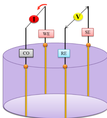
Figura 3. Configuración de cuatro electrodos tipo Van der Pauw. (CO: contraelectrodo; WE: electrodo de trabajo; SE: Sensor y RE: electrodo de referencia). La excitación de corriente se realiza en los electrodos CO y WE y la respuesta en voltaje se mide por SE y RE.
