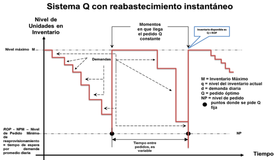
Grafico 4. Esquema de sistema de reabastecimiento instantáneo
