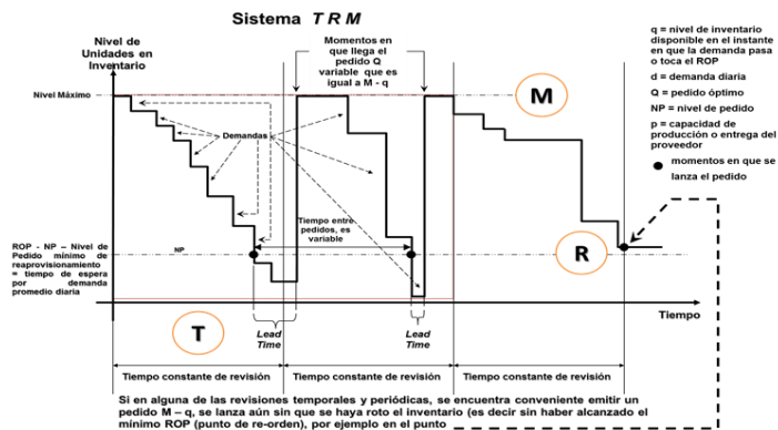
Grafico 8. Sistema TRM.
