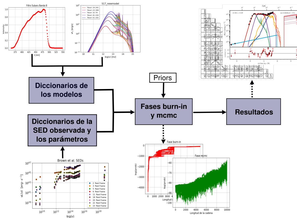
Figura 3.4 Esquema general del funcionamiento de AGNfitter.
