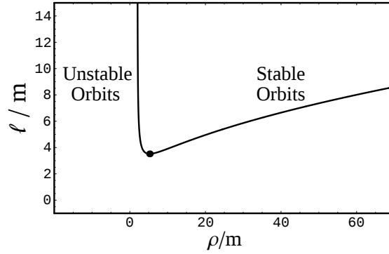
Figura 3.4: Relación entre el momentum angular específico, \ell/m , y el radio de una trayectoria circular, \rho/m , para geodésicas temporales en el caso de Chazy-Curzon. El punto tiene coordenadas (\ell/m, \rho/m) = (3,52, 5,23) . El rango de estabilidad está en 3,52m \leq \ell < \infty y 5,23m \leq \rho < \infty .
