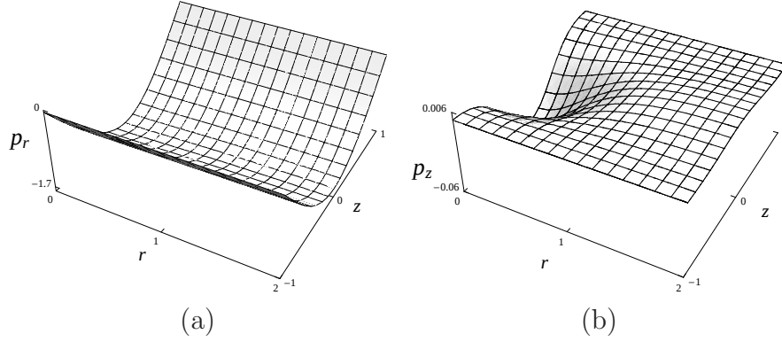
Figura 3.16: (a) Tensión Radial. (b) Presión Vertical, para el Disco Grueso tipo Bonnor-Sackfield, los parámetros escogidos son a = 1 , \gamma = 1 , y b = 2 .
