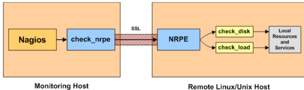
Figura 31: Modelo lógico nagios.
