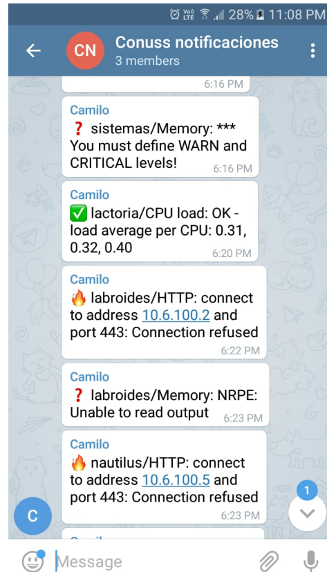
Figura 38: Notificaciones en la aplicación Telegram.
