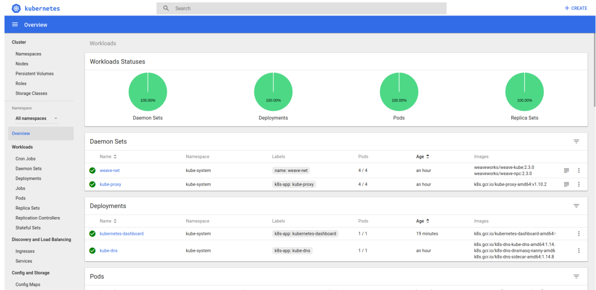
Figura 25: Pantalla inicial del dashboard de kubernetes.
