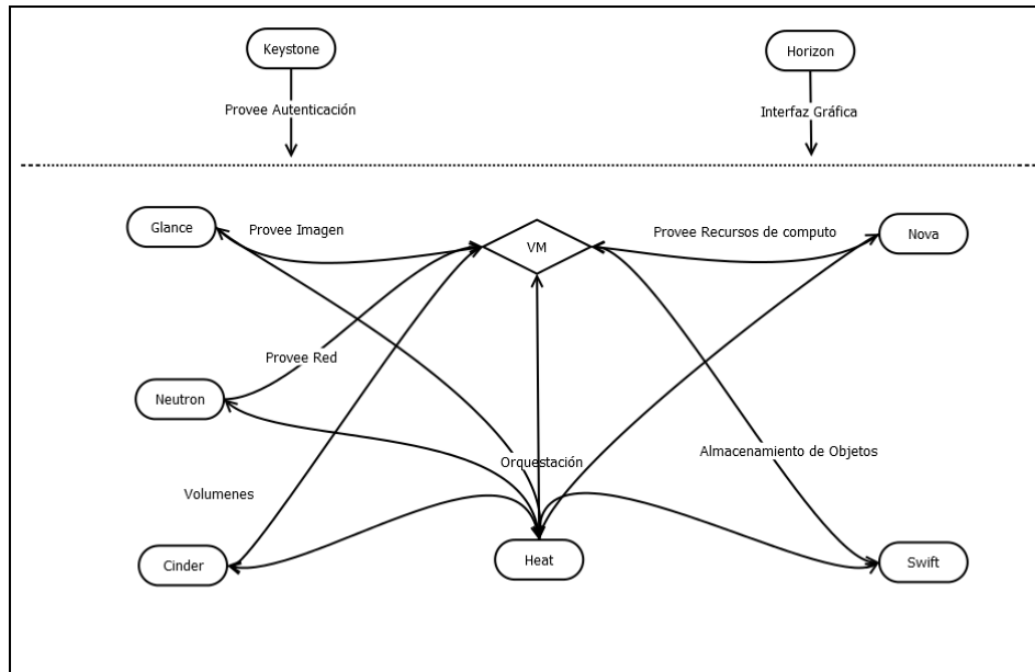
Figura 6: Modelo Conceptual.
