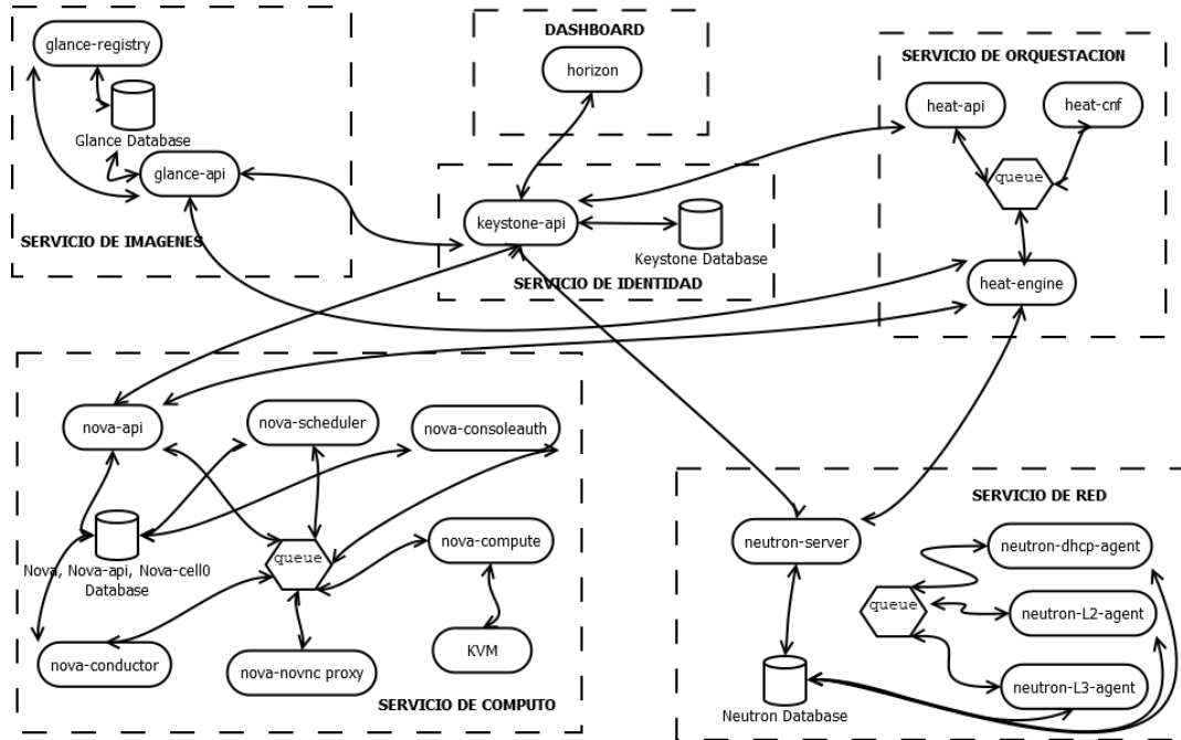
Figura 7: Modelo Lógico.
