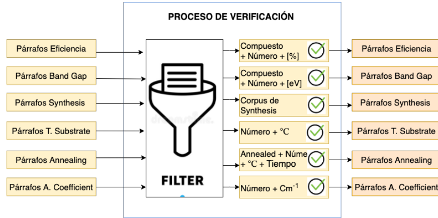
Figura 4: Diagrama de bloques del proceso de verificación.
