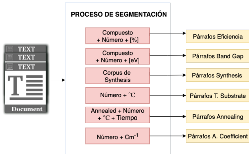
Figura 3: Diagrama de bloques del proceso de segmentación.
