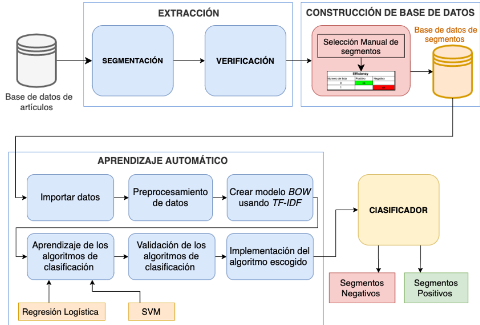
Figura 5: Diagrama de bloques del proceso de clasificación.
