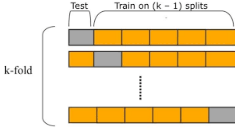
Figura 9: Proceso de funcionamiento de la validación k-fold.
