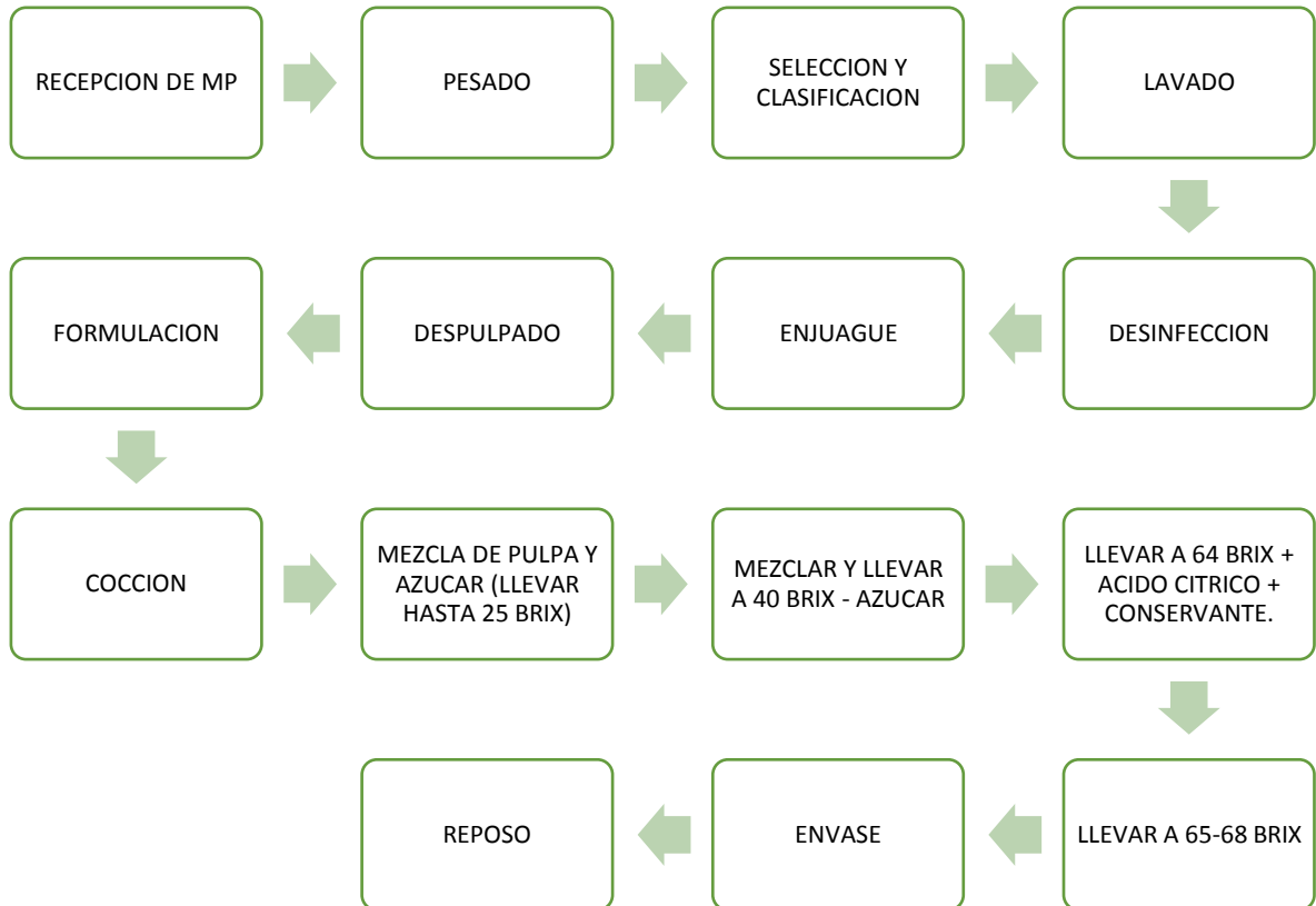
Figura 3. Diagrama proceso fabricación de mermelada
