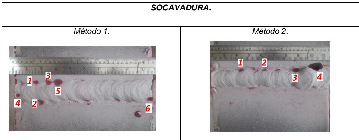
Figura 9. Fotografías del ensayo de líquidos penetrantes aplicado a las probetas con socavadura inducida generadas con el método uno y dos.
