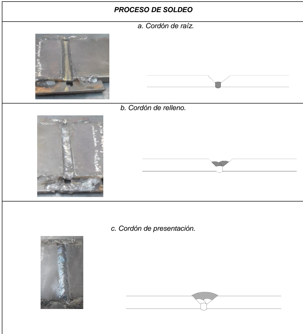
Figura 4. Proceso de soldeo.
