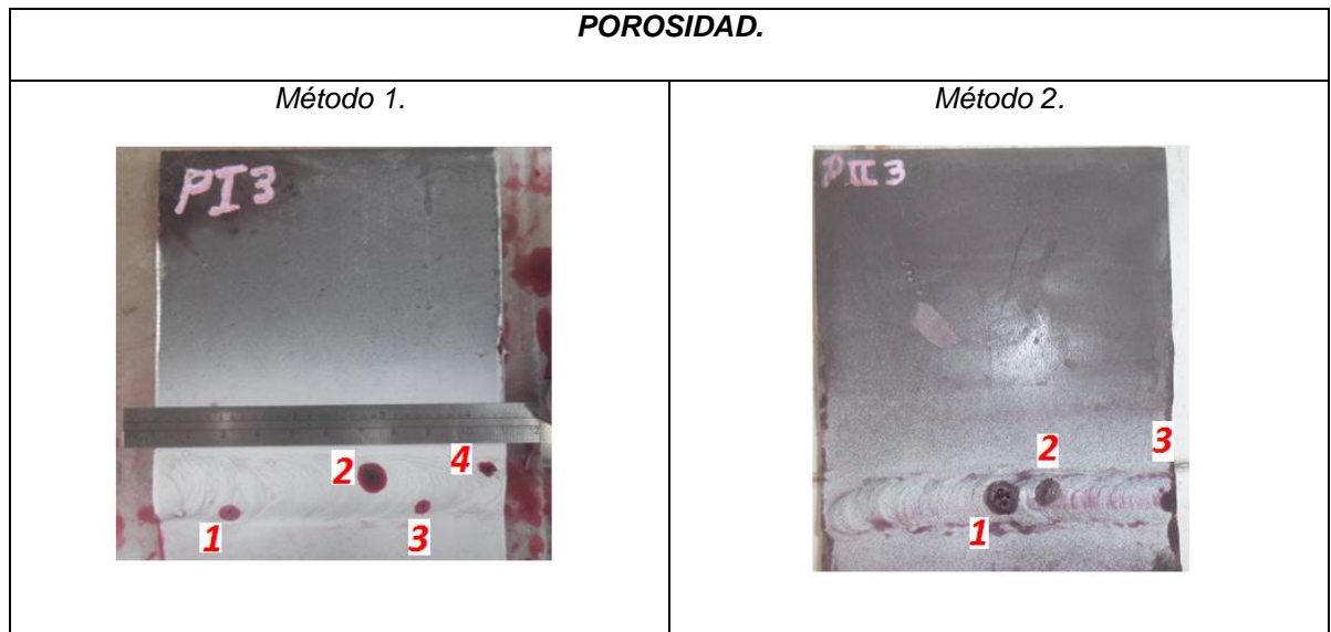
Figura 7. Fotografías del ensayo de líquidos penetrantes aplicado a las probetas con porosidad inducida generadas con el método uno y dos.
