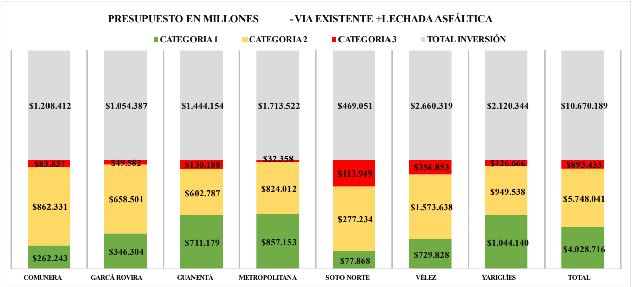
Figura 4. Presupuesto en millones para cada categoría por provincias para alternativa de mejoramiento: Vía existente + Lechada Asfáltica
