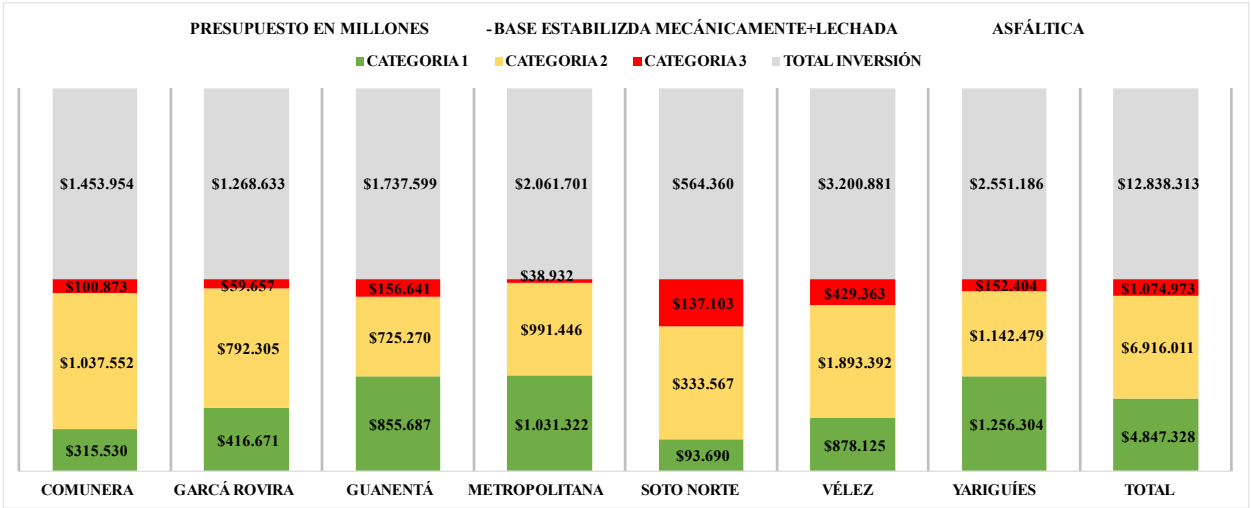
Figura 5. Presupuesto en millones para cada categoría por provincias para alternativa de mejoramiento: Base estabilizada mecánicamente + Lechada Asfáltica
