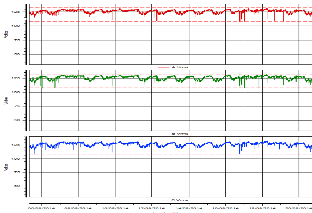
Figura 33. Perfiles de tensión por fase edificio FMB.
