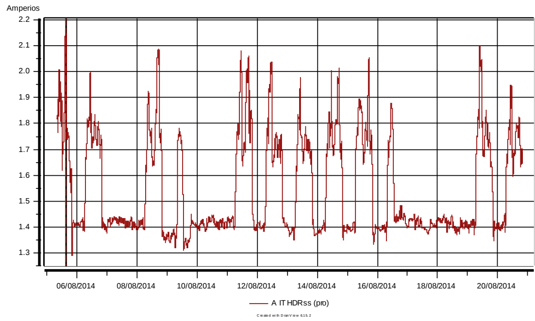
Figura 36. Armónico de corriente de la fase A
