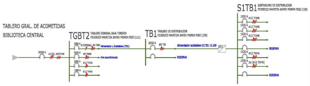
Figura 5. Diagrama Unifilar edificio Mamitza Bayer TG 2
