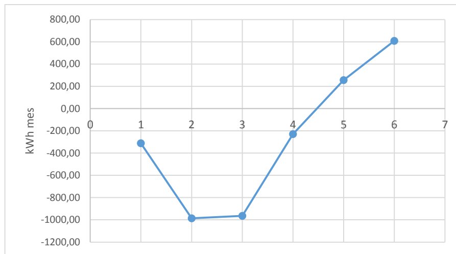
Figura 61 Diagrama de Sumas Acumuladas edificio DC
