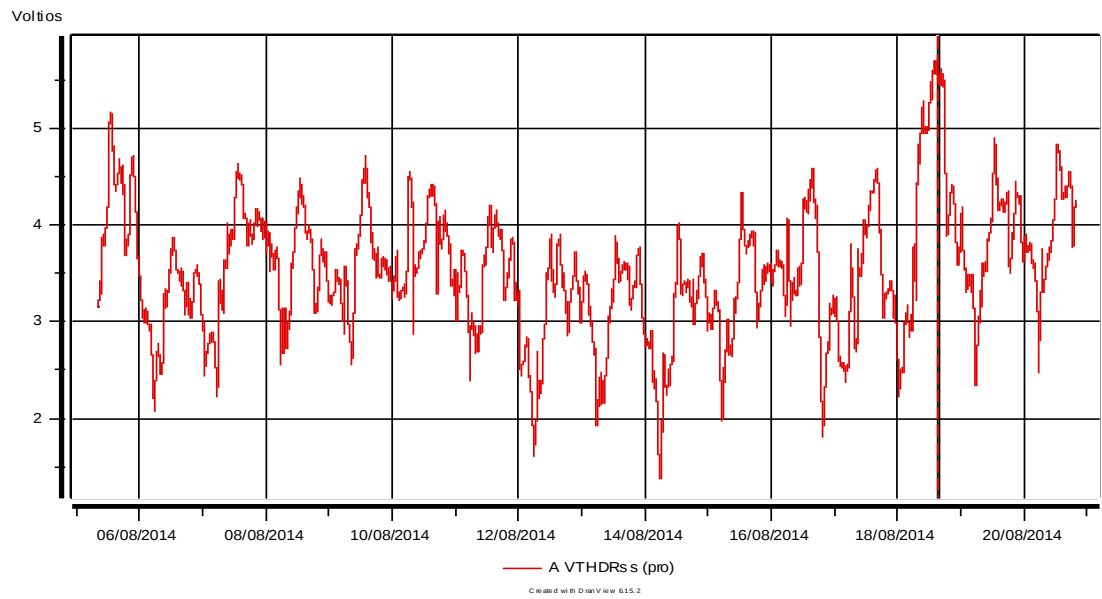
Figura 35. Armónico de tensión de la fase A
