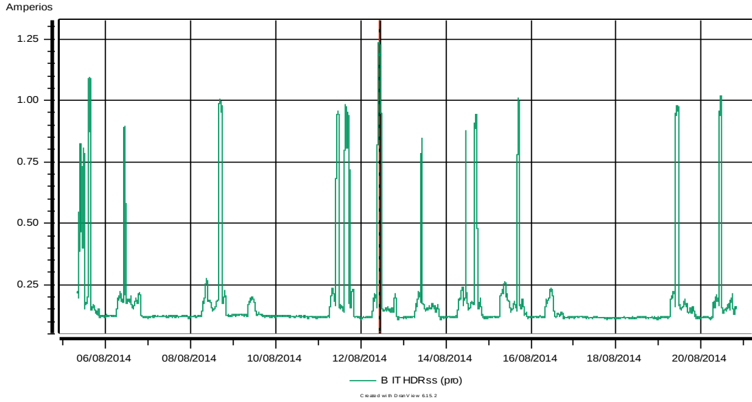
Figura 38. Armónico de corriente de la fase B
